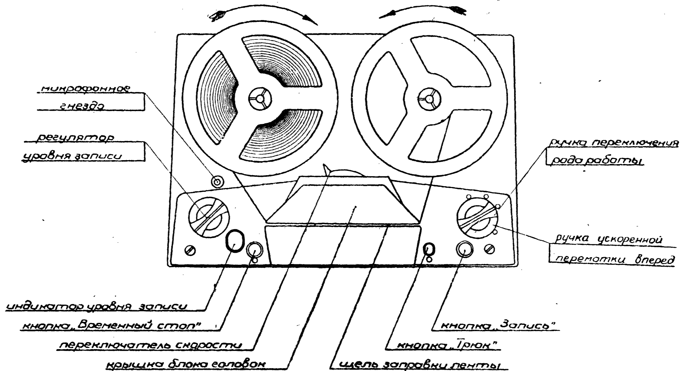
Рис. 4. Магнитофонная панель (вид, сверху)
