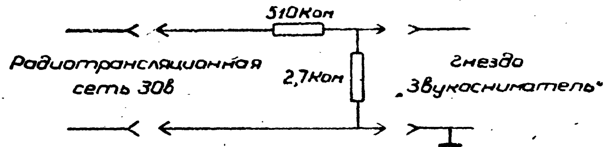
Рис. 5. Делитель напряжений для записи с радиотрансляционной линии
