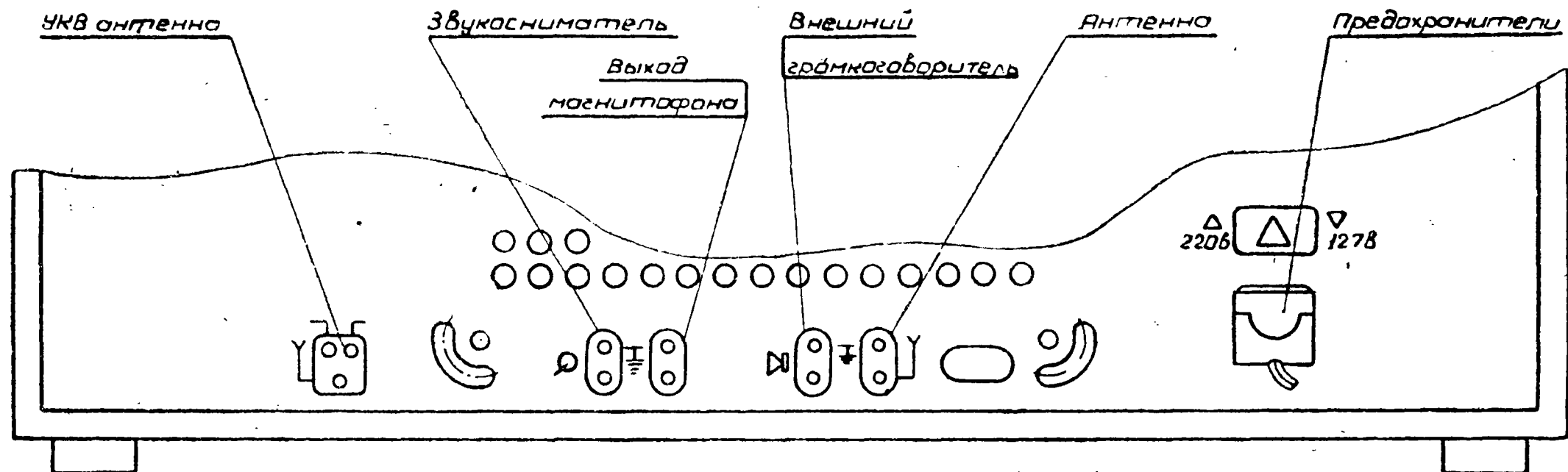
Рис. 3. Задняя стенка
