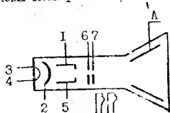
Схема расположения выводов
