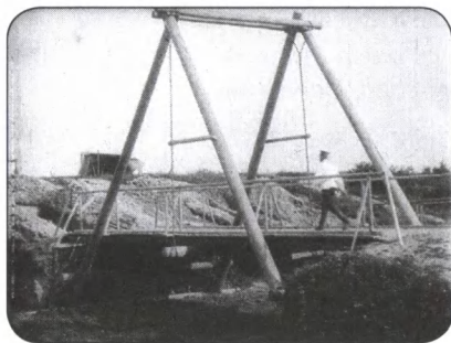
Вид стропильного подвесного моста. Фильм Скобелевского комитета «Л. Гв. Саперный батальон – наводка моста» РГАКФД. Уч. № 12388.
