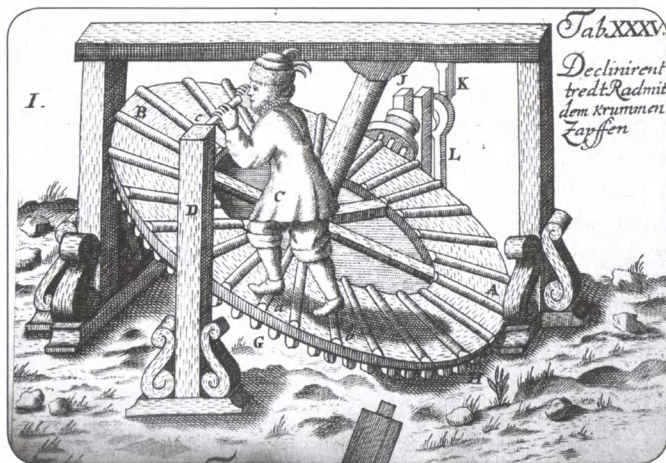
Иллюстрация из 7-томного труда «Theatri machinarum» Я. Леопольда, переданного В.Н. Татищевым в пользу заводов в 1734 г. По этим книгам обучался механике будущий создатель первой паровой машины в России Иван Ползунов
