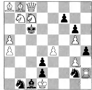
Обратный мат в 5 ходов
