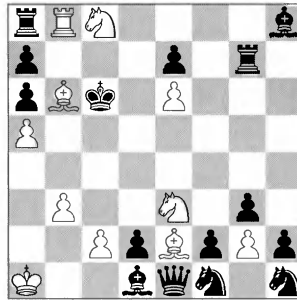
Коопмат в 2 хода 3 решения
