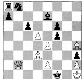
Обратный мат в 8 ходов
