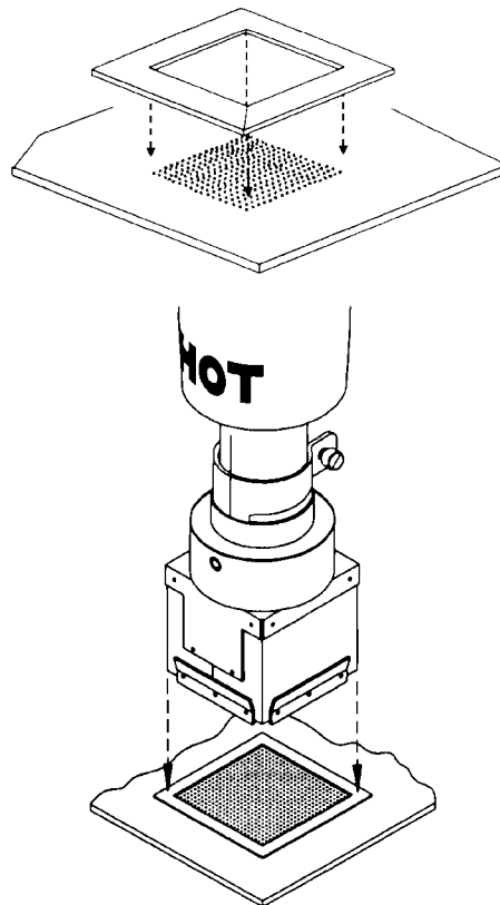
Рис. 3. Совмещение BGA-компонента с платой с помощью рамки
