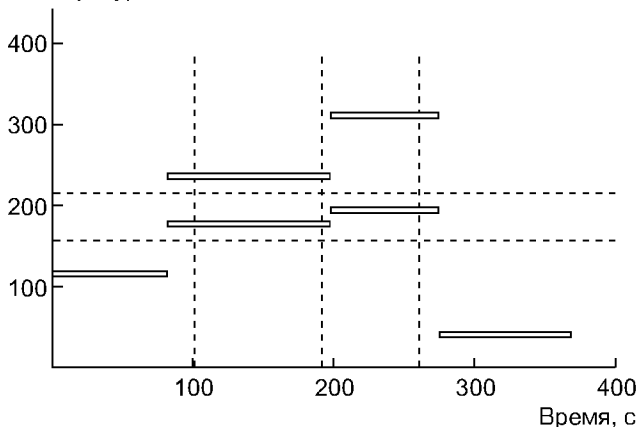
Рис. 2. Термопрофиль для BGA-492 (с сайта www.developer.intel.com/ ). Выше — температура воздуха в каждой зоне, ниже — температура компонента
