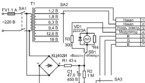
Рис. 1. Принципиальная схема прибора
