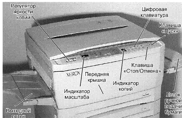
Рис. 1. Внешний вид аппарата
