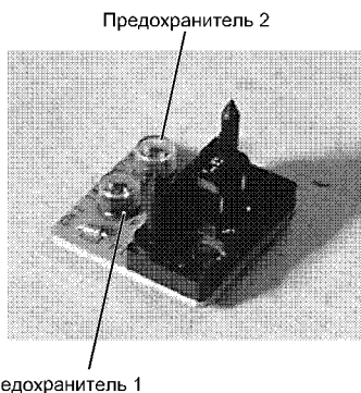
Рис. 2. Блок предохранителей
