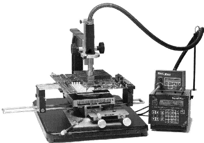
Рис. 1. Конвекционная паяльная система ThermoFlo
