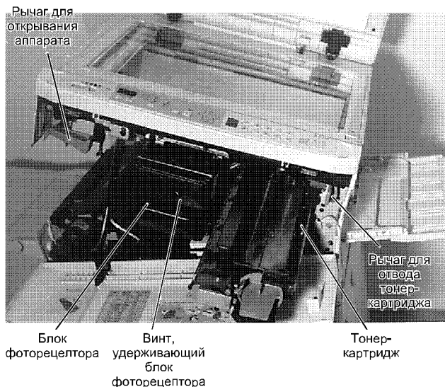
Рис. 3. Внешний вид открытого аппарата
