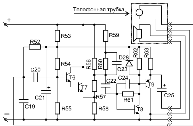
Т6, Т7, Т8 – КТ3102, 2N9014, Т9 – КТ502; D28 – КД521...; С19 – 10 нФ, С20, С22 – 100 нФ, С21 – 100 мкФ × 16 В, С23, С24 – 1 нФ, С25 – 20 мкФ; R52 – 5,6 кОм, R53 – 620 Ом, R54, R55 – 100 кОм, R56 – 110 кОм, R57 – 3,3 кОм, R58 – 18 Ом, R59 – 43 кОм, R60 – 270 кОм, R61 – 150 кОм, R62 – 3,3 кОм, R63 – 470 Ом
