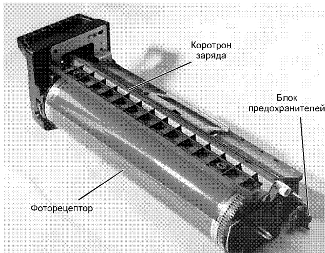
Рис. 4. Внешний вид блока фоторецептора
