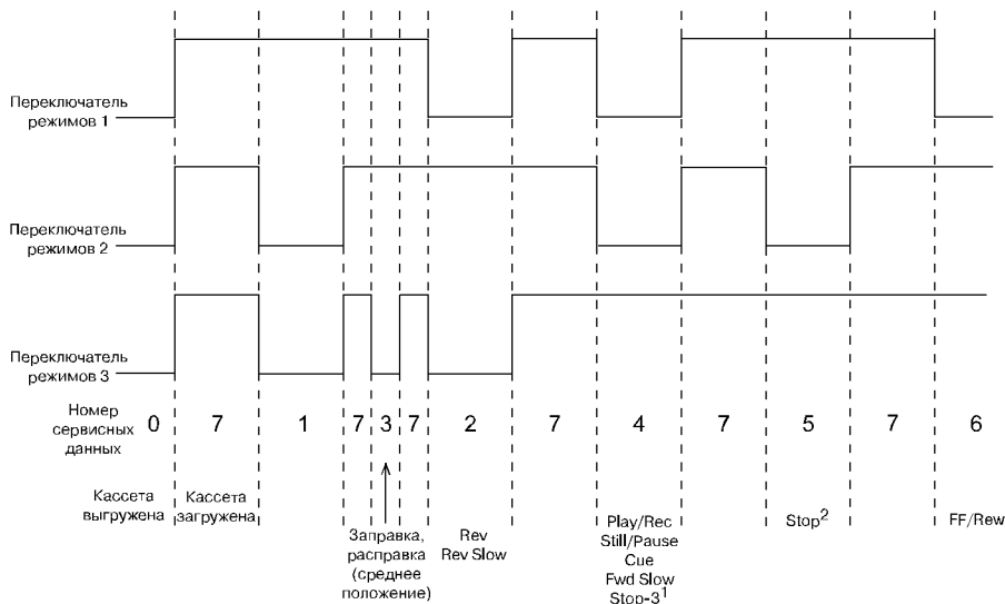
Рис. 1. Временная диаграмма переключателя режимов
