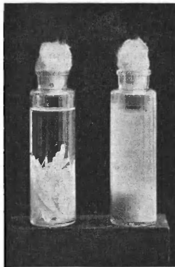
Рис. 1. Денитрификація при 37°. Слева культура только-что поставленная; жидкость совершенно прозрачна; на днѣ склянки бумага нарѣзанная полосками. Справа культура послѣ разрушенія трехъ послѣдовательно прибавленныхъ порцій \text{Ca}(\text{NO}_3)_2 ; жидкость сильно замутилась; на днѣ — разрушенные остатки бумаги. (Фотографія.)
