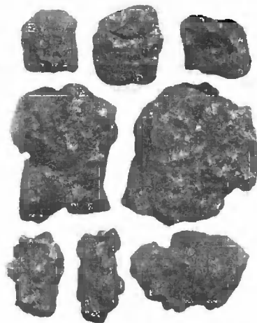
Рис. 5. Стяженія гидратовъ окиси желѣза.
