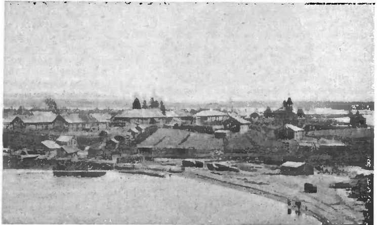
Рис. 3. С. Койкиницы, близъ котораго во многихъ мѣстахъ дно озера Выгъ покрыто рудой; на берегу въ пяти верстахъ имѣются дерновые руды.
