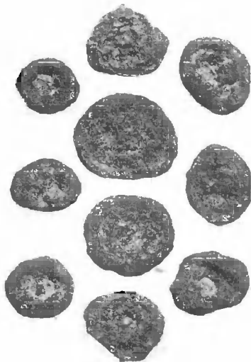
Рис. 6. Отложение гидратовъ окиси желѣза вокругъ галекъ и зеренъ кварца.
