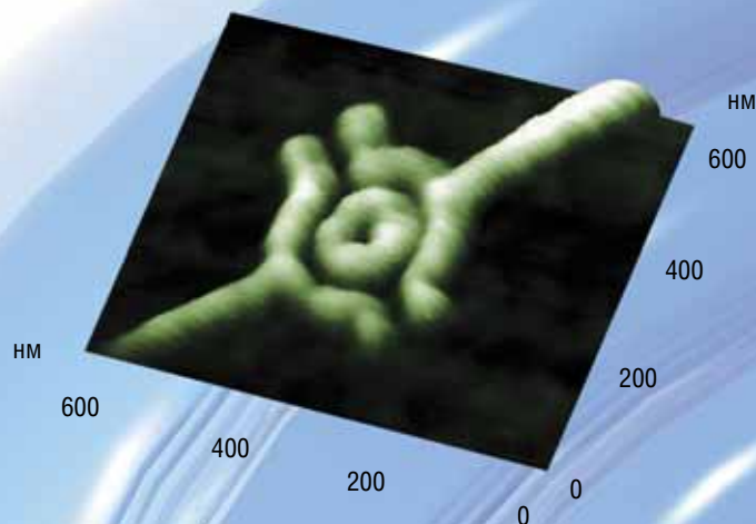
Электронный интерферометр, созданный с помощью запатентованной в ИФП СО РАН технологии локального анодного окисления на большую глубину посредством твердотельного зонда сканирующего зондового микроскопа. Атомно-силовой микроскоп. Фото из архива лаборатории нанодиагностики и нанолитографии ИФП СО РАН
