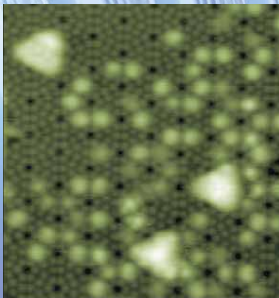
Изображение нанокластеров германия на реконструированной поверхности кремния с ориентацией (111) и шагом реконструкции (7×7). Сканирующий туннельный микроскоп (22 нм×22 нм). Фото к. ф.-м. н. С. А. Тийса
