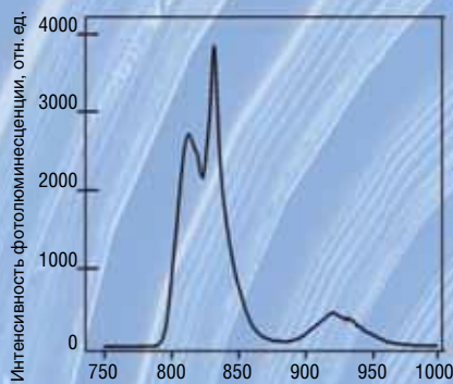
а) Фотолюминесценция массива квантовых точек при лазерном облучении (диаметр лазерного пятна 100 мкм)
