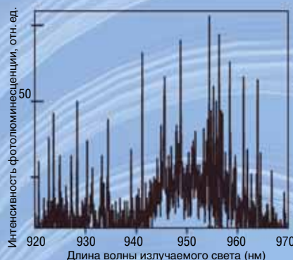
б) Микрофотолюминесценция квантовых точек (диаметр лазерного пятна 2 мкм)
