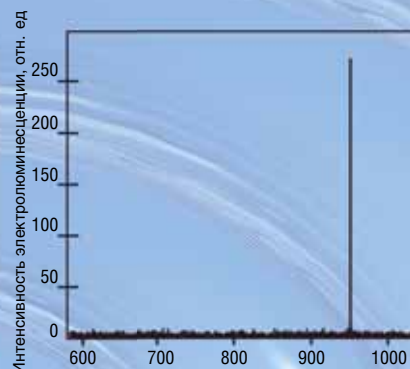
в) Нанoeлектролюминесценция при пропускании тока (диаметр токовой апертуры 0,85 мкм)
