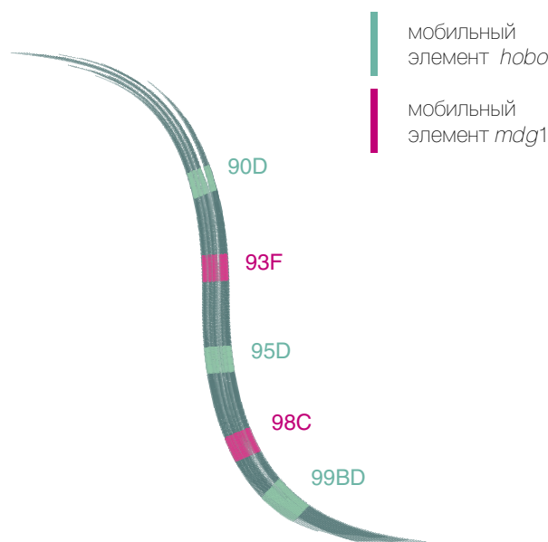
Положение мобильных элементов на фрагменте 3R хромосомы согласно базе данных 2000 г.
