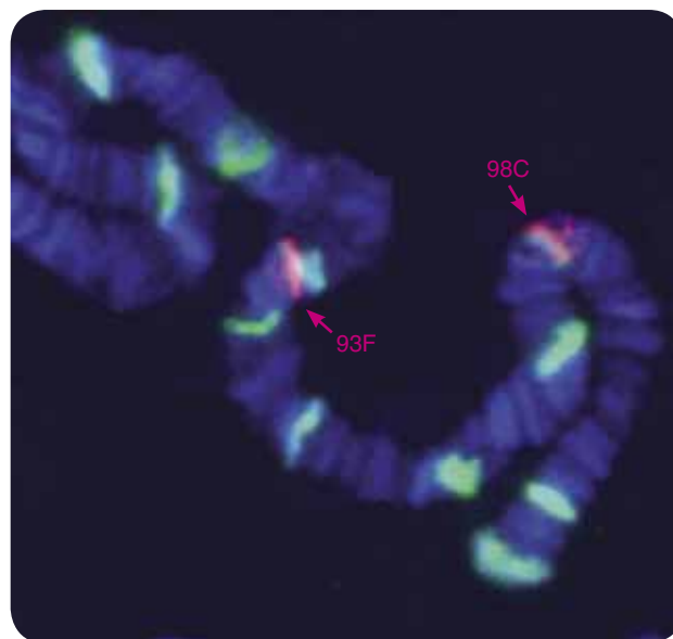
В 2005 г. анализ распределения мобильных элементов показал, что мобильный элемент mdg1 свои позиции в том же фрагменте хромосомы не поменял, а число hobo -элементов увеличилось в несколько раз, изменилось также их местоположение
