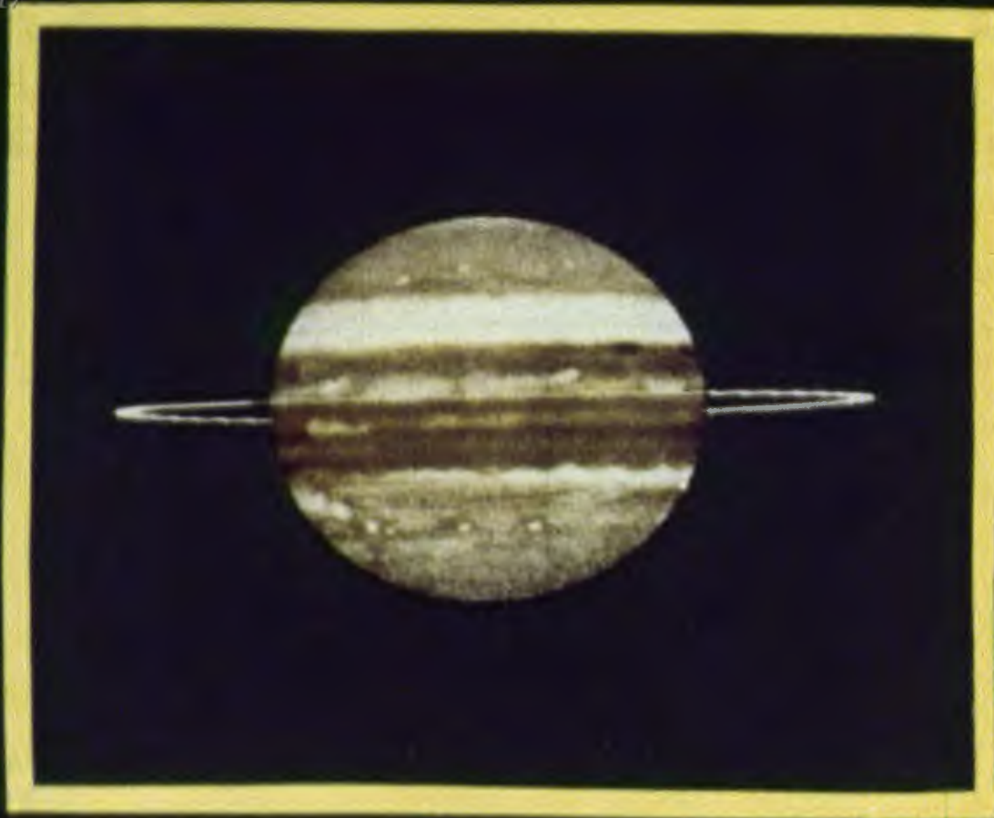
Юпитер с кольцом (рисунок).
