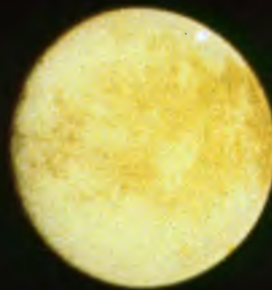
Европа
