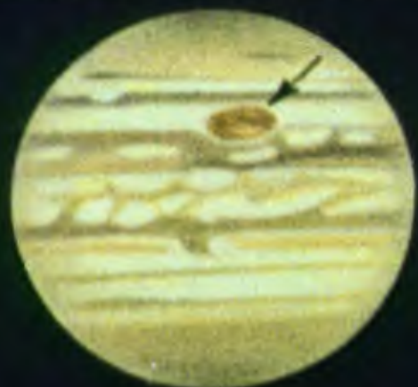
Красное Пятно— вид с Земли.
