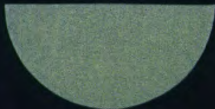
Земля Ø 12756 км
