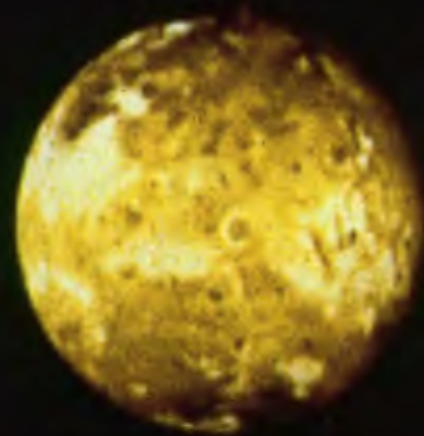
Ио
