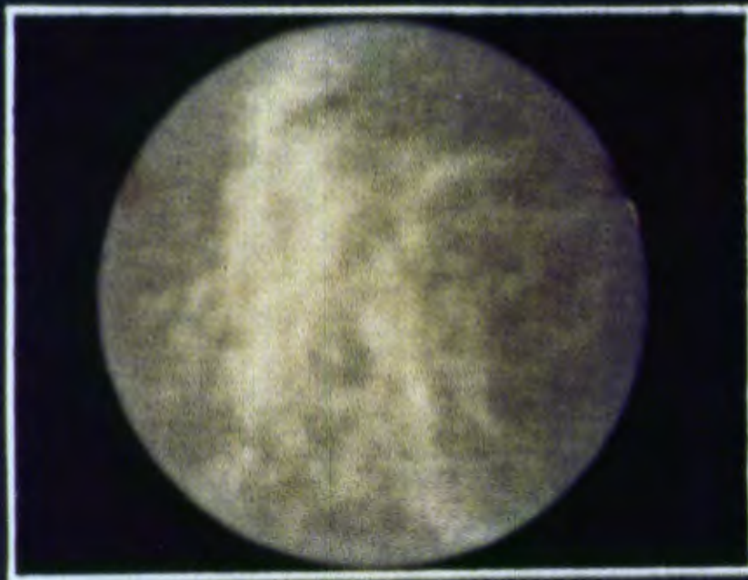
Рея.
