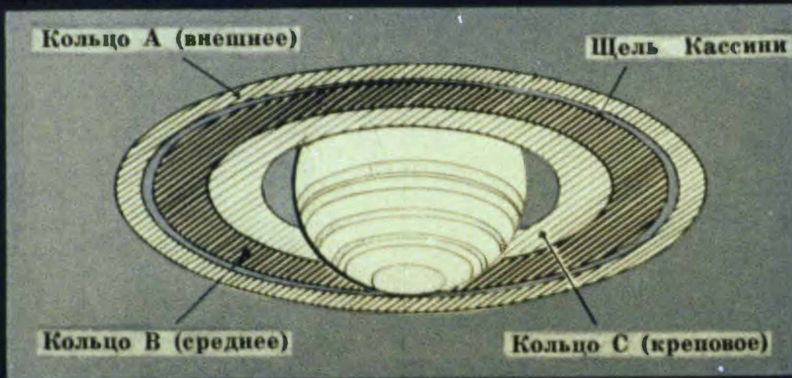
Схема видимых с Земли колец Сатурна.
