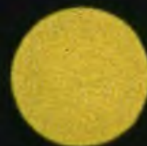
Ио 3640 км
