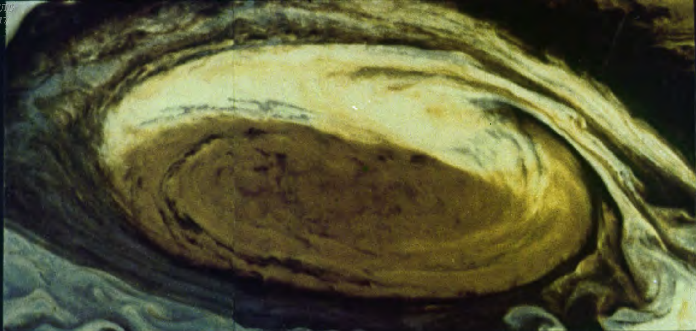
Красное Пятно— с расстояния 280 000 км.
