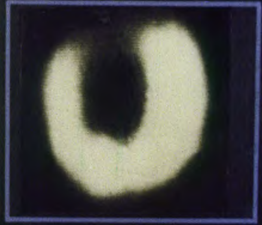
Первое фотографическое изображение колец Урана. 43
