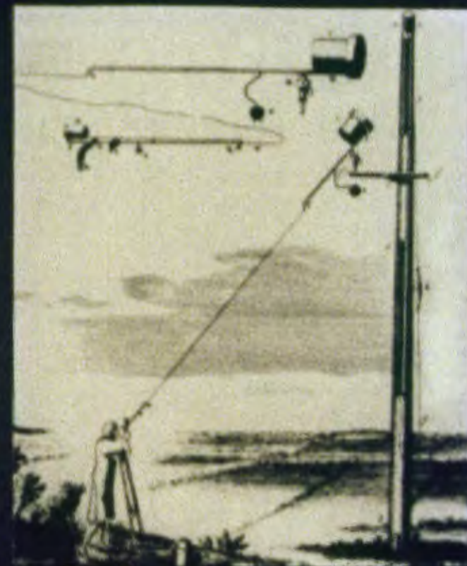
Гюйгенс во время наблюдения в свой телескоп.
