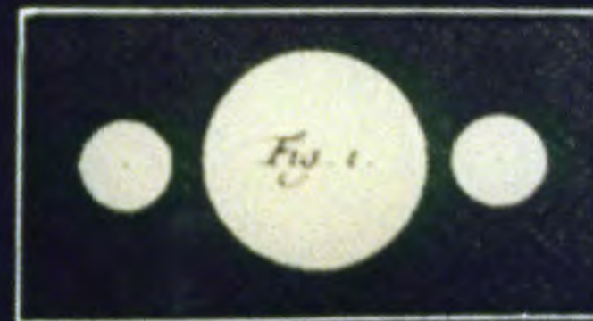
Рисунок Галилея.
