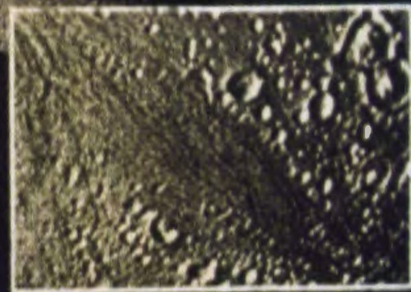
Энцелад.
