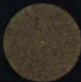
Каллисто 4820 км
