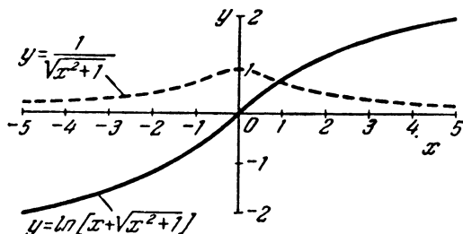
Рис. 200.01. Графики функций y = \frac{1}{\sqrt{x^2+1}} (пунктирная линия) и y = \ln |x + \sqrt{x^2+1}| (сплошная линия).
