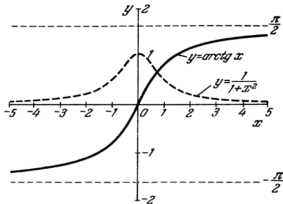
Рис. 120. Графики функций y = \frac{1}{1+x^2} (пунктирная линия) и y = \operatorname{arctg} x (сплошная линия).
