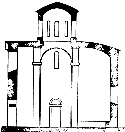
Рис. 4. Восточный фасадъ.
