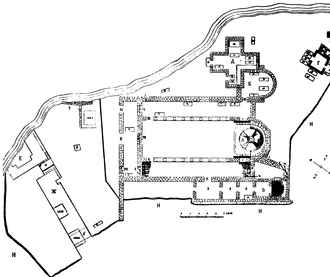
Рис. 1. Планъ раскопокъ въ сѣв.-западномъ углу Херсонесскаго городища въ 1901 году.
