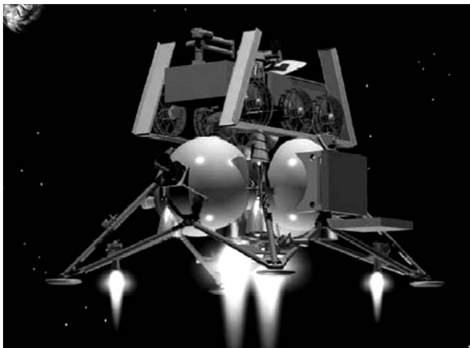
«Луна-Глоб»
