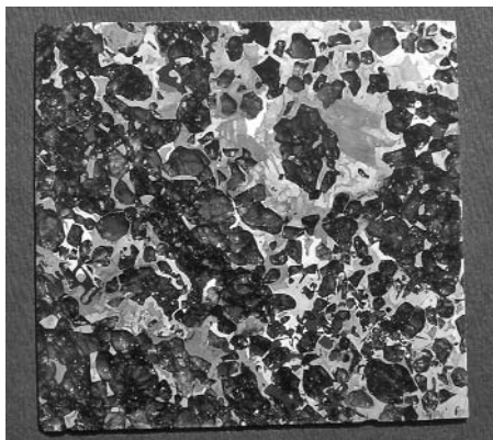
Кристаллы оливина
