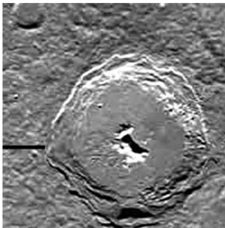
Кратер Пифагор
