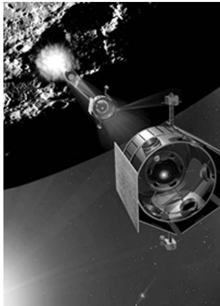
Зонд LCROSS
