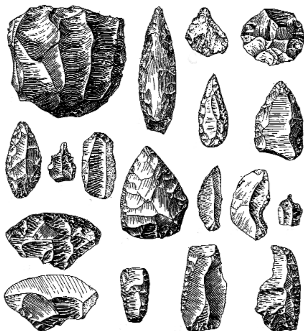
Ашельские скребки
