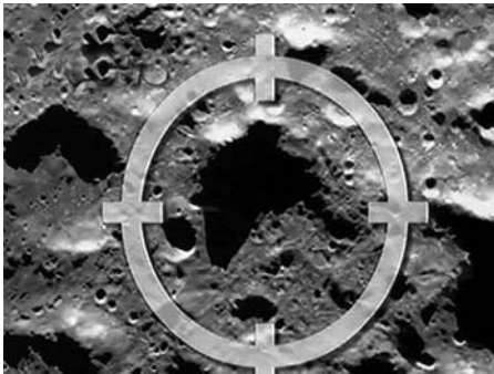
Кратер Кабеус
