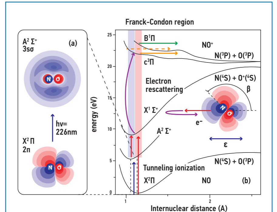
(a) Схематическое изображение состояний молекулы NO, (b) Переходы между различными состояниями молекулы NO (стрелки) и определение угла наклона молекулярной оси
