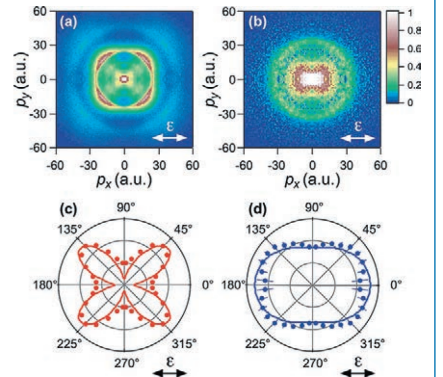
Распределение ионов N + по импульсу для начальной молекулы NO в основном (a и c) и возбужденном (b и d) электронных состояниях. Точками обозначены результаты эксперимента. Сплошными линиями обозначены результаты теоретических расчетов
