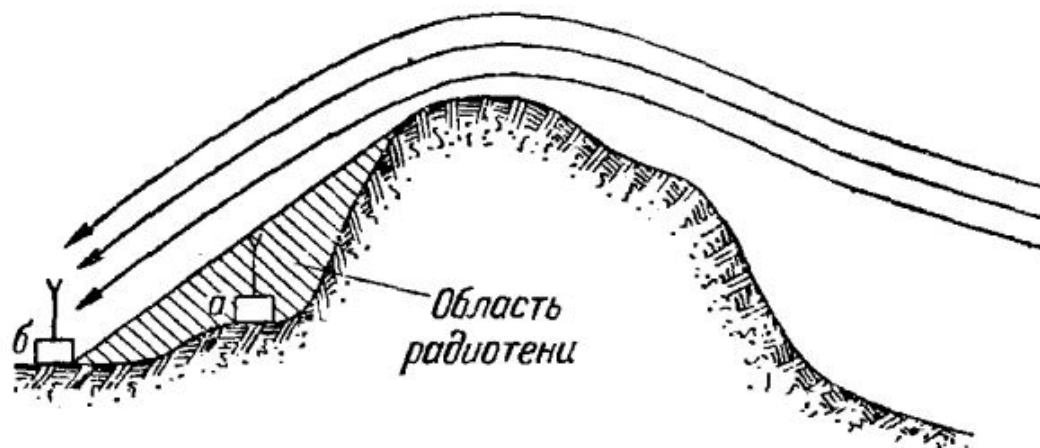
Рис. 1. Дифракция радиоволны
