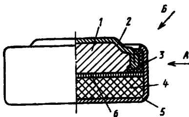
Рис. 4.11. Устройство дискового серебряно-цинкового элемента:
