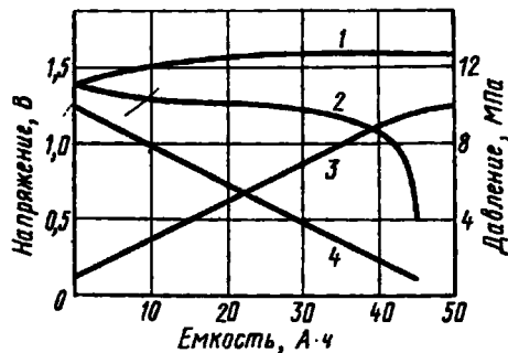
Рис. 11.3. Изменение напряжения (1, 2) и давления (3, 4) при заряде (1, 3) и разряде (2, 4) НВ аккумулятора емкостью 40 А·ч
