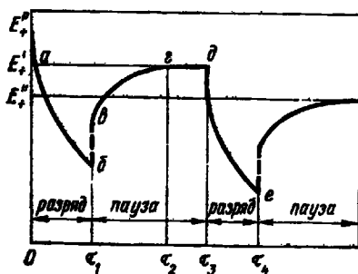
Рис. 4.1. Изменение потенциала положительного электрода МЦ элемента при разряде и в периоды токовой паузы
