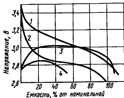
Рис. 5.1. Разрядные характеристики водоактивируемых батарей «Дымок» (1, 2) и «Маячок» (3, 4): активация соленой водой при 30°C (1, 3) и пресной при 1°C (2, 4)
