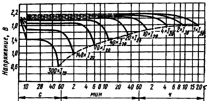
Рис. 7.12. Разрядные характеристики герметичного свинцового аккумулятора фирмы Sonnenschein при различных токовых нагрузках
