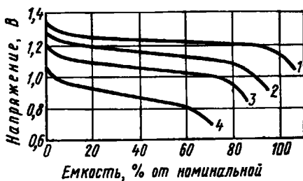
Рис. 9.2. Разрядные характеристики ламельного НК аккумулятора при температуре 20^{\circ}\text{C} и разряде током: 1 — 0,1 C_{\text{ном}} ; 2 — 0,5 C_{\text{ном}} ; 3 — 1 C_{\text{ном}} ; 4 — 2 C_{\text{ном}}
