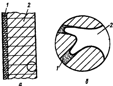
Рис. 6.1. Схема двухслойного гидрофильного газожидкостного электрода (а) и распределения электролита в газа и активном слое электрода (б): а — 1 — газозапорный слой; 2 — активный слой; б — 1 — жидкостная пора; 2 — газовая пора
