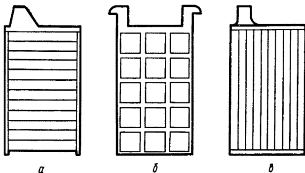
Рис. 2.2. Варианты каркаса электрода закрытого типа: а — ламельный; б — коробчатый; в — панцирный
