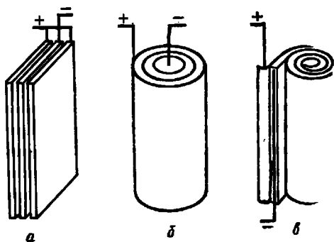
Рис. 2.4. Взаимное расположение электродов источника тока: а — плоскопараллельное. б — соосное; в — спиральное
