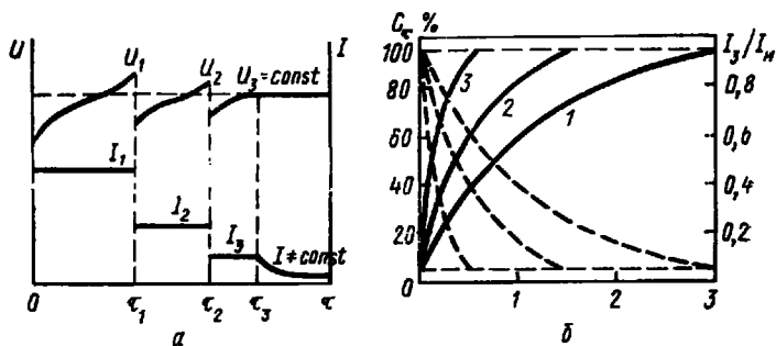
Рис. 3.6. Зарядные характеристики свинцового аккумулятора при комбинированных методах заряда:
