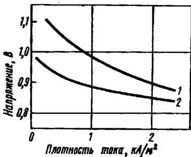
Рис. 6.4. Вольт-амперная характеристика среднетемпературного (1) и низкотемпературного (2) кислородно-водородного топливного элемента
