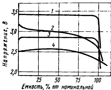
Рис. 4.16. Сравнительные разрядные характеристики литиевых элементов с апротонным электролитом:
