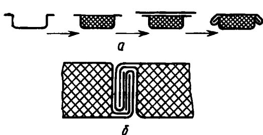
Рис. 8.2. Схема формования ламели (а) и соединение двух соседних ламелей «в замок» (б)
