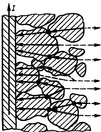
Рис. 1.3. Схема образования электрической цепи в пористом электроде:
