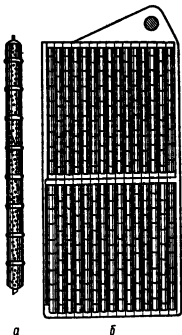
Рис. 8.4. Внешний вид ламели трубчатой конструкции (а) и трубчатой пластины (б)
