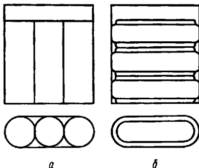
Рис. 4.5. Расположение элементов в батареях 3336 «Планета» (а) и «Рубин» (б)
