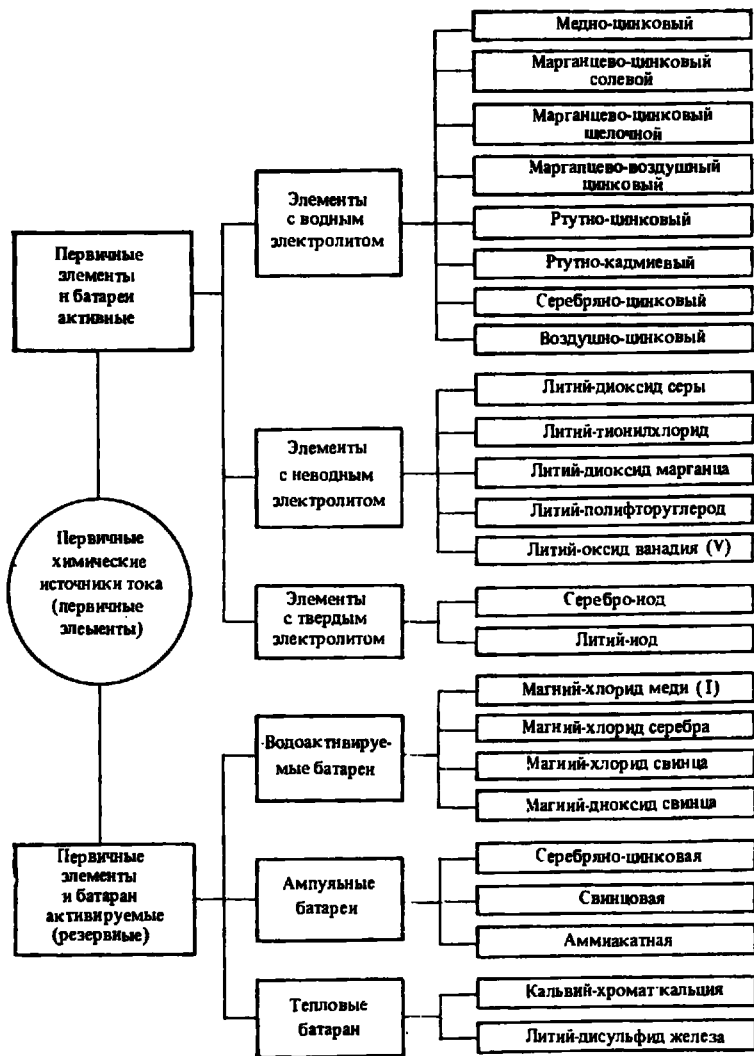
Схема 2.1. Классификация первичных ХИТ
