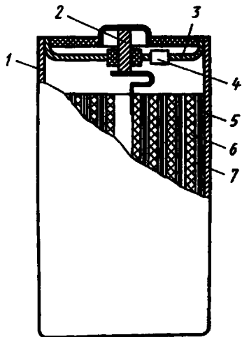
Рис. 4.14. Устройство цилиндрического элемента системы «литий — диоксид серы»: 1 — корпус; 2 — гермовывод; 3 — крышка; 4 — клапан; 5 — отрицательный электрод; 6 — положительный электрод; 7 — сепаратор
