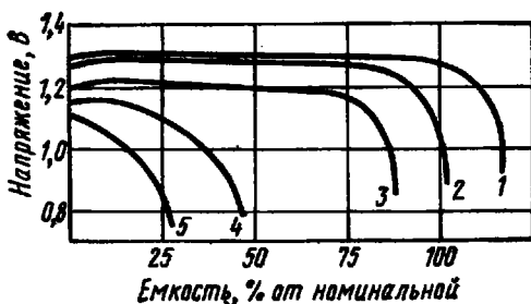
Рис. 4.9. Разрядные характеристики дискового элемента РЦ73 при температуре 50°C (1), 20°C (2) и 0°C (3—5):
