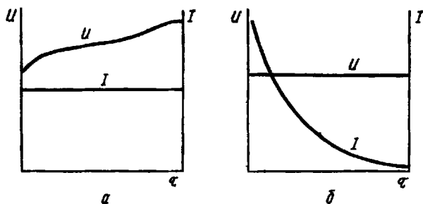
Рис. 3.5. Зарядные характеристики свинцового аккумулятора при заряде стабилизированным током (а) и при стабилизированном напряжении (б)
