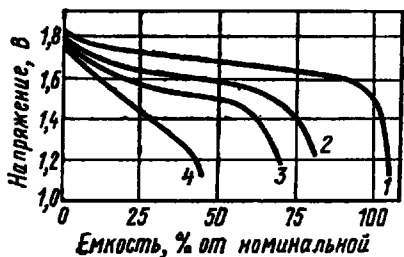
Рис. 11.2. Влияние температуры на разрядные характеристики НЦ аккумулятора при токе 0,5 C ном и температуре: 1 — 20 °С; 2 — 5 °С; 3 — минус 10 °С; 4 — минус 20 °С
