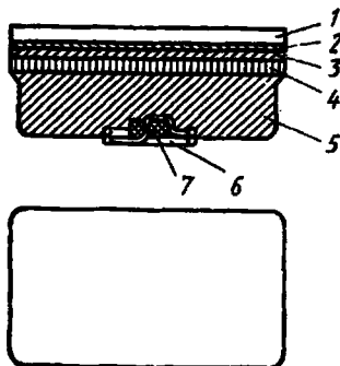
Рис. 4.13. Устройство воздушно-марганцево-цинкового элемента батареи «Крона ВЦ»:
