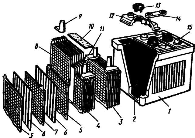
Рис. 7.1. Устройство стартерной аккумуляторной батареи:
