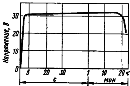
Рис. 5.3. Разрядная характеристика ампульной серебряно-цинковой батареи фирмы Eagle — Picher
