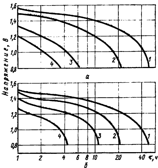
Рис. 4.7. Разрядные характеристики МЦ элементов при разных токах разряда, 20 °С:
