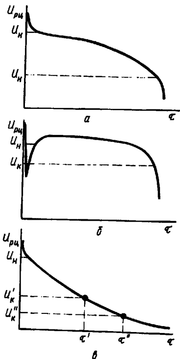
Рис. 3.1. Варианты разрядных характеристик химических источников тока
