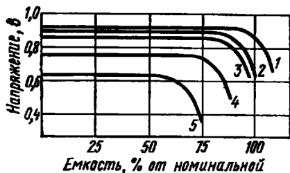
Рис. 4.10. Разрядные характеристики дискового ртутно-кадмиевого элемента:
