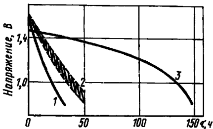
Рис. 4.6. Сравнительные разрядные характеристики солевого и щелочного МЦ элемента при токе разряда 40 мА, 20 °С:
