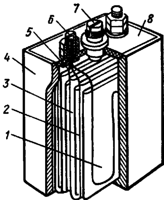
Рис. 10.2. Устройство серебряно-цинкового аккумулятора:
