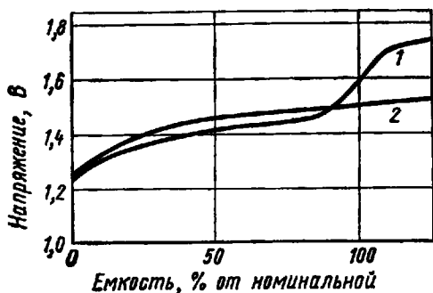
Рис. 9.1. Изменение напряжения при заряде негерметичного (1) и герметичного (2) НК аккумулятора
