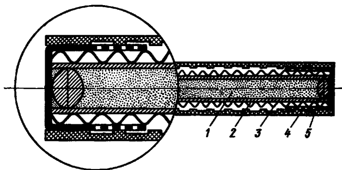
Рис. 7.4. Конвертовка положительных электродов аккумуляторов типа СН:
