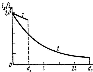
Рис. 1.4. Распределение плотности тока по толщине в тонком (1) и толстом (2) пористом электроде
