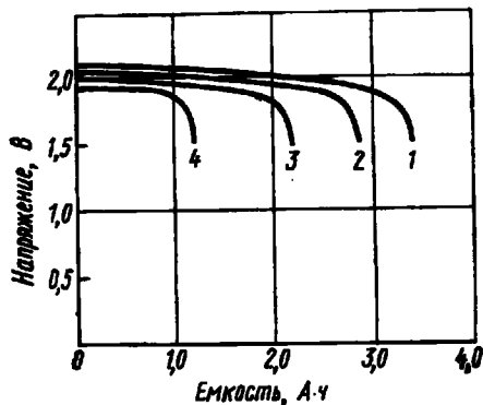
Рис. 7.13. Разрядные характеристики цилиндрического герметизированного свинцового аккумулятора фирмы General Electric:
