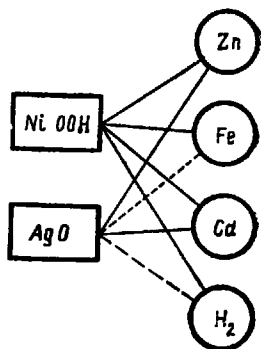
Рис. 2.3. Обратимые электрохимические системы на основе щелочного электролита:
