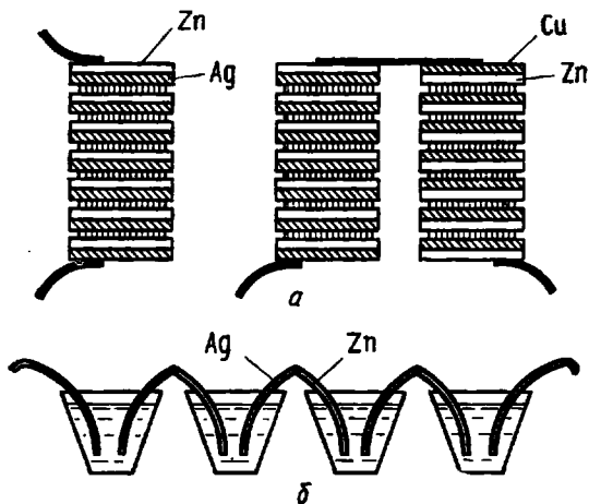
Рис. В.1. Химические источники тока А. Вольта:
