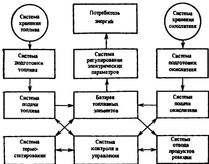
Схема 6.1. Функциональная схема электрохимического генератора
