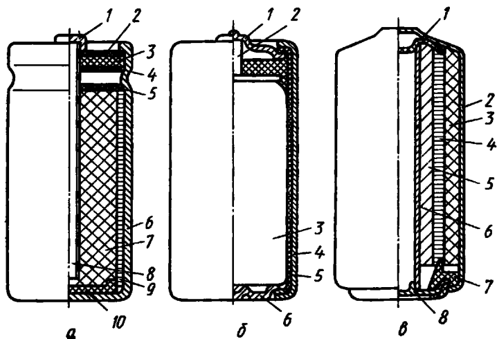
Рис. 4.2. Устройство цилиндрических МЦ элементов:
