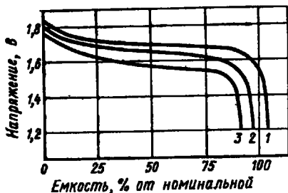
Рис. 11.1. Разрядные характеристики НЦ аккумулятора при температуре 20 °С и разряде током: 1 — 0,06 C ном ; 2 — 0,5 C ном ; 3 — 1 C ном
