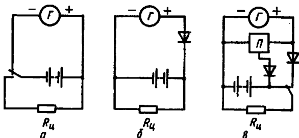
Рис. 3.7. Схемы включения аккумуляторной батареи в зарядно-разрядную цепь при различных режимах эксплуатации:
