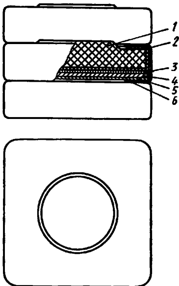
Рис. 4.3. Устройство галетного МЦ элемента:
