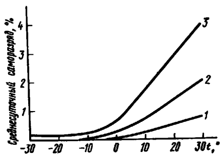
Рис. 7.11. Среднесуточный саморазряд стартерной батареи при хранении в течение 14 сут в зависимости от температуры:
