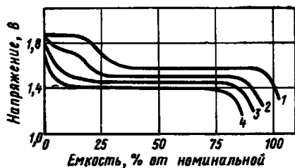
Рис. 10.3. Разрядные характеристики СЦ аккумулятора при температуре 20 °С и разряде тока:
