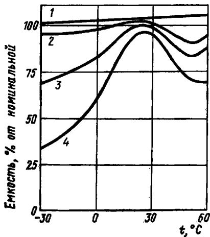
Рис. 4.15. Влияние температуры на емкость элемента 373 системы «литий — диоксид серы» при токах разряда:
