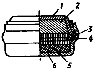
Рис. 4.8. Устройство дискового ртутно-цинкового элемента:
