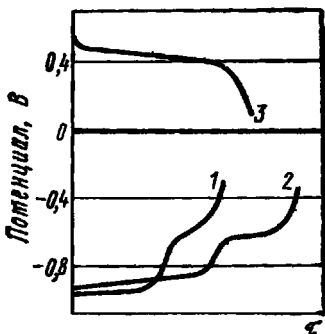
Рис. 8.1. Изменение потенциалов железного (1, 2) и оксидоникелевого (3) электродов НЖ аккумулятора при разряде:
