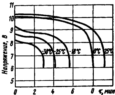
Рис. 7.9. Влияние температуры на разрядные характеристики батареи БСТ-182 при разряде током 500 А
