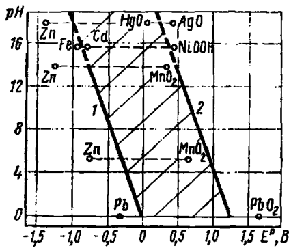
Рис. 3.4. Соотношение равновесных потенциалов электродов некоторых электрохимических систем и потенциалов водородного (1) и кислородного (2) электродов в зависимости от рН раствора: средняя зона — область термодинамической устойчивости воды
