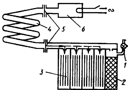
Рис. 5.2. Устройство ампульной серебряно-цинковой батареи фирмы Eagle — Picher:
