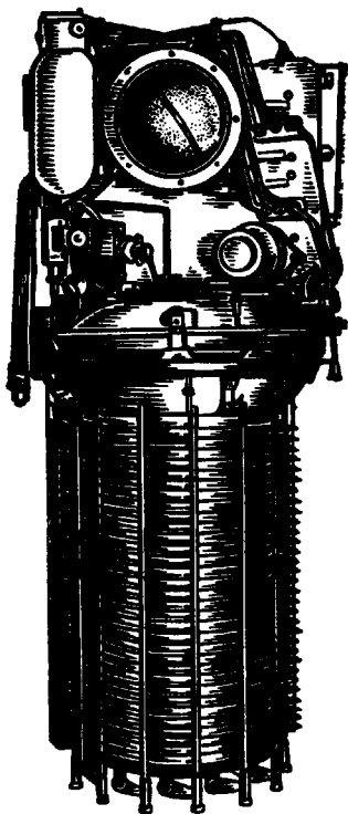
Рис. 6.3. Электрохимический генератор фирмы Pratt and Whitney для космического корабля «Аполлон»
