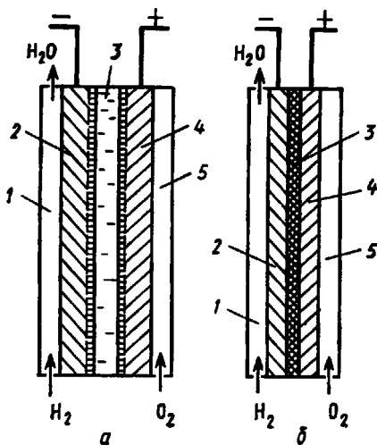
Рис. 6.2. Схема кислородно-водородного топливного элемента со свободным (а) и матричным (б) электролитом:
