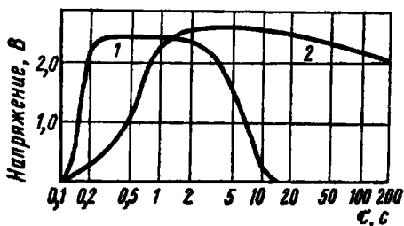
Рис. 5.4. Типичные разрядные характеристики тепловых батарей в расчете на элемент:
