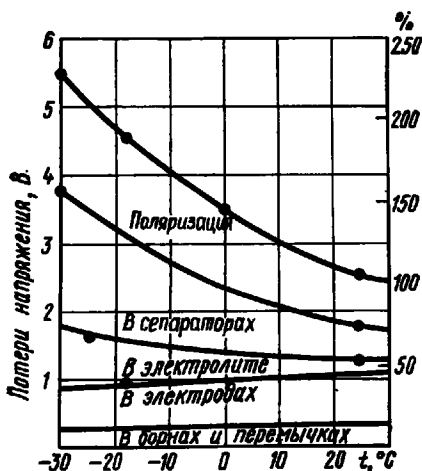
Рис. 7.10. Распределение составляющих баланса напряжения батарей 6СТ-132 в начале разряда током 396 А в зависимости от температуры
