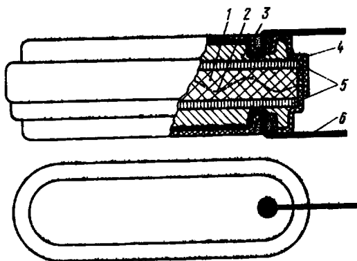
Рис. 4.4. Устройство чашечного марганцево-никелевого элемента:
