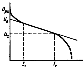
Рис. 3.2. Типичная вольт-амперная характеристика химического источника тока
