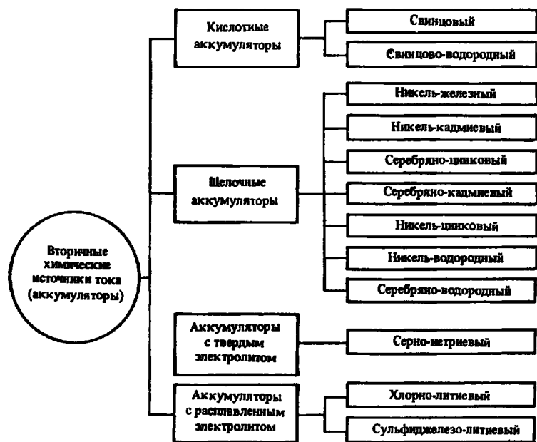
Схема 2.2. Классификация вторичных ХИТ
