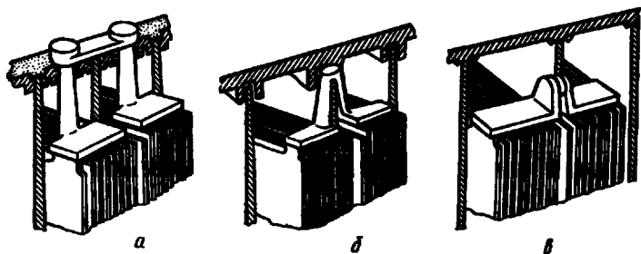
Рис. 7.2. Способы соединения аккумуляторов:
