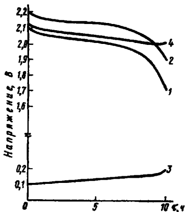
Рис. 7.7. Изменение напряжения (1), НРЦ (4), потенциала положительного (2) и отрицательного (3) электрода свинцового аккумулятора в процессе разряда
