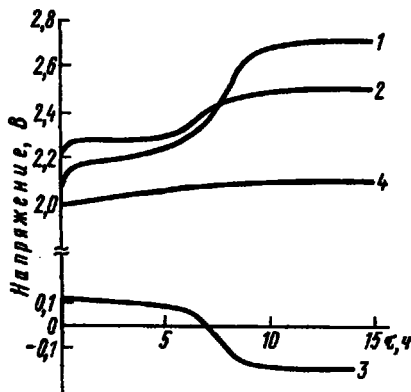
Рис. 7.6. Изменение напряжения (1), НРЦ (4), потенциала положительного (2) и отрицательного (3) электрода свинцового аккумулятора в процессе заряда
