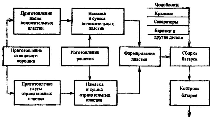
Схема 7.1. Краткая технологическая схема производства стартерных свинцовых батарей
