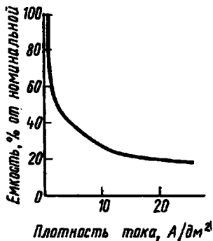
Рис. 7.8. Зависимость емкости стартерных батарей от плотности разрядного тока
