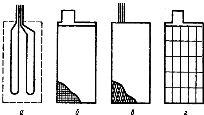
Рис. 2.1. Варианты каркаса электрода открытого типа:
