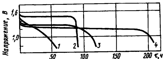
Рис. 4.12. Разрядные характеристики щелочных малогабаритных элементов:
