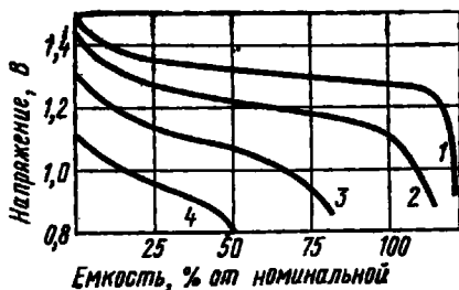
Рис. 8.5. Разрядные характеристики ламельного НЖ аккумулятора при температуре 20^{\circ}\text{C} :
