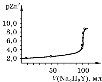
Рис. 9.2. Кривая титрования 100,0 мл 0,01M Zn(NO_3)_2 при рН10 в присутствии NH_3 + NH_4Cl 0,01M раствором Na_2H_2Y
