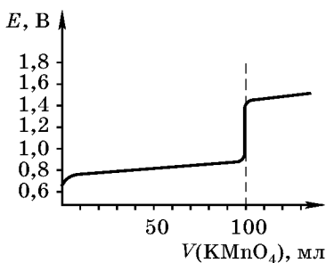
Рис. 11.1. Кривая титрования 100,0 мл 0,1М \text{FeSO}_4 0,1н. раствором \text{KMnO}_4 ( f_{\text{э.кв.}} = 1/5 ) при [\text{H}^+] = 1,0
