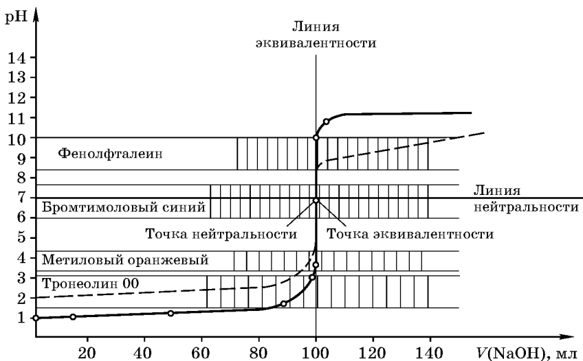
Рис. 7.1. Кривая титрования 100,0 мл 0,1М НСl 0,1М раствором NaOH
