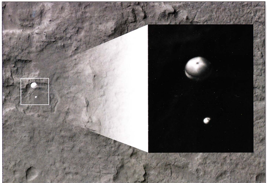
Спуск посадочной капсулы MSL в марсианской атмосфере, сфотографированный с ареоцентрической орбиты аппаратом MRO.
