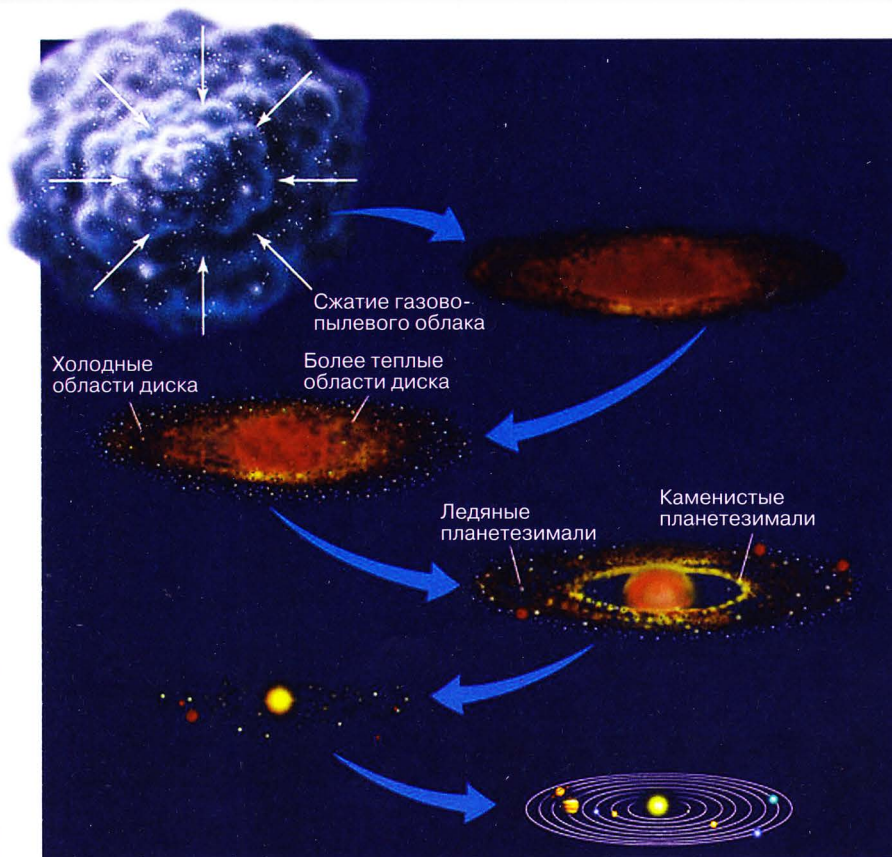
Последовательные этапы формирования Солнечной системы: сгущение газовой-пылевой облака, начало ядерных реакций в звезде и формирование протопланетного диска, образование планетезималей, а затем — планет.
