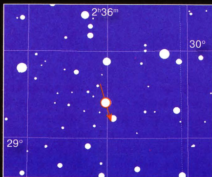
Оккультация звезды HIP 12115 ( \alpha = 2^h 36^m 04^s , \delta = 29^\circ 24' 14'' ) астероидом Сеченов (5234 Sechenov) 4 октября
