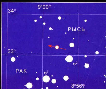
Оккультация звезды TYC 2488-479 ( \alpha = 8^{\text{h}}58^{\text{m}}21^{\text{s}} , \delta = 33^{\circ}11'42'' ) астероидом Эгерия (13 Egeria) 28 октября. Координаты звезд даны на эпоху 2000.0. Детали явления — в тексте
