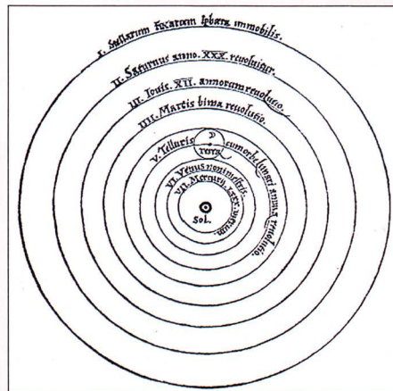
Модель мира Коперника.
