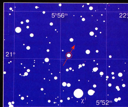
Оккультация звезды TYC 1324-366 ( \alpha = 5^h 55^m 14^s , \delta = 21^\circ 04' 39'' ) астероидом №21967 (1999 WS9) перед рассветом 23 октября
