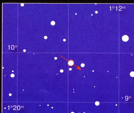
Оккультация звезды HIP 5898 ( \alpha = 1^h 15^m 47^s , \delta = +9^\circ 47' 06'' ) астероидом Тампере (1497 Tampere) в ночь с 22 на 23 октября
