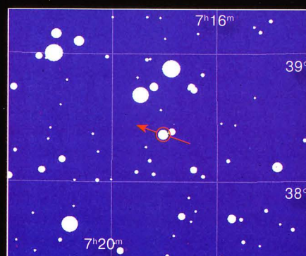
Оккультация звезды HIP 35338 ( \alpha = 7^h 18^m 01^s , \delta = 38^\circ 21' 51'' ) астероидом Тюрингия (934 Thuringia) в ночь с 22 на 23 октября
