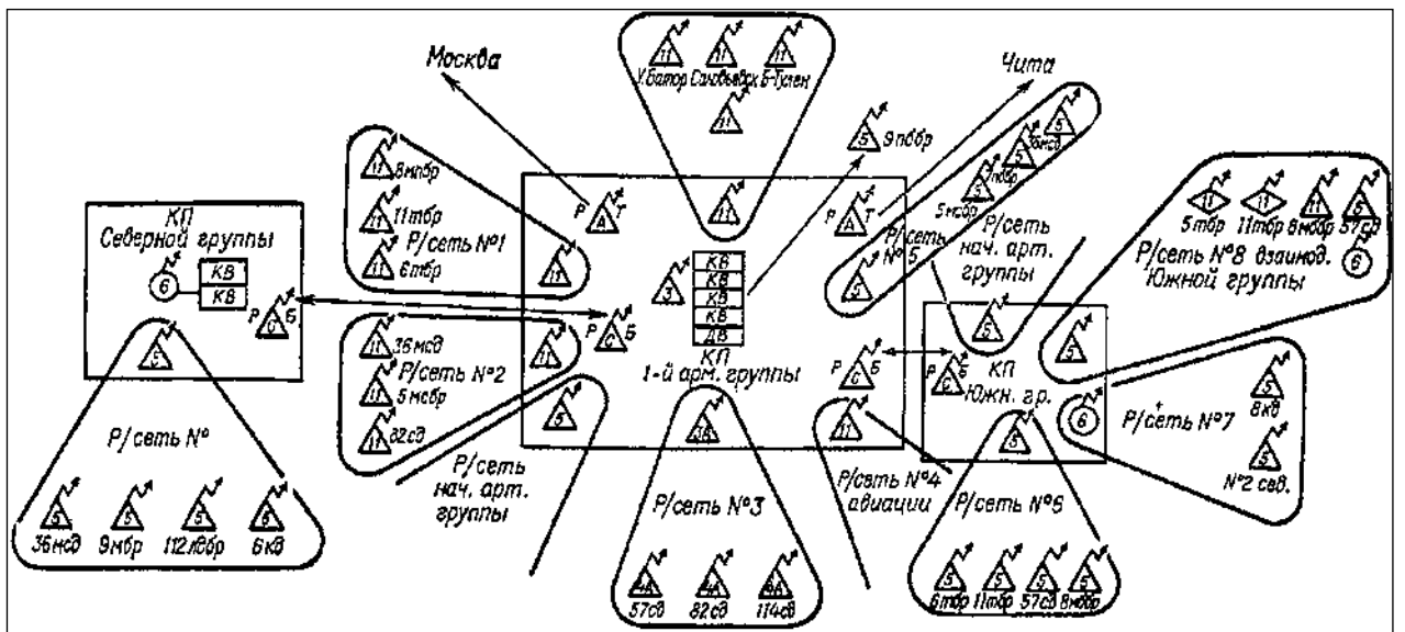
Рис. 2. Схема организации радиосвязи 1-й армейской группы войск в боях на р. Халхин-Гол Август 1939 г.
