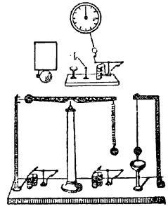
Рис. 4. Электрический сейсмоскоп сист. Forster'a
