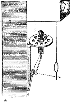
Рис. 3. Сейсмоскоп сист. Lesaux.
