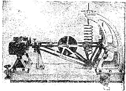
Рис. 7. Вертикальный сейсмограф системы Голицына.
