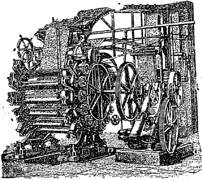
Рис. 3. Ситцепечатная машина.
