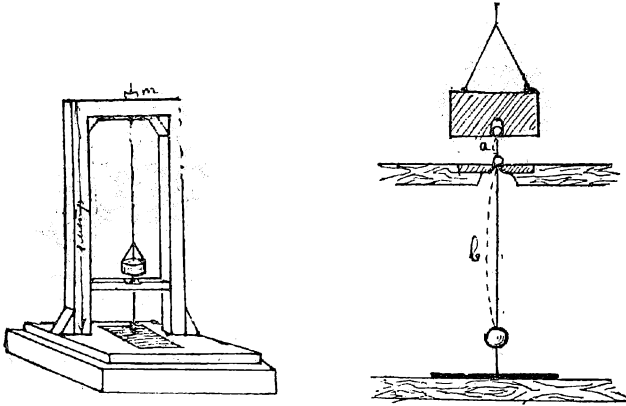
Рис. 10 и 11. Чертежи простейшей конструкции любительского сейсмографа.
