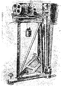
Рис. 5. Горизонтальный сейсмограф сист. Вихерта
