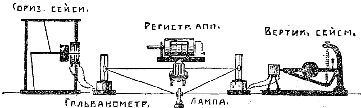
Рис. 6. Схема рабочей установки вертикального сейсмографа сист. Голицына.
