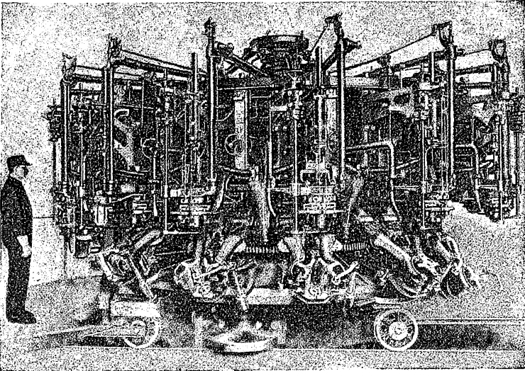
Рис. 6 Машина для выдувания бутылок, заменяющая вредную и опасную работу ста человек—стеклодувов
