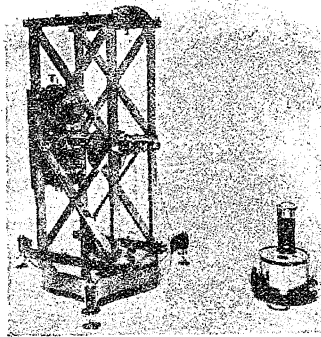
Рис. 8. Горизонтальный сейсмограф сист. Голицына.
