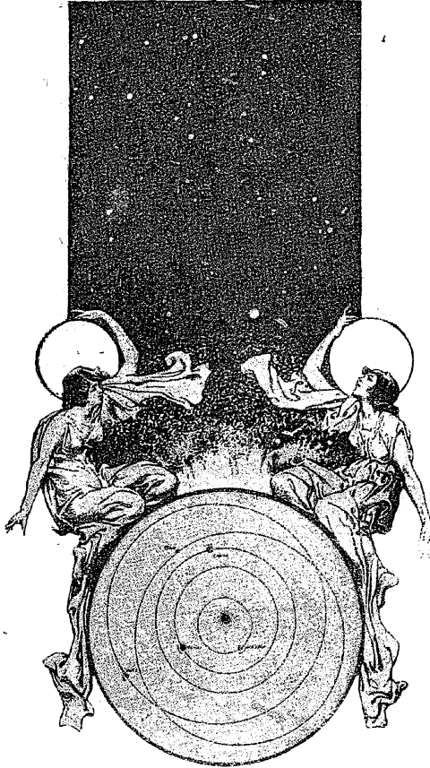
Вверху — фотографии, которая обнаруживает наличие астероида Эрос, диаметром в 23 километра. Пластика, выставленная в течение нескольких часов, двигалась для того, чтобы удерживать звезды в фокусе прибора. Эрос, движущийся относительно быстрее, представляется в виде четкой, а не точечной (в верхней части снимка). Ниже: расположение планет друг относительно друга в 1930—31, когда Эрос будет находиться от Земли на расстоянии 16.200.000 миль (1 миль = 1,609 километра).
