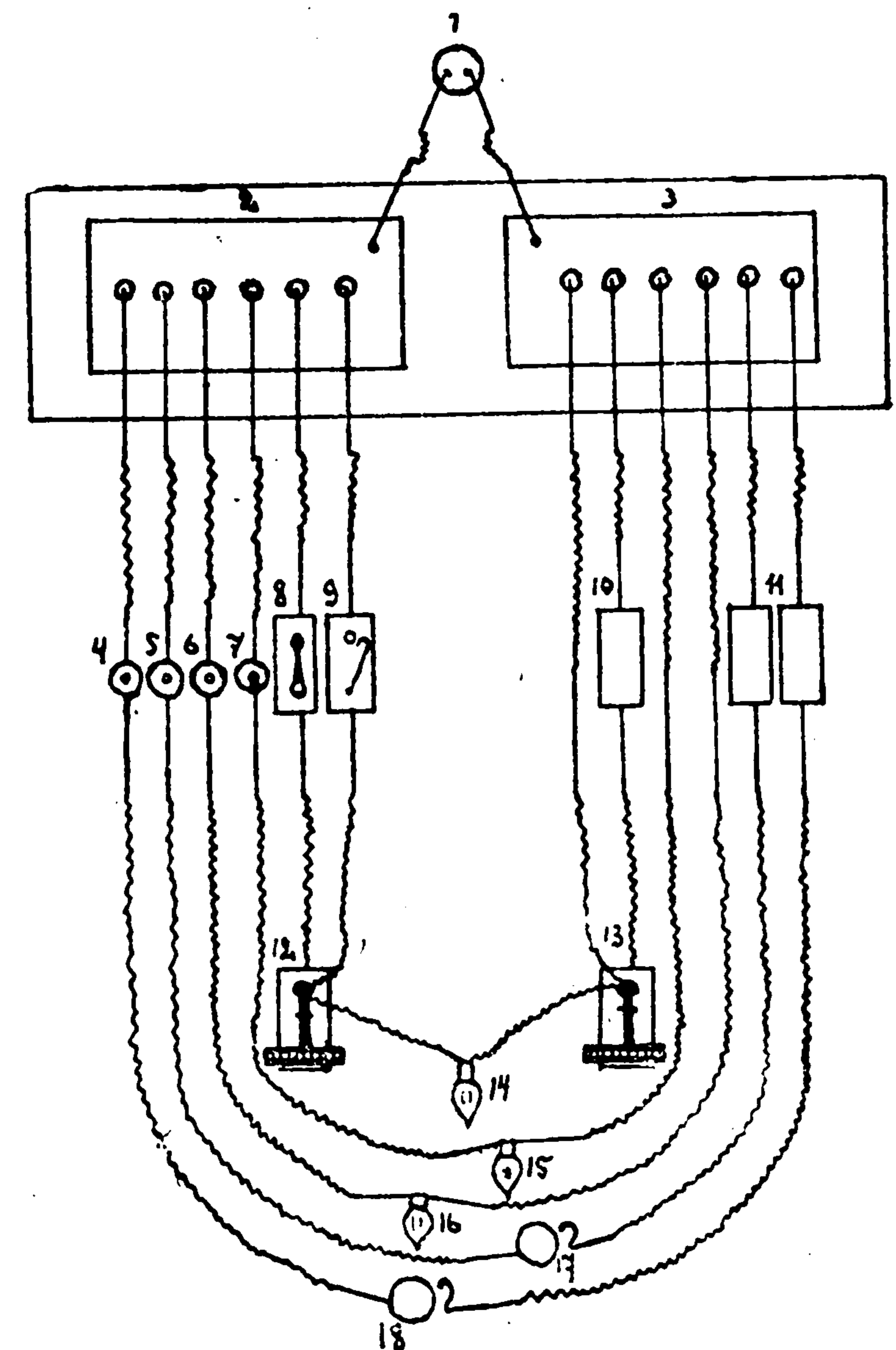
Рис. 4. Схема распределения электрической сигнализации в камере.
