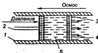
Рис. 6.2 Обратный осмос
