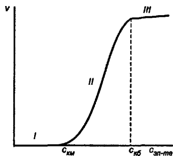
Рис. 10.1 Зависимость скорости коагуляции от концентрации электролита
