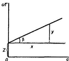
Рис. 3.8 Зависимость величины c/\Gamma от концентрации ПАВ
