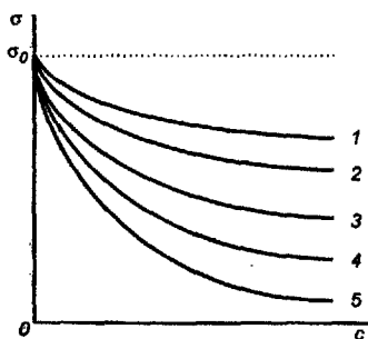
Рис. 3.4 Изотерма поверхностного натяжения некоторых кислот
