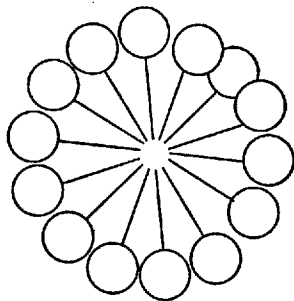
Рис. 12.3 Мицелла Гартли
