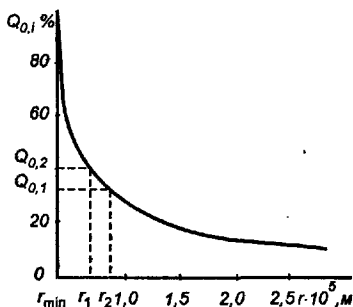
Рис. 15.6 Интегральная кривая распределения талька в воде
