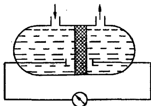
Рис. 8.3 Схема возникновения потенциала течения
