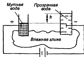
Рис. 8.2 Схема электрофореза
