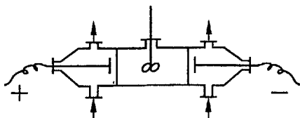
Рис. 6.1 Схема электродиализатора
