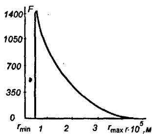
Рис. 15.7 Дифференциальная кривая распределения талька в воде
