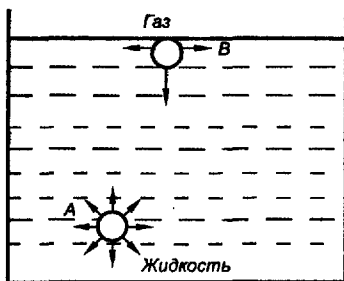
Рис. 2.1 Схема возникновения поверхностной энергии
