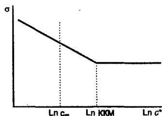
Рис. 12.6 Зависимость поверхностного натяжения от \ln c
