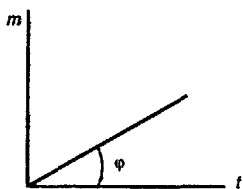
Рис. 15.3 График седиментации монодисперсной системы
