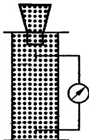
Рис. 8.4 Схема возникновения потенциала седиментации
