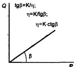
Рис. 11.3 Зависимость расхода жидкости от давления
