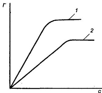
Рис. 4.1 Изотермы адсорбции при двух температурах
