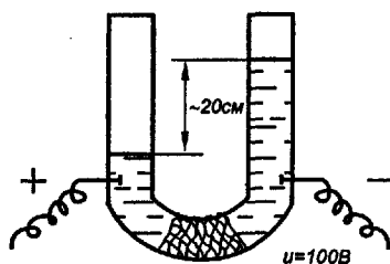
Рис. 8.1 Схема электроосмоса
