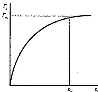
Рис. 3.3 Изотерма адсорбции
