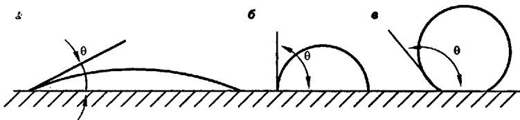
Рис. 5.1 Различные случаи неполного смачивания
