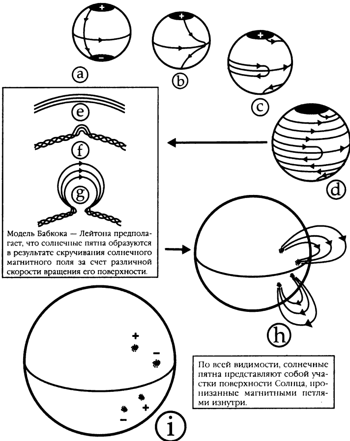
Рис. А14. Известно, что вариации солнечного излучения совпадают с изменениями активности солнечных пятен. В 1961 году английские инженеры Бабкок и Лейтон предположили, что солнечные пятна возникают в результате скручивания двух отдельных магнитных полей Солнца. Таким образом, солнечное излучение и плодovitость живых существ на Земле коррелируются с активностью солнечных пятен.
