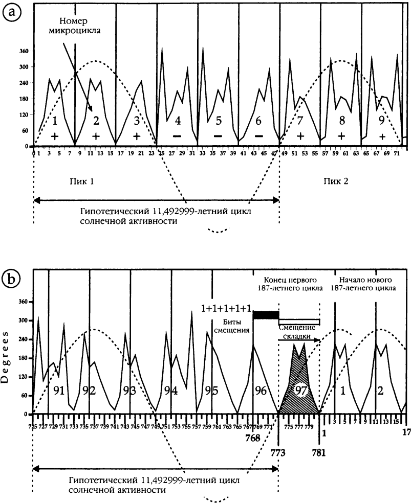
Рис. А1б. (а) Первые 9 циклов в серии из 97 микроциклов, или импульсов, которые составляют один 187-летний цикл солнечной активности, демонстрируют гипотетический 11,492999-летний цикл (пунктирная линия). (б) Последние 7 циклов в серии из 97 микроциклов; черная горизонтальная черта отмечает конец одного 187-летнего цикла (96 микроциклов), сдвинутого вперед на 5 делений с 768 до 773. Еще восемь делений отделяют старый фундаментальный цикл (белая полоса над словами «смещение складки») от нового фундаментального цикла, который начинается после бита 781.
