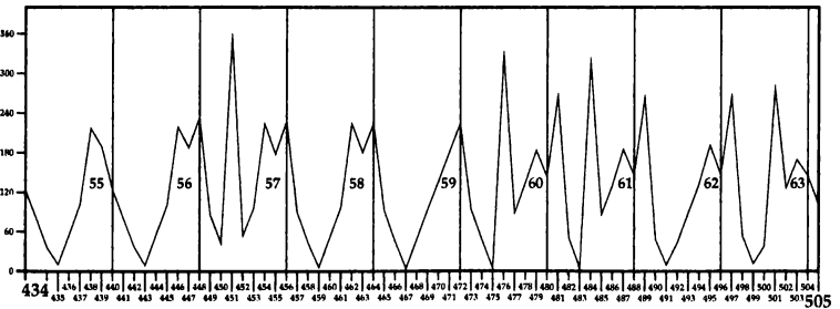
Интервал времени каждые 87,4545 дня
