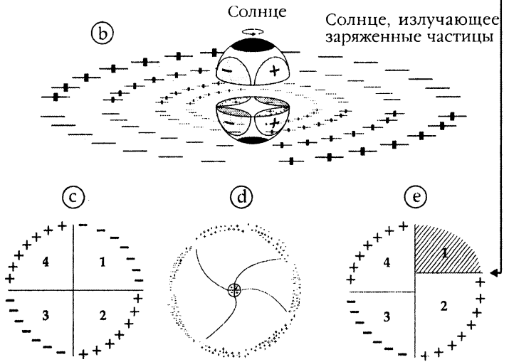
Идеализированная схема магнитного поля Солнца
