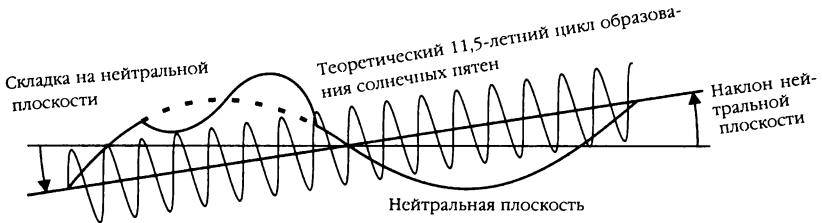
Рис. А18. Более мелкие циклы представляют собой теоретический 11,5-летний цикл солнечной активности. Именно они искажают нейтральную плоскость, придавая ей наблюдаемую искривленную форму.
