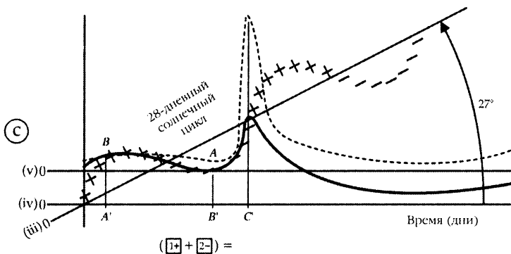
Рис. Аб. (а) Поперечный разрез Солнца; полярная область закрашена черным цветом, а квадранты экваториального поля указаны цифрами 1, 2, 3 и 4. Эмиссия солнечного ветра в каждом квадранте имеет положительную или отрицательную полярность, как показано на рисунке. (б) ФСР коррелируется с ЦСР в пределах квадрантов 1 и 2, выключается на 14-й день, и быстро разлагается. (с) ФСР + ЦСР (квадранты 1 и 2) вместе дают пик ЛГ на 14-й день цикла.
