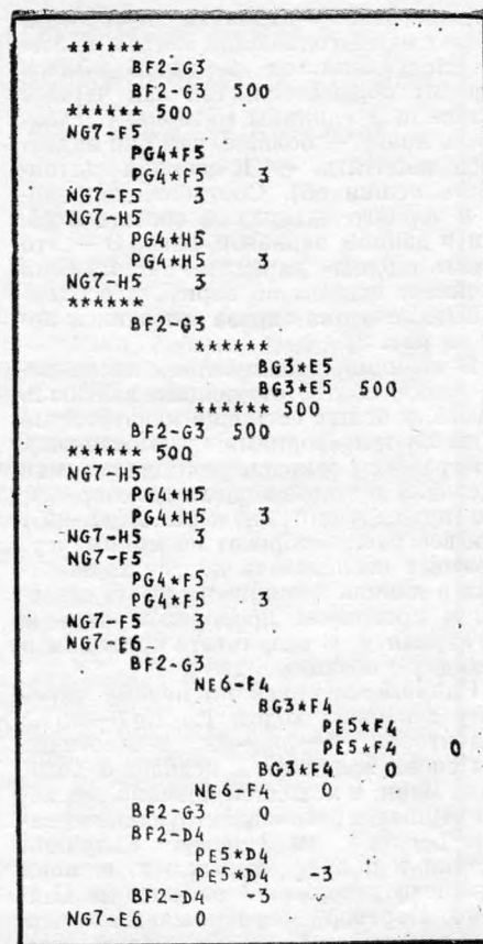
Рис. 3. Пример перебора ходов, выполненного программой формирования зоны. В машинной распечатке Кр—К, С—В, К—N, п—P, пропуск хода — *****
