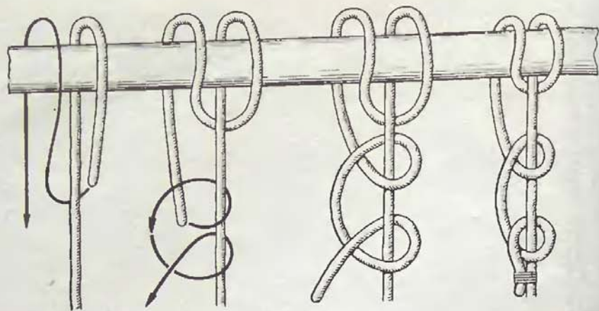
Рис. 14. Штык с обносом
