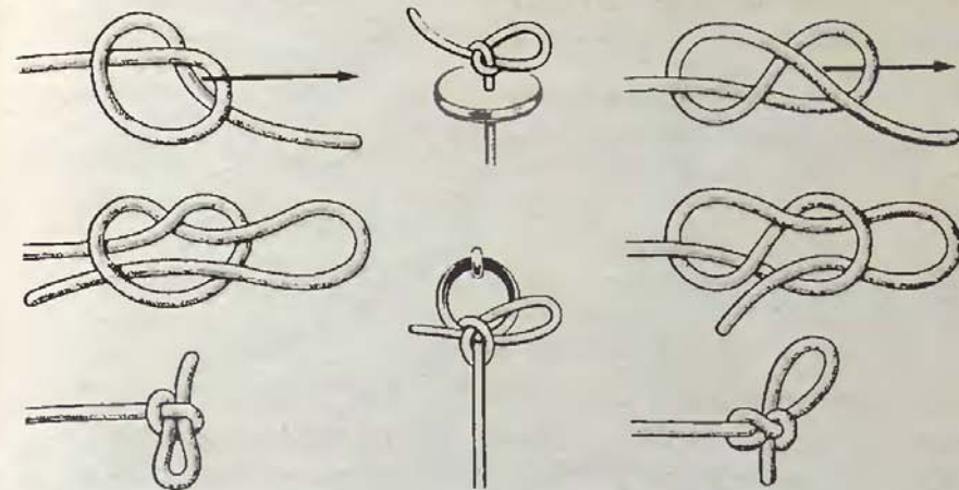
Рис. 91. Развязывающийся простой узел
