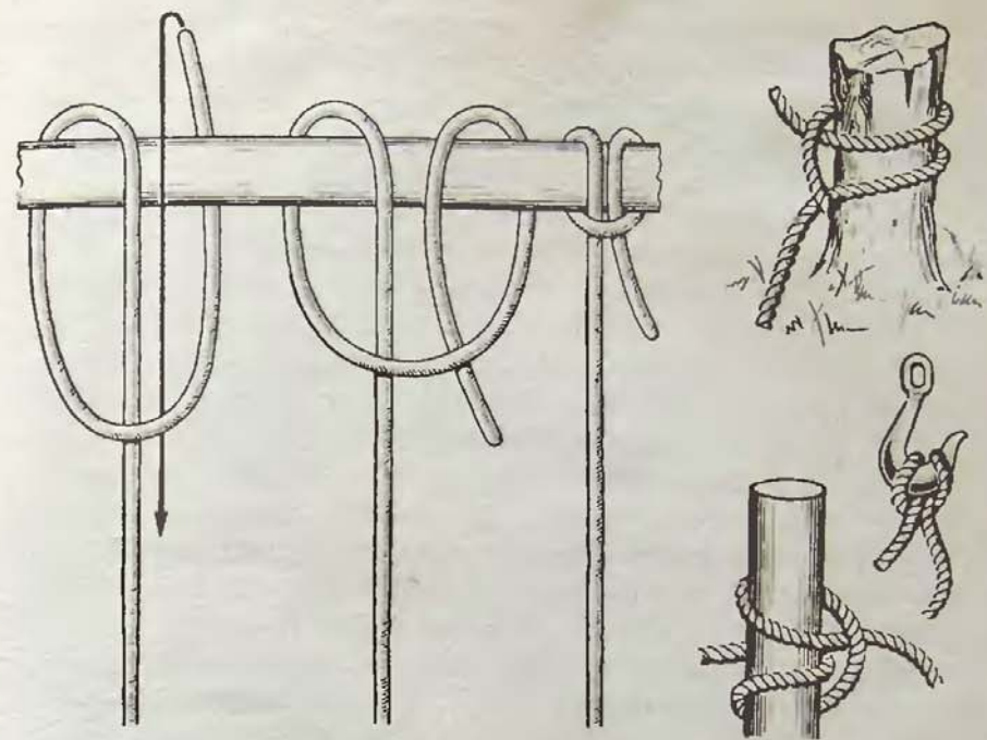
Рис. 46. Коровий узел
