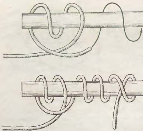
Рис. 60. Стопорный узел
