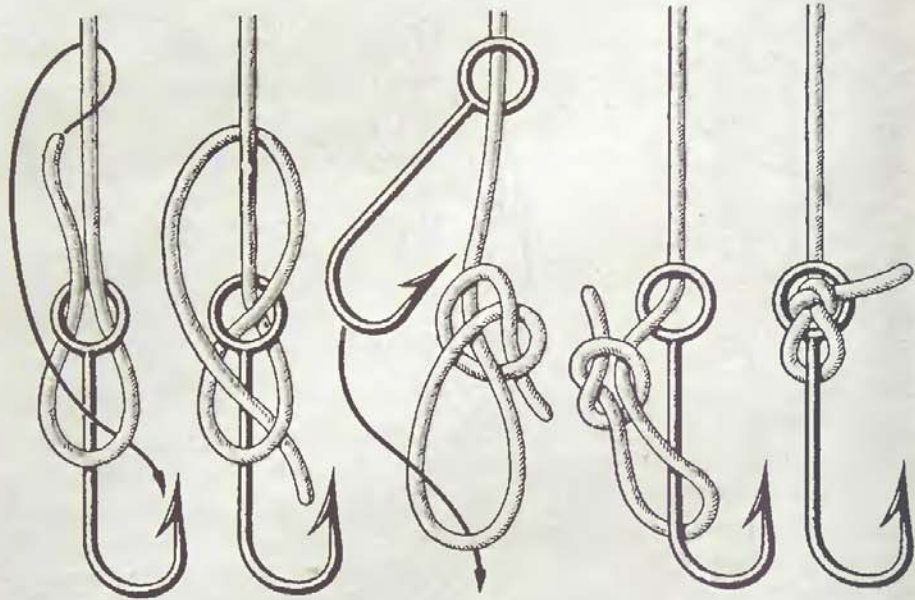
Рис. 122. Рыбацкая восьмерка
