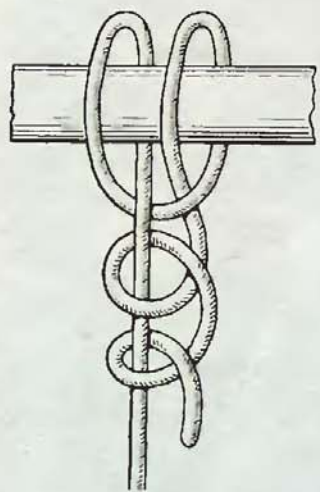
Рис. 17. Мачтовый штык
