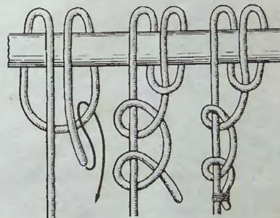
Рис. 16. Обратный штык
