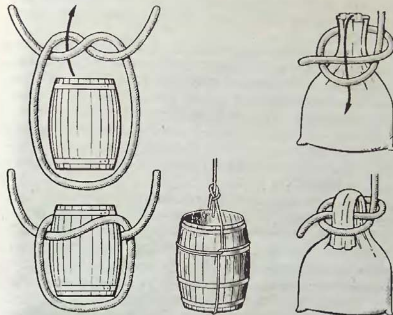
Рис. 108. Бочечный узел
