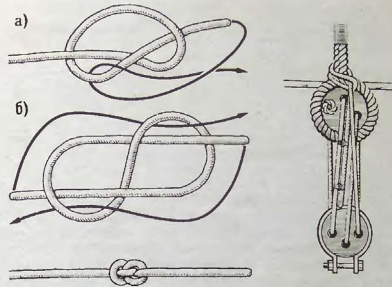
Рис. 5. Юферсный узел: а — первый способ вязки; б — второй способ вязки
