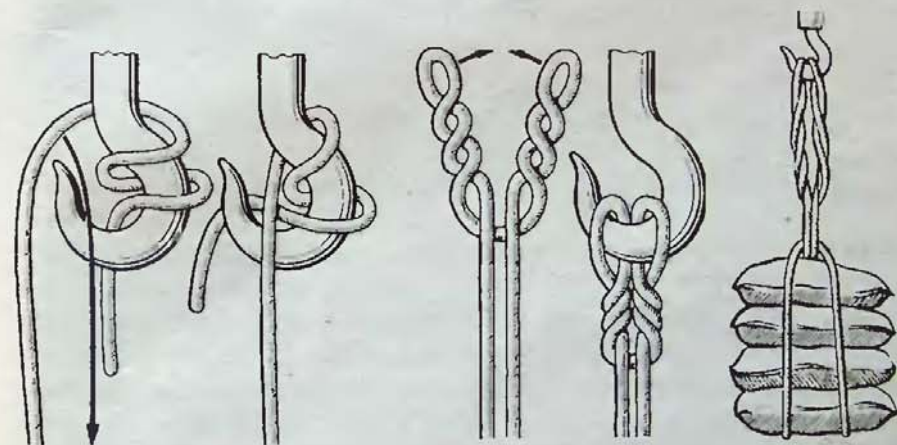
Рис. 106. Гачный узел со шлагом
