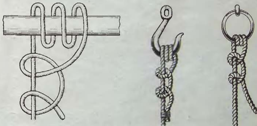
Рис. 13. Простой штык с двумя шлагами
