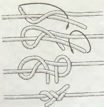
Рис. 32. Пакетный узел
