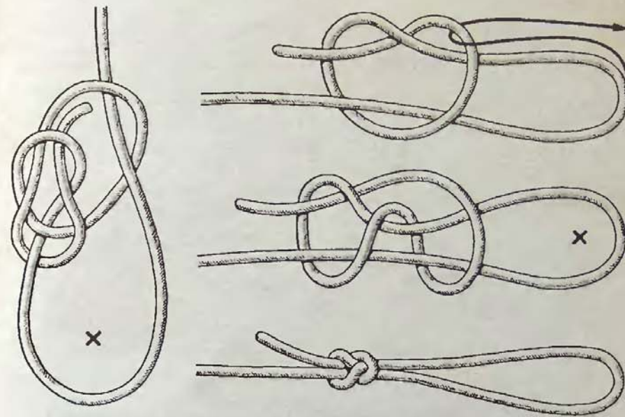
Рис. 85. Бегущий булинь
