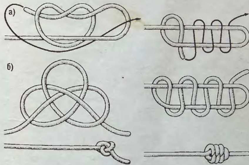
Рис. 7. Множественная восьмерка
