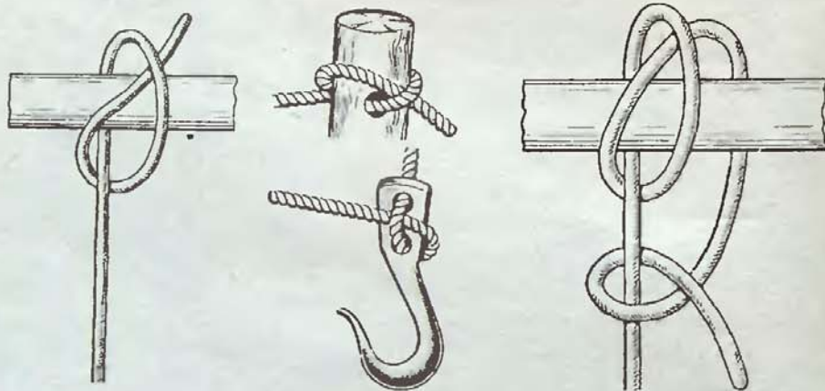
Рис. 44. Самозатягивающийся узел
