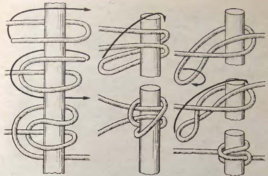
Рис. 62. Зигзаговым узел
