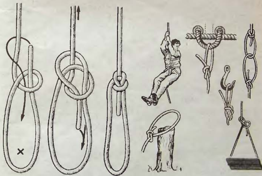
▲ Рис. 76. Беседочный узел
