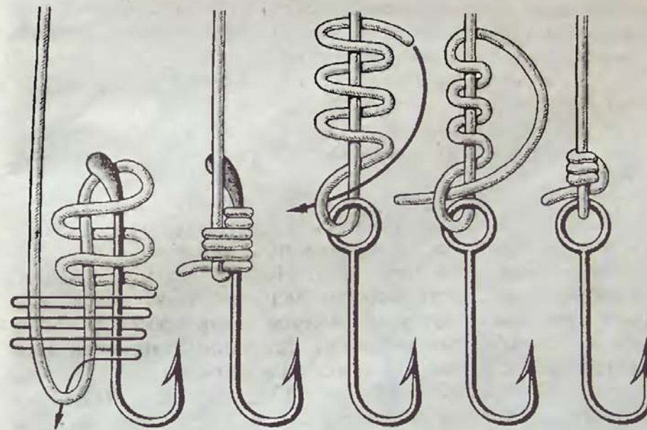
Рис. 125. Ступенчатый узел
