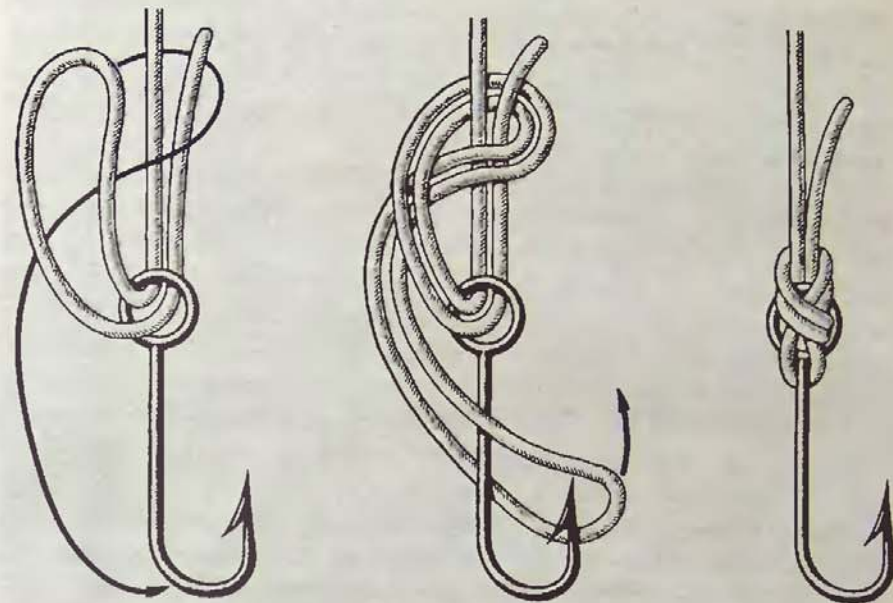
Рис. 124. Калифорнийский узел
