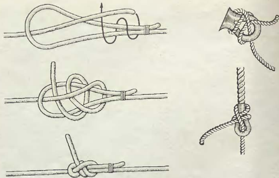
▲ Рис. 39. Брам-шкотовый узел
