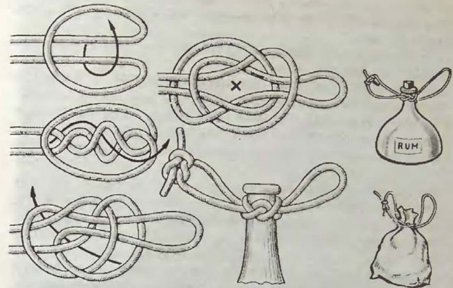
Рис. 111. Амфорный узел
