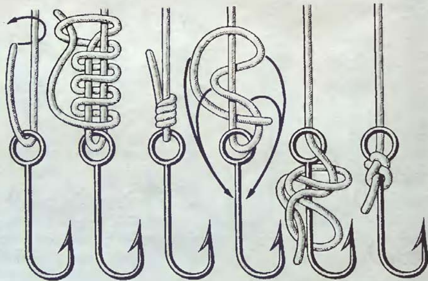
Рис. 127. Акулий узел
