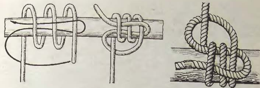
Рис. 57. Фаловый узел
