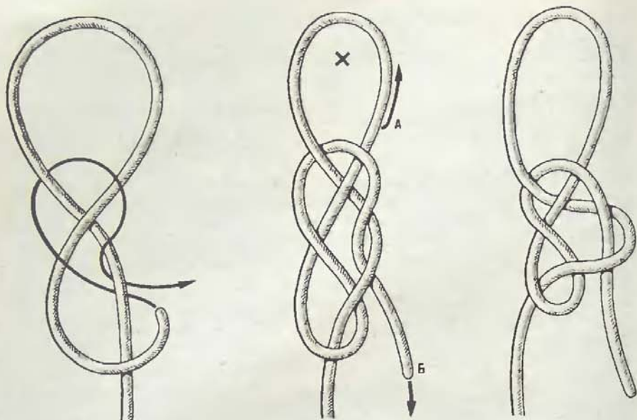
Рис. 118. Кабестановая петля
