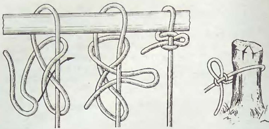
Рис. 102. Курьерский узел
