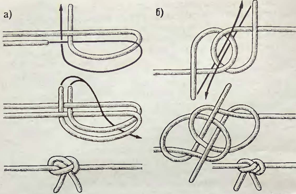
Рис. 41. Скорняжный узел: a — первый способ вязки; b — второй способ вязки
