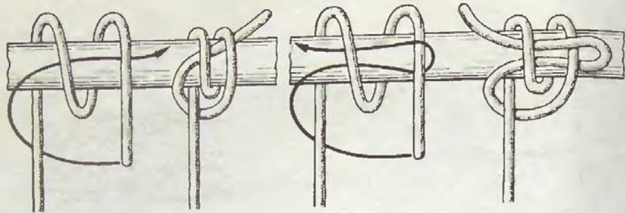
Рис. 56. Лисельный узел
