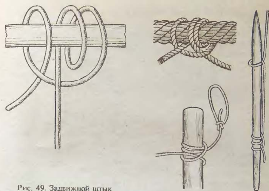
Рис. 49. Задвижной штык
