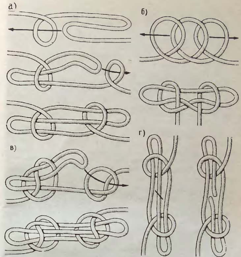
Рис. 113. Колышка («баранья нога»): а — первый способ вязки; б — второй способ вязки; в — «баранья нога» со сваячными узлами; г — принцип действия «бараньей ноги»
