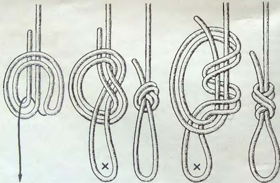
Рис. 66. Дубовая петля
