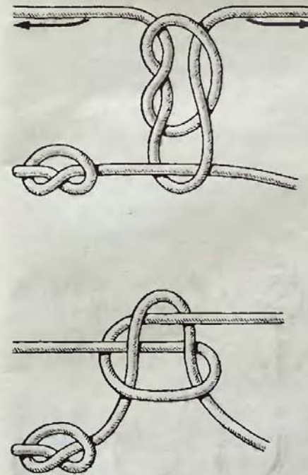
Рис. 131. Поводковый на основе бегущего узла
