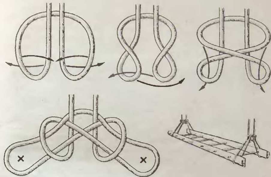
Рис. 78. Боцманский узел (испанский беседочный)
