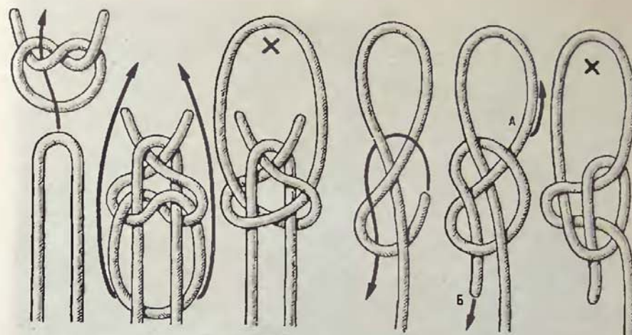
Рис. 116. Лучниковская петля
