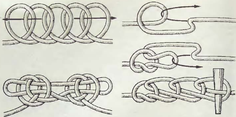
Рис. 115. «Мартышкина цепочка»
