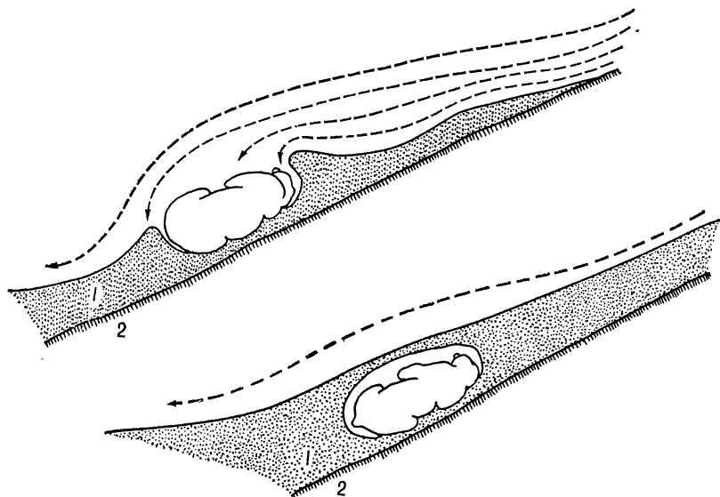
Нередко «строят» берлогу снег и ветер: 1— снег, 2— грунт
