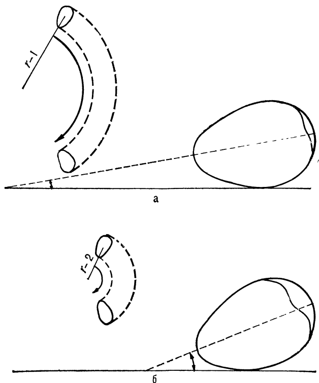
Положение яйца толстоклювой кайры на гнездовом карнизе и радиус окружности, описываемой им при толчке: а — ненасиженное яйцо, б — насиженное яйцо
