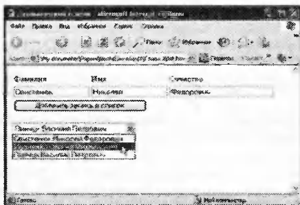
Рис. 3.8. Динамическое добавление пунктов в список
