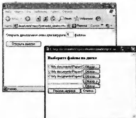
Рис. 7.8. Открытие диалогового окна выбора файлов для загрузки на сервер
