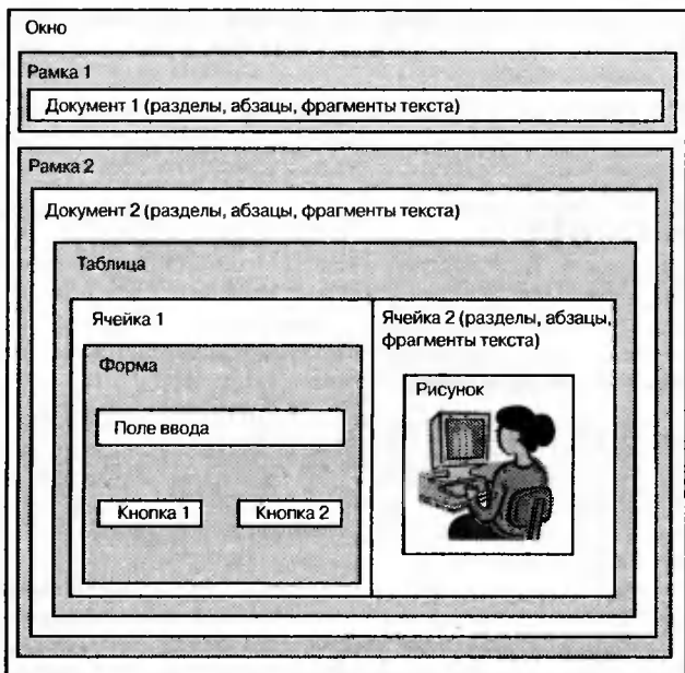
Рис. 1.3. Иерархия объектов окна обозревателя
