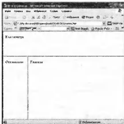
Рис. 2.16. Набор рамок
