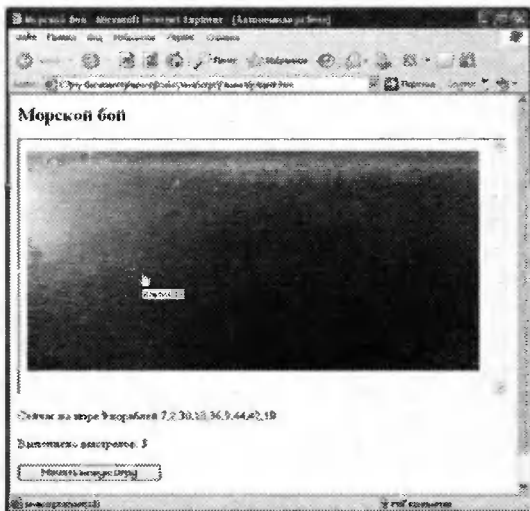
Рис. 6.13. Морской бой
