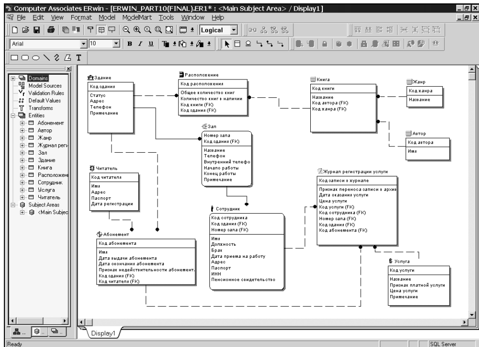
Рис. 10.76. Логическая модель базы данных "Библиотекарь"
