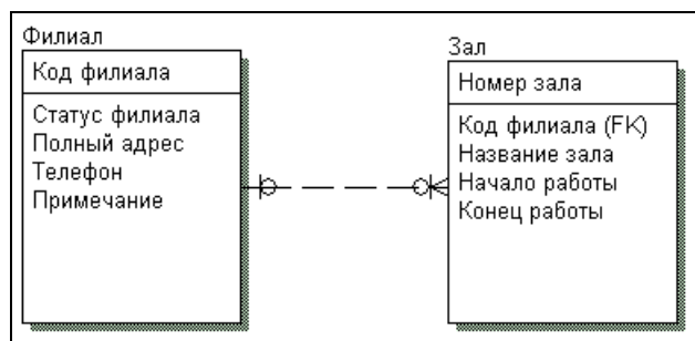
Рис. 10.6. Пример фрагмента логической модели в варианте IE
