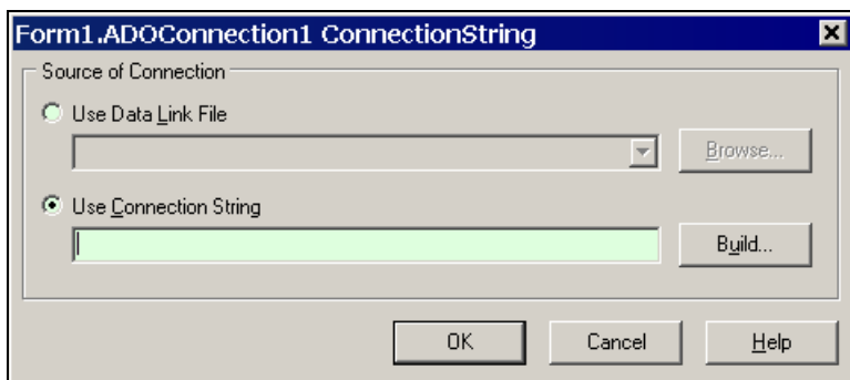
Рис. 4.51. Окно установки ConnectionString
