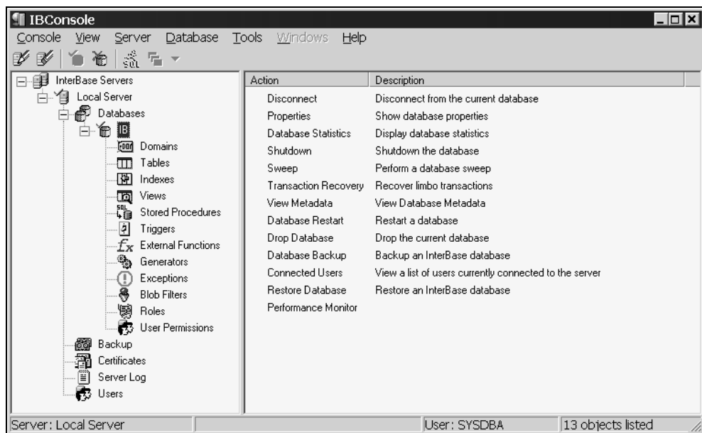
Рис. 3.18. Окно IBConsole после создания базы данных
