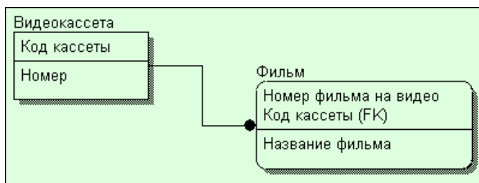
Рис. 10.69. Пример идентифицирующей связи (на каждой видеокассете может быть несколько фильмов, первичный ключ сущности "Фильм" состоит из порядкового номера фильма и кода кассеты, на которой он расположен)
