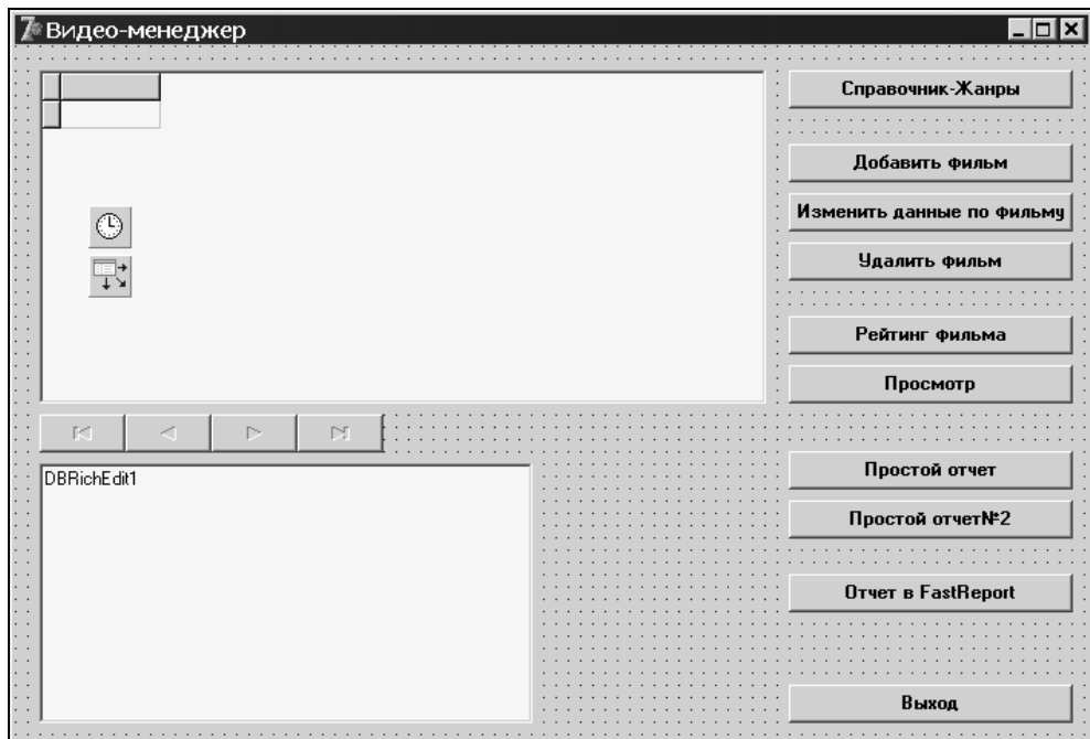
Рис. 8.11. Добавление кнопки вызова отчета на форму MainForm
