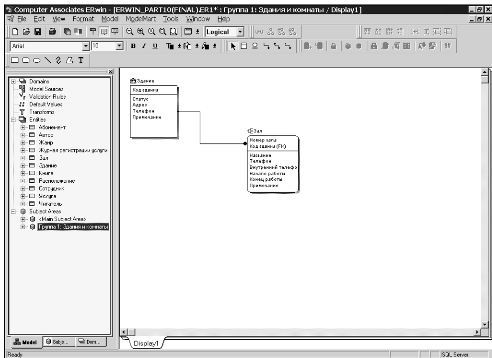
Рис. 10.82. Вид области с добавленными сущностями "Здание" и "Зал"
