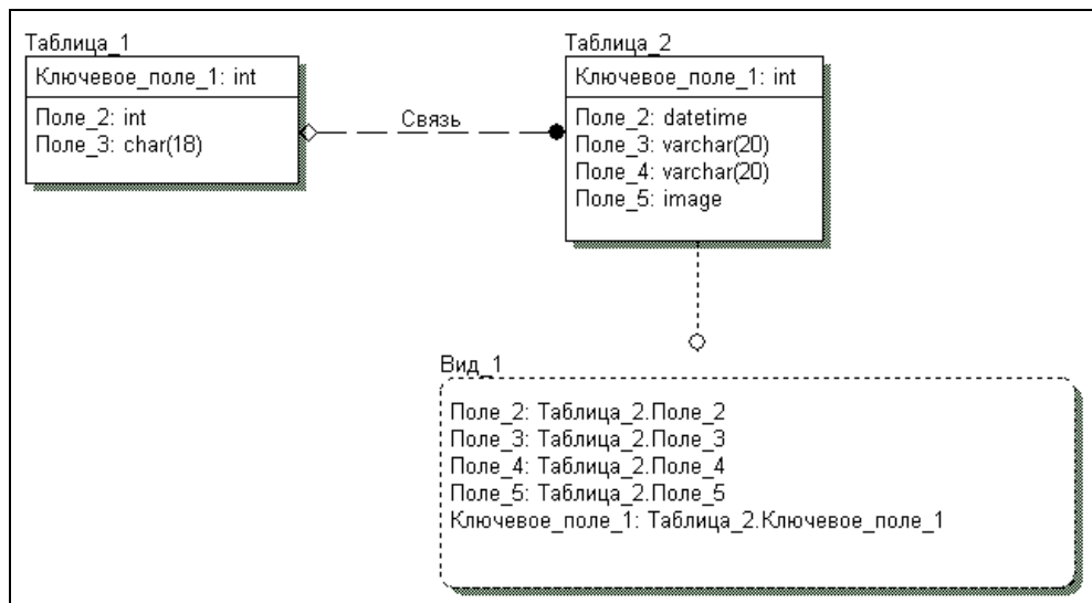
Рис. 10.9. Фрагмент физической модели (вариант IDEF1X)
