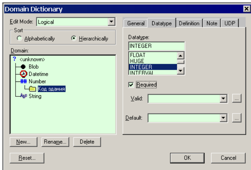
Рис. 10.51. Вкладка Datatype окна Domain Dictionary
