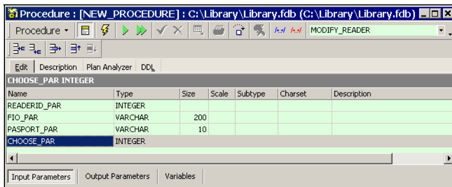
Рис. 5.55. Добавление входных параметров
