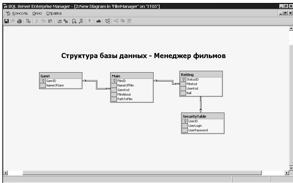
Рис. 4.35. Моя диаграмма базы данных
