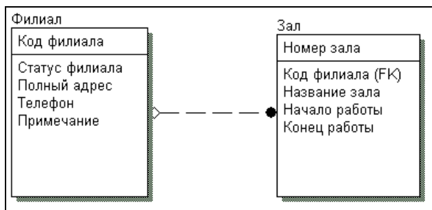
Рис. 10.3. Пример фрагмента логической модели в варианте IDEF1X
