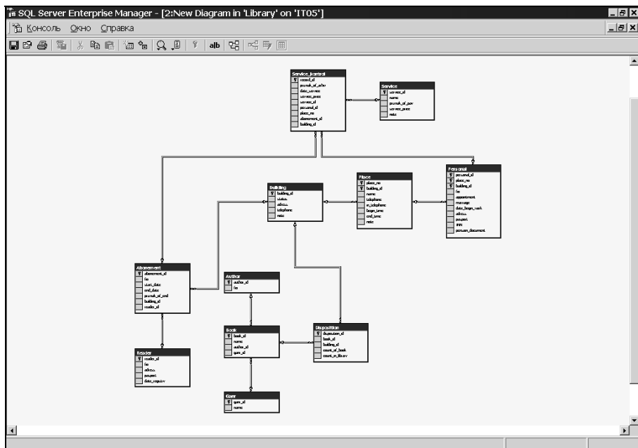
Рис. 10.90. Диаграмма в MS SQL Server для базы данных "Библиотекарь"
