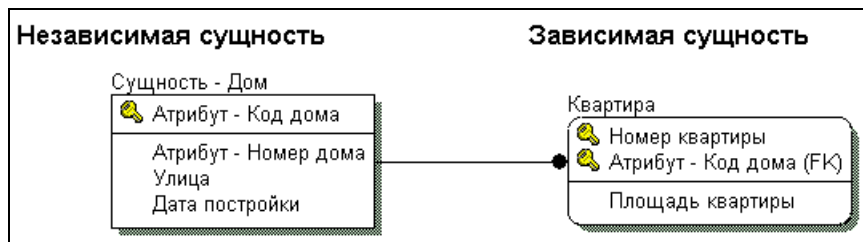
Рис. 10.8. Независимая и зависимая сущности
