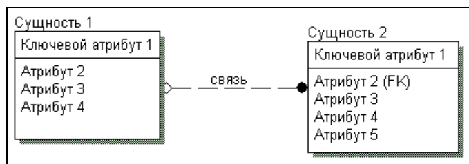
Рис. 10.7. Фрагмент логической модели (вариант IDEF1X)
