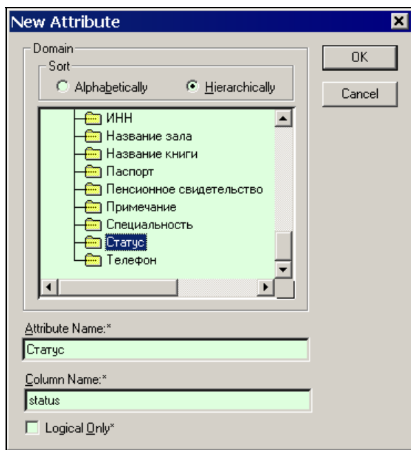
Рис. 10.56. Создание атрибута посредством домена
