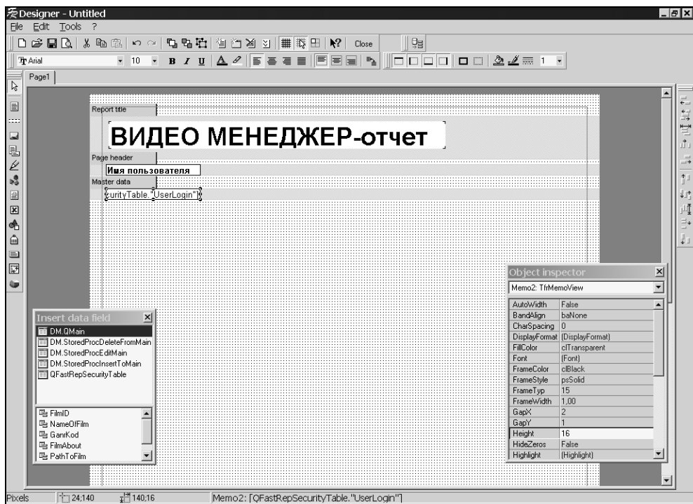
Рис. 8.26. Вид отчета в дизайнера
