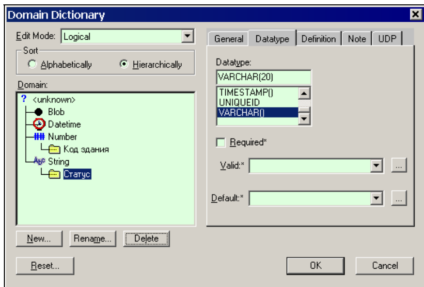
Рис. 10.54. Установка Datatype свойства "Статус"
