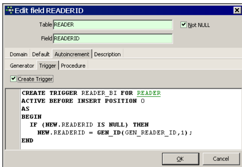
Рис. 5.30. Вкладка Trigger окна редактирования атрибута READERID
