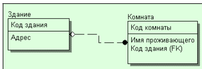
Рис. 10.70. Пример неидентифицирующей связи (каждая комната принадлежит какому-то зданию)
