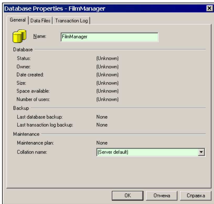
Рис. 4.13. Окно Database Properties
