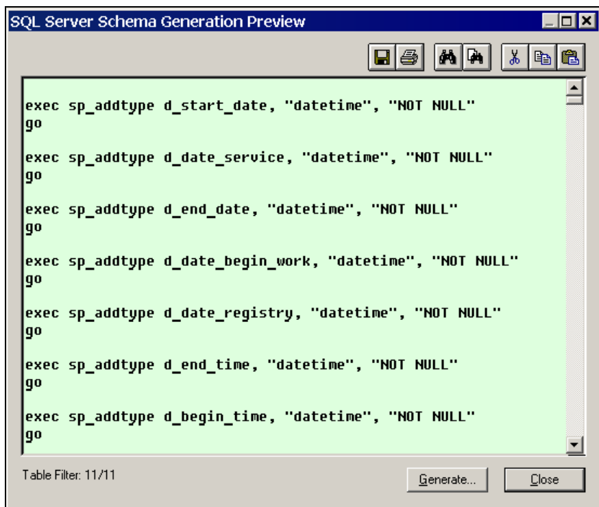
Рис. 10.86. Скрипт для создания базы данных "Библиотекарь"
