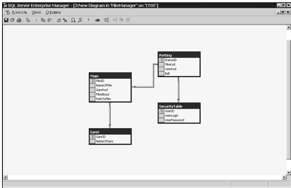
Рис. 4.34. Диаграмма базы данных
