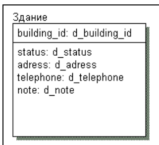
Рис. 10.59. Вид сущности "Здание" в физической модели
