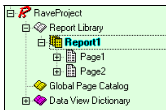
Рис. 7.36. Объект ReportLibrary в инспекторе отчета с активным пунктом Report1
