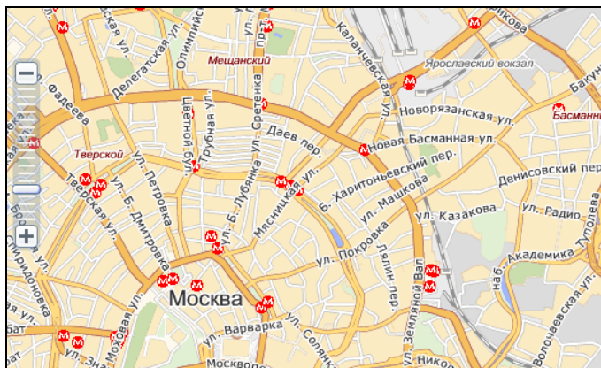
Рис. 3.7. Элемент масштабирования
