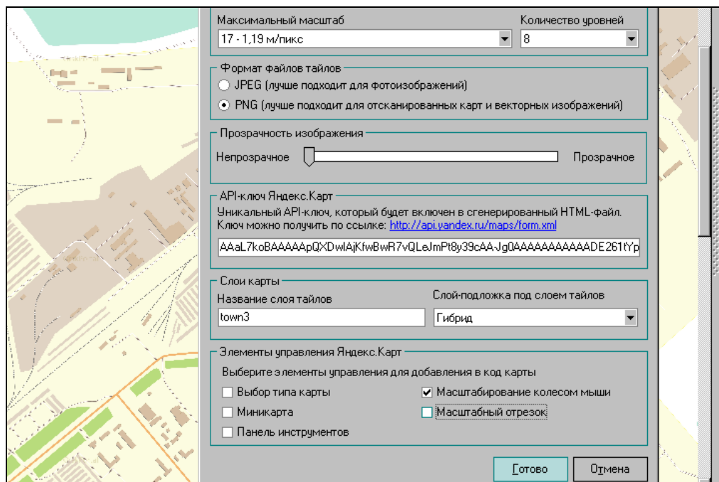
Рис. 4.22. Экспорт карты
