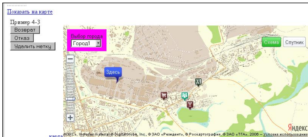
Рис. 4.29. Создание метки
