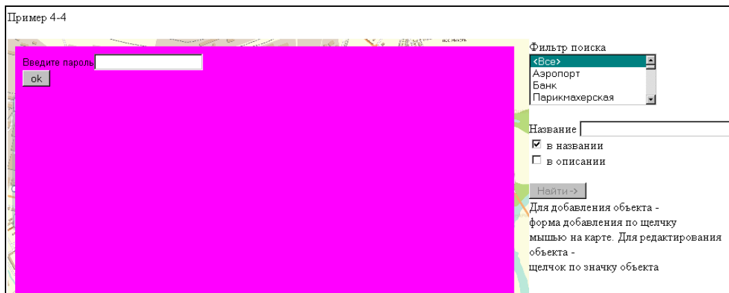
Рис. 4.31. Форма авторизации
