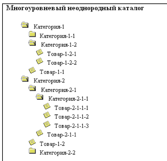
Рис. 1.13. Многоуровневый каталог
