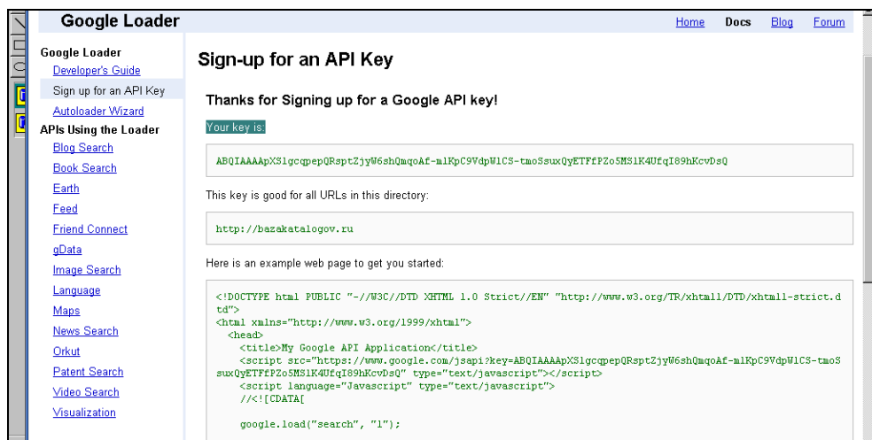
Рис. 7.3. Ключ получен
