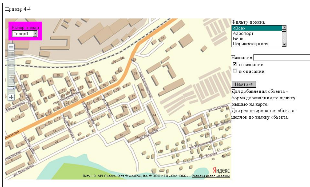
Рис. 4.30. Панель администратора
