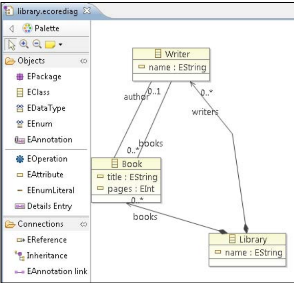
Рис. 17.10. Есоре-диаграмма метамодели библиотеки
