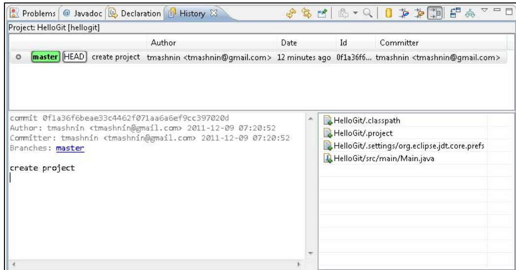
Рис. 3.36. Представление History , отображающее фиксации проекта
