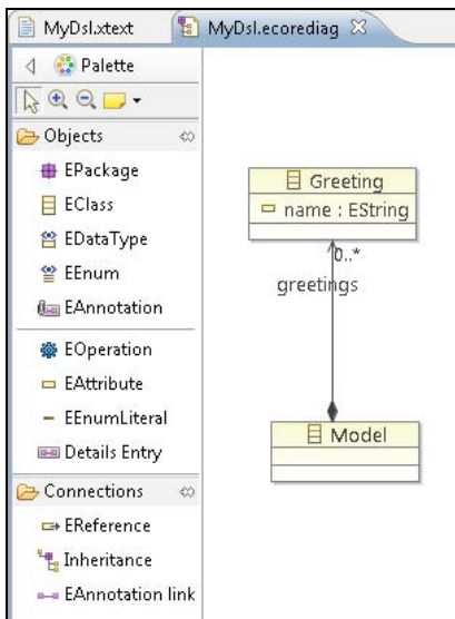
Рис. 17.8. Ecore-диаграмма структуры DSL-языка
