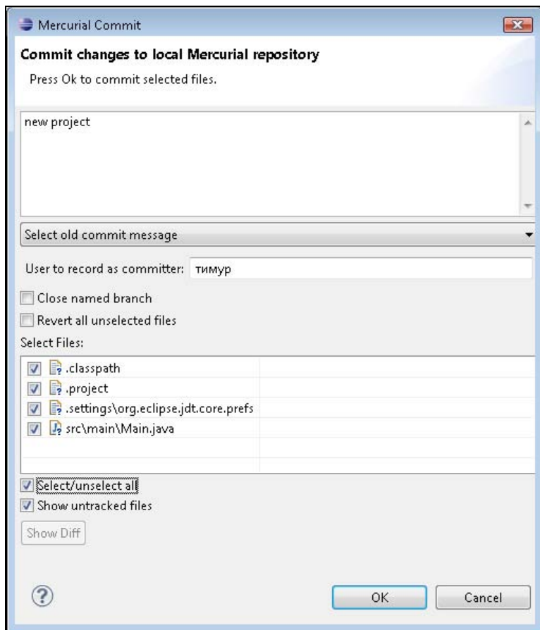
Рис. 3.42. Мастер Mercurial Commit, помогающий создать набор изменений проекта
