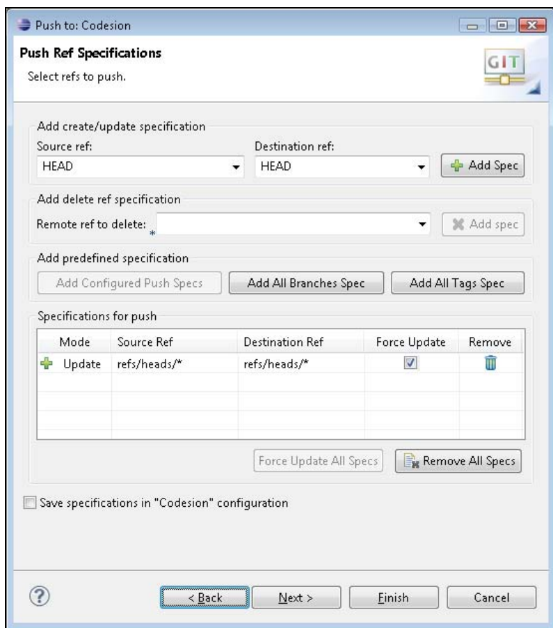
Рис. 3.41. Мастер передачи изменений из локального Git-репозитория в удаленный Git-репозиторий
