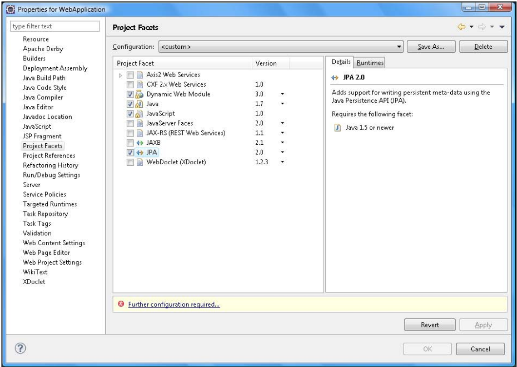
Рис. 14.8. Добавление поддержки JPA в проект приложения
