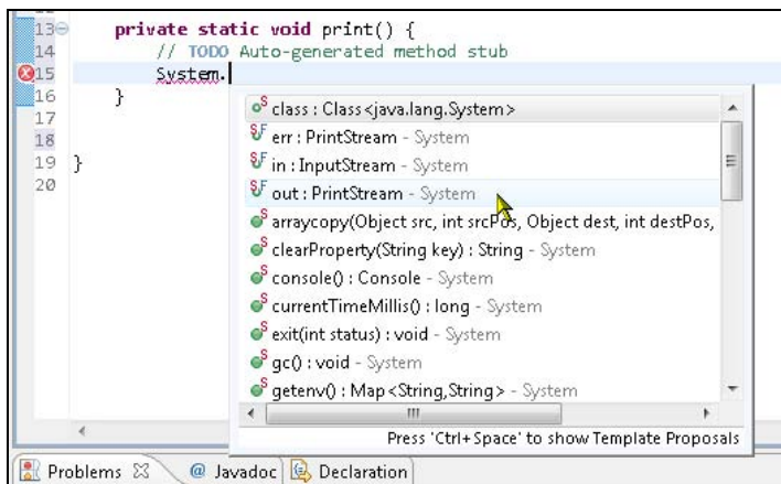
Рис. 1.20. Подсказка Content Assist появляется сама при вводе разделителя ".".
