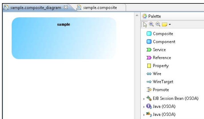
Рис. 12.4. Окно редактора Composite-диаграммы
