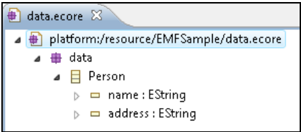
Рис. 17.2. Графическое представление Ecore-модели
