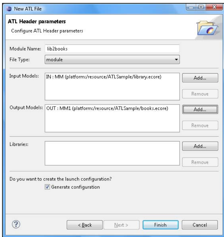
Рис. 17.13. Мастер создания ATL-файла трансформации
