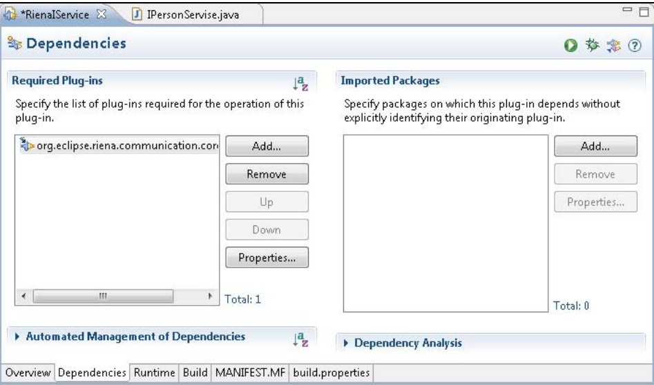
Рис. 11.7. Добавление зависимости от плагина org.eclipse.reina.communication.core
