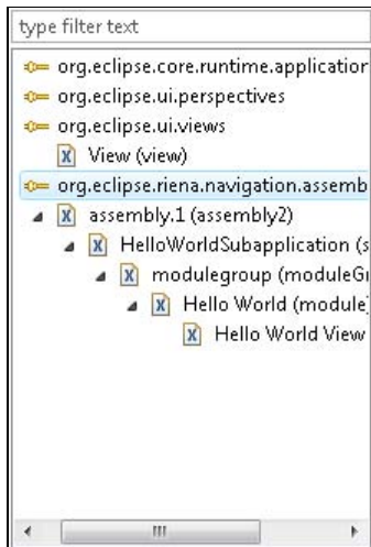
Рис. 11.4. Дерево компонентов GUI-интерфейса Riena-приложения
