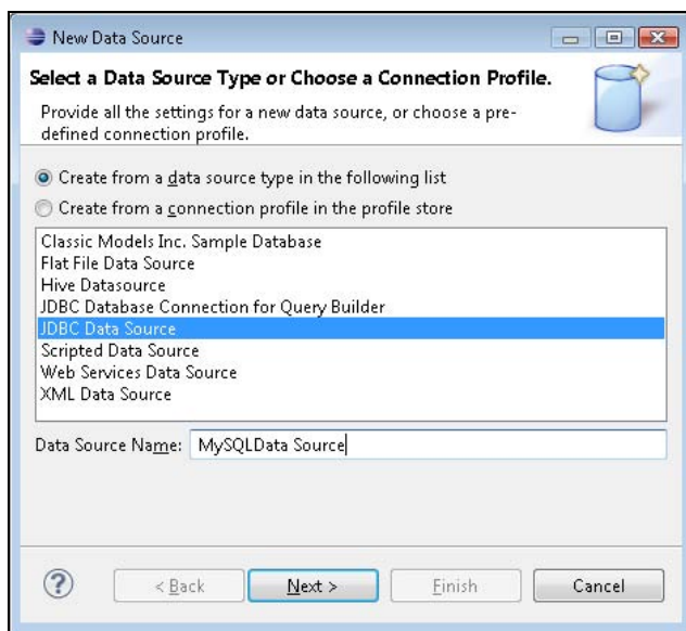
Рис. 16.4. Диалоговое окно создания источника данных BIRT-отчета
