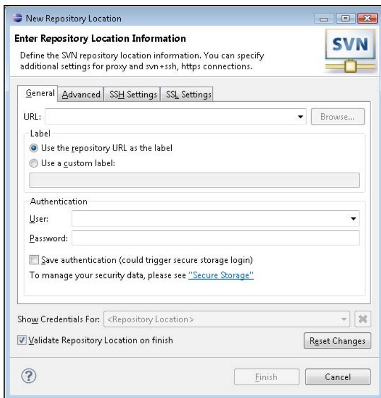
Рис. 3.31. Мастер Subversion-плагина New Repository Location создания соединения с удаленным репозиторием
