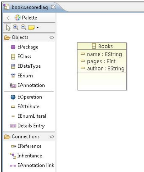
Рис. 17.11. Есоре-диаграмма метамодели списка книг
