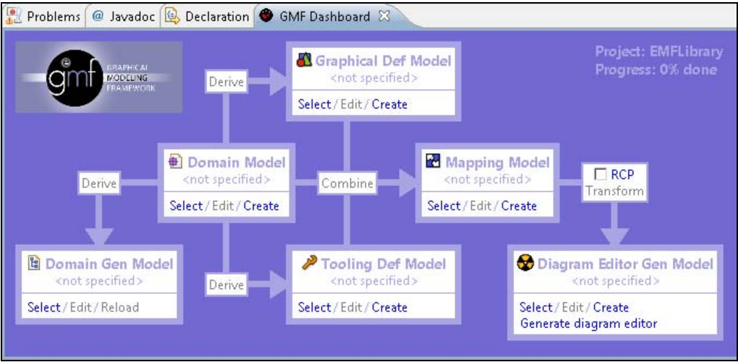
Рис. 17.7. Инструмент GMF Dashboard создания GMP-редактора
