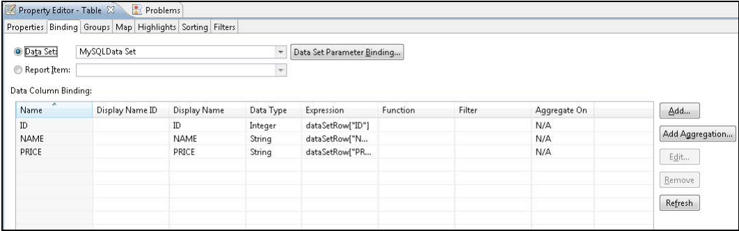
Рис. 16.10. Связывание столбцов таблицы BIRT-отчета с набором данных
