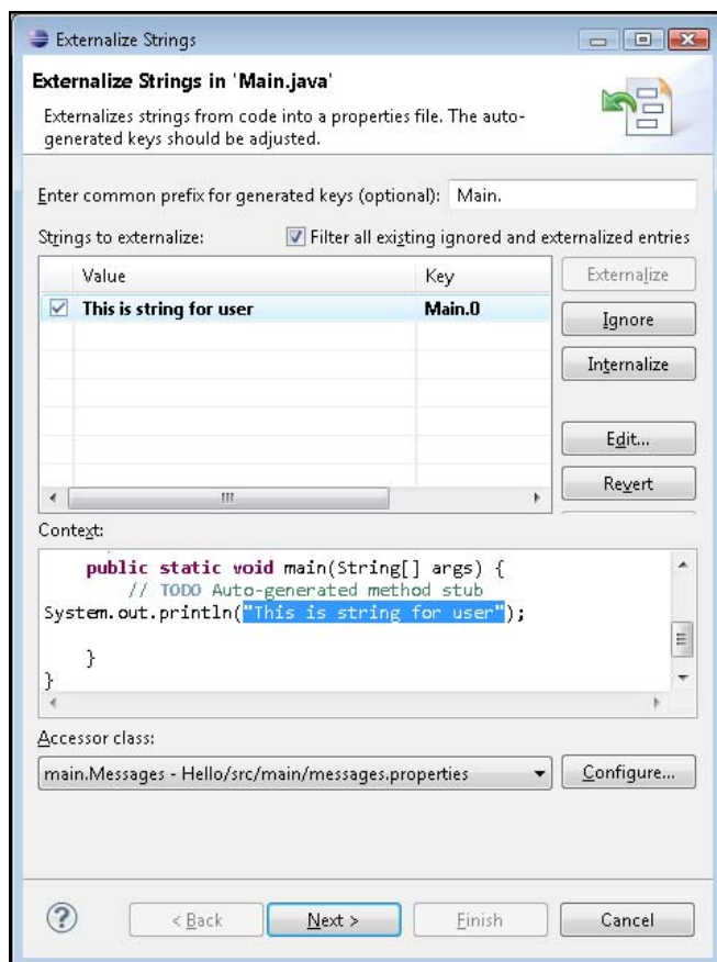
Рис. 4.3. Мастер интернационализации JDT-плагина
