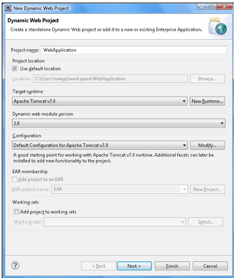
Рис. 14.2. Мастер создания проекта Dynamic Web Project
