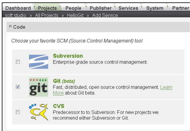
Рис. 3.39. Создание удаленного Git-репозитория
