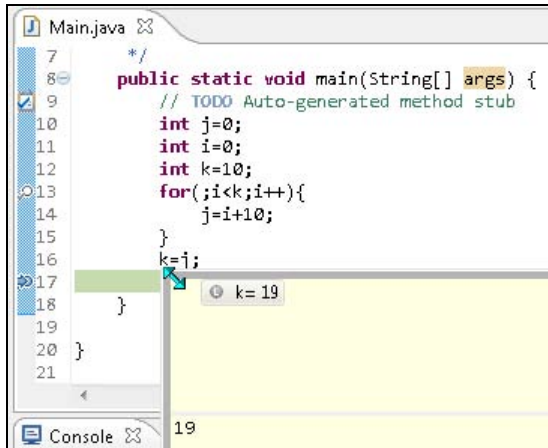
Рис. 2.9. Просмотр значения переменной в редакторе кода с помощью всплывающего окна
