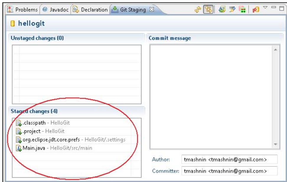
Рис. 3.35. Представление Git Staging плагина EGit, отображающее подготовленные к фиксации файлы проекта
