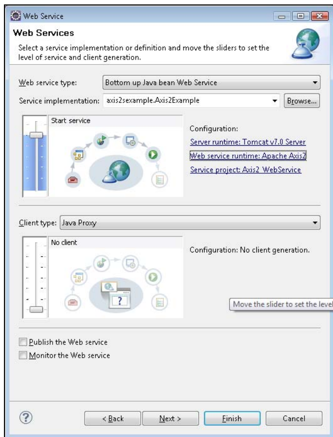
Рис. 14.14. Диалоговое окно создания Web-сервиса
