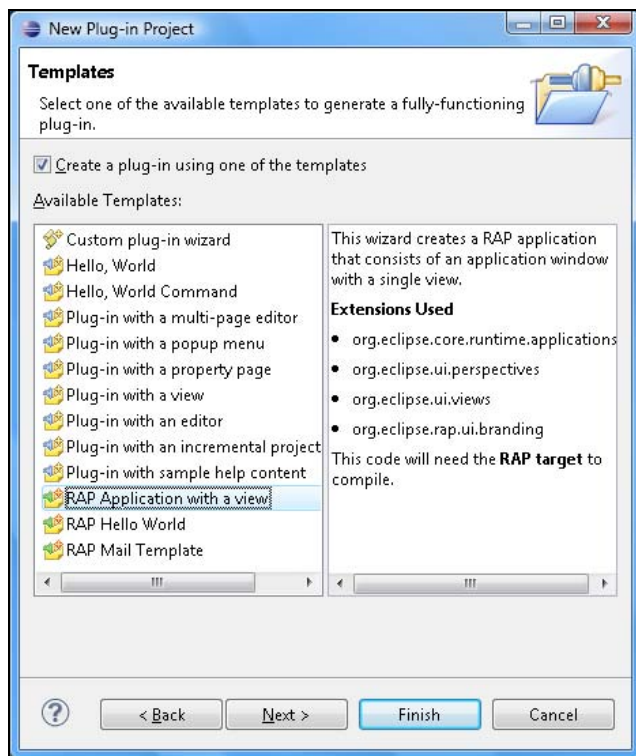
Рис. 9.3. Шаблоны RAP-приложений мастера создания проекта Eclipse-плагины
