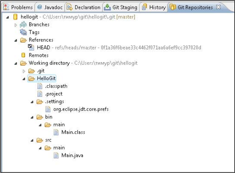
Рис. 3.37. Представление Git Repositories , отображающее структуру созданного репозитория
