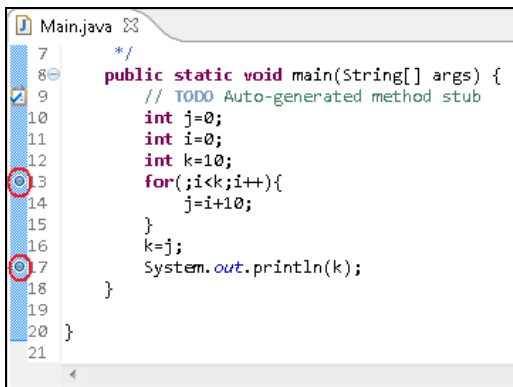
Рис. 2.3. Маркеры точек останова в окне редактора
