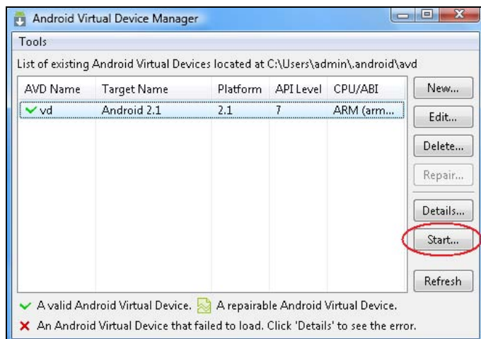
Рис. 8.18. Окно приложения AVD Manager
