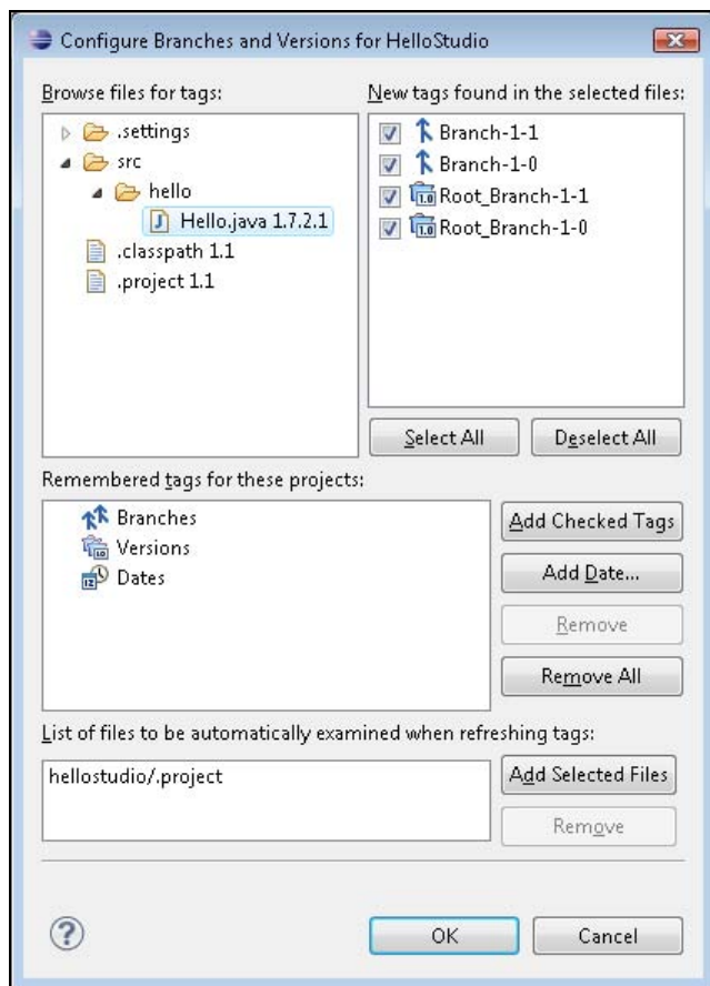
Рис. 3.16. Добавление тегов в опцию Merge
