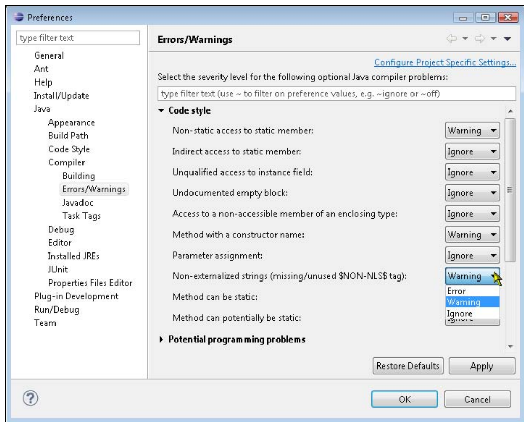
Рис. 4.1. Установка вывода предупреждений при компиляции кода для неинтернационализированных строк
