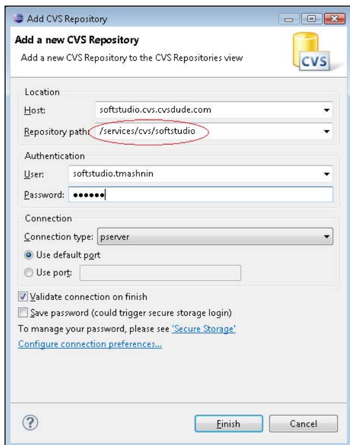
Рис. 3.8. Окно мастера создания соединения с репозиторием
