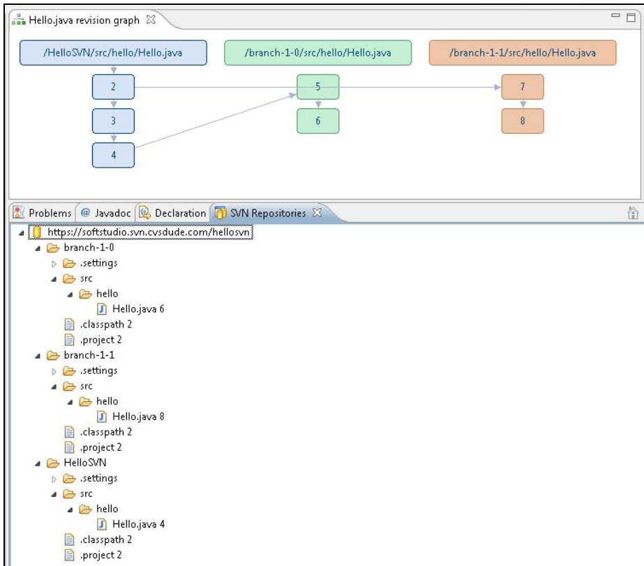
Рис. 3.25. Репозиторий, содержащий главный ствол разработки и ветки. Ревизии ресурсов веток следуют общей истории изменений репозитория. Каталог ветки branch-1-0/ имеет ревизию 6, а каталог ветки branch-1-1/ — ревизию 8
