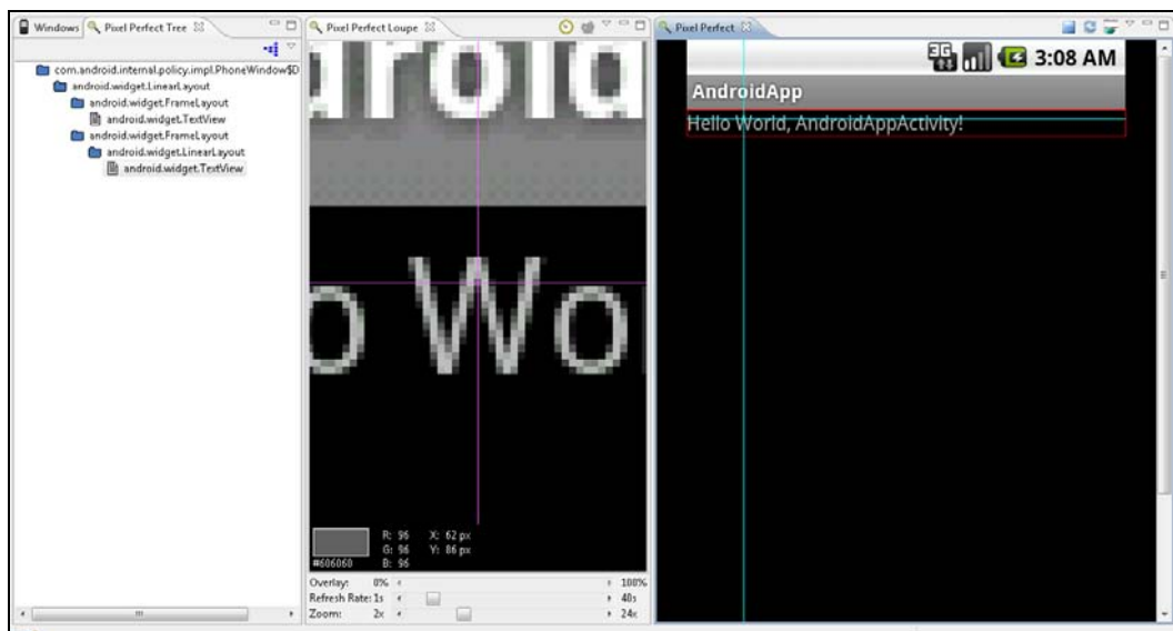
Рис. 8.11. Представления перспективы Pixel Perfect
