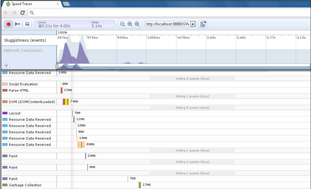
Рис. 10.8. Анализ работы GWT-приложения инструментом Speed Tracer
