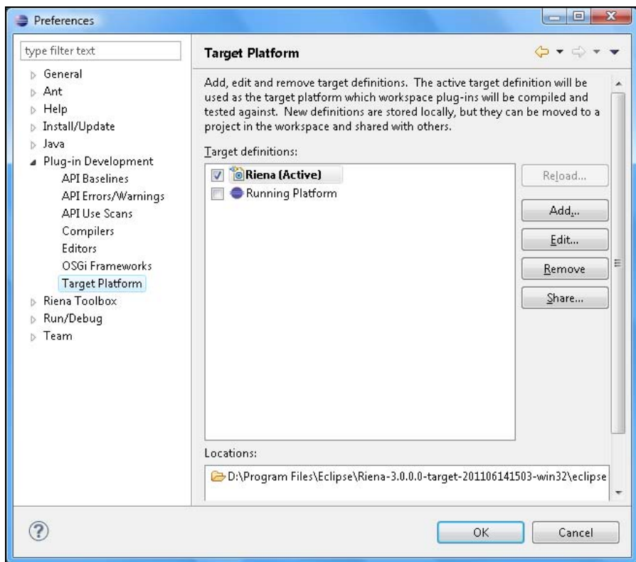
Рис. 11.1. Назначение платформы Riena в качестве целевой платформы разработки
