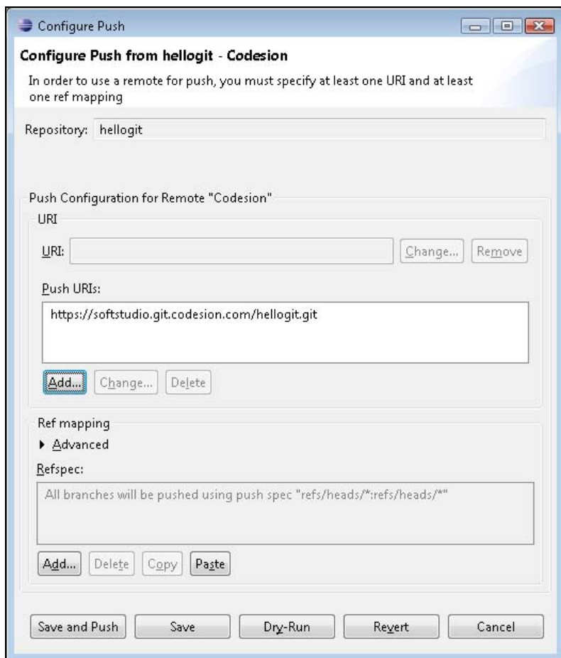
Рис. 3.40. Мастер настройки конфигурации соединения с удаленным Git-репозиторием для передачи ему изменений из локального Git-репозитория
