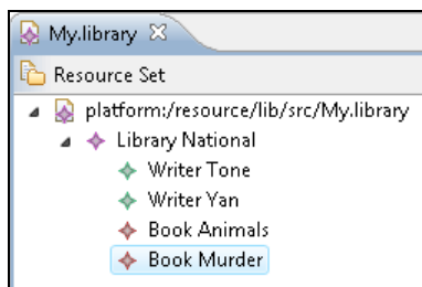
Рис. 17.12. Модель библиотеки
