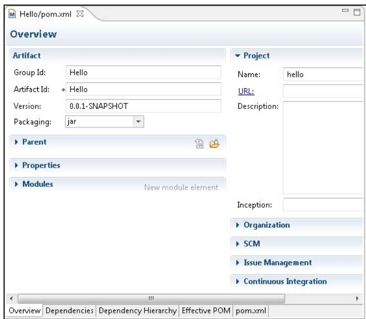
Рис. 1.36. Редактор POM-файлов
