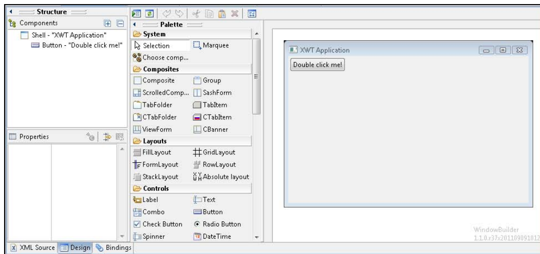
Рис. 5.7. WindowBuilder-редактор XWT-файла
