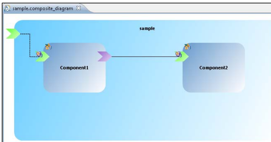
Рис. 12.5. Composite-диаграмма SCA-приложения
