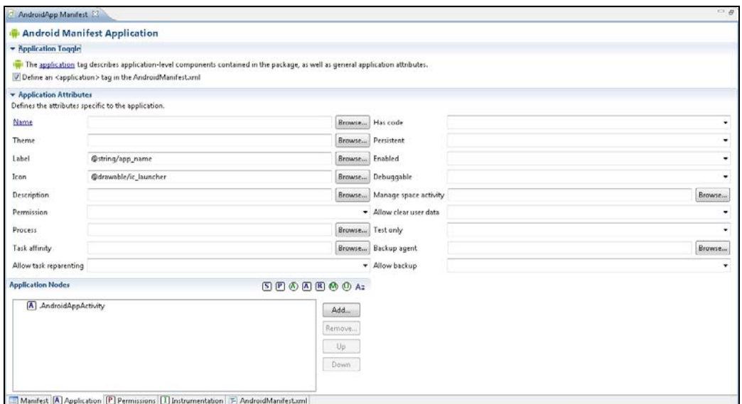
Рис. 8.25. Редактор файла AndroidManifest.xml ADT-плагина
