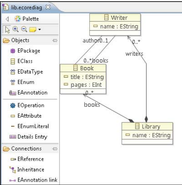
Рис. 17.6. Ecore-диаграмма простой модели данных библиотеки
