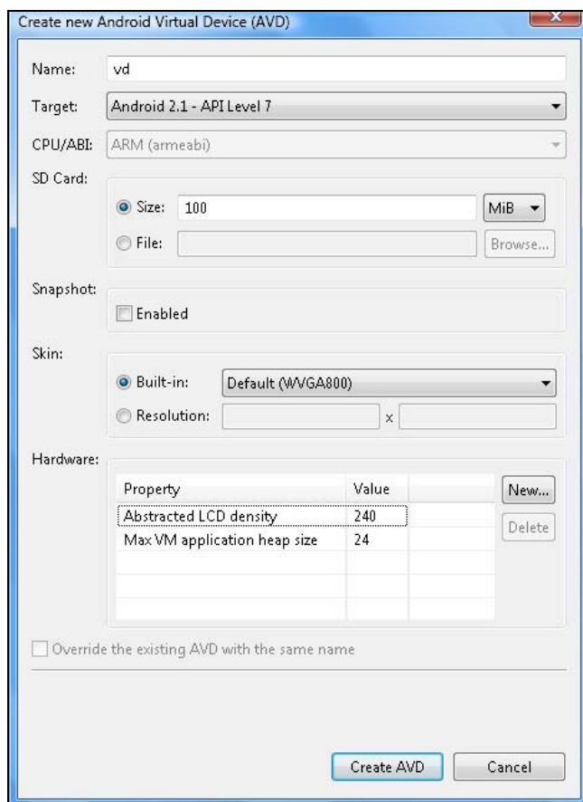
Рис. 8.17. Мастер создания виртуального Android-устройства
