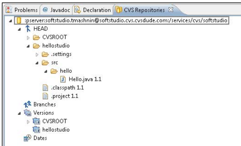
Рис. 3.12. Структура репозитория после сохранения проекта
