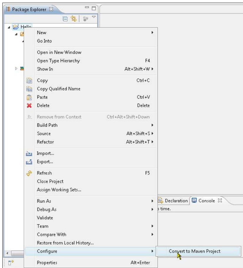
Рис. 1.34. Команда конвертации Java-проекта в Maven-проект
