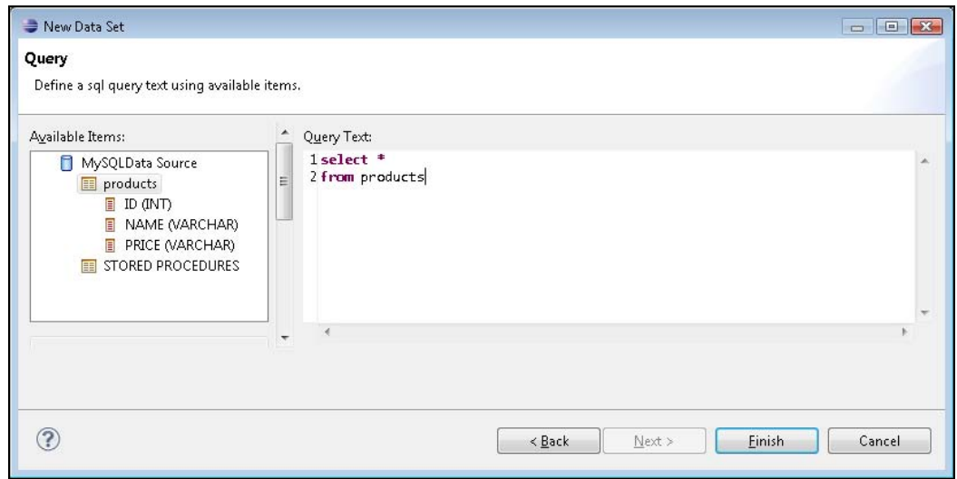
Рис. 16.6. Создание набора данных BIRT-отчета
