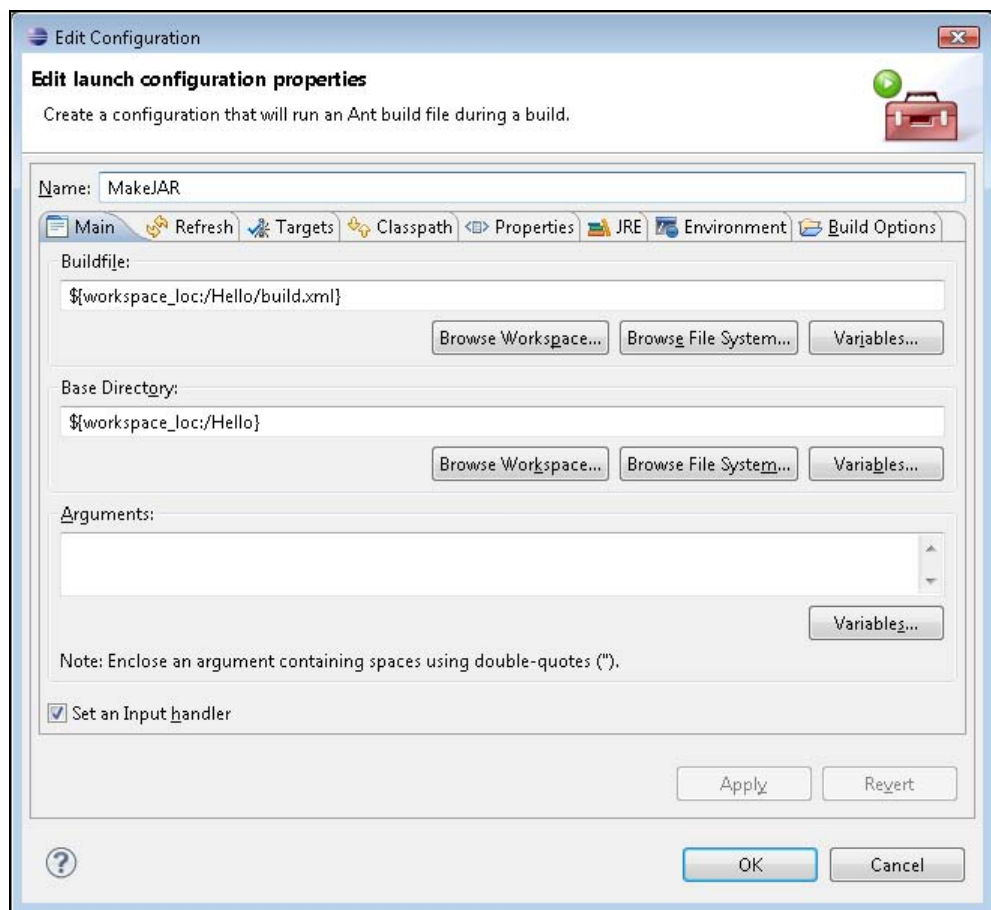
Рис. 1.27. Создание Ant-сборщика проекта
