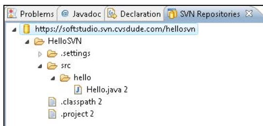
Рис. 3.21. Структура репозитория
