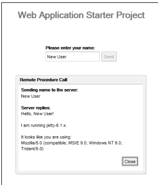
Рис. 10.5. Web-страница GWT-приложения
