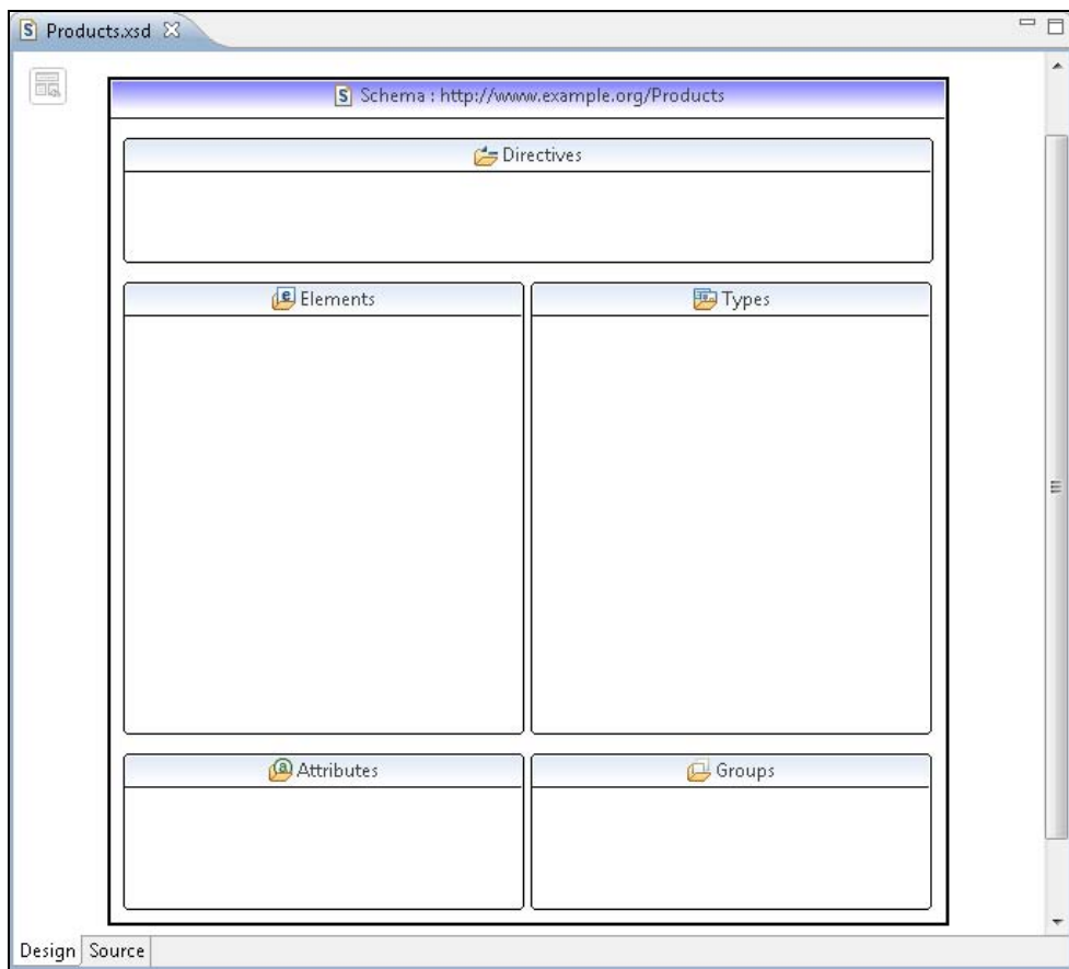
Рис. 1.40. XML-редактор XML-схемы
