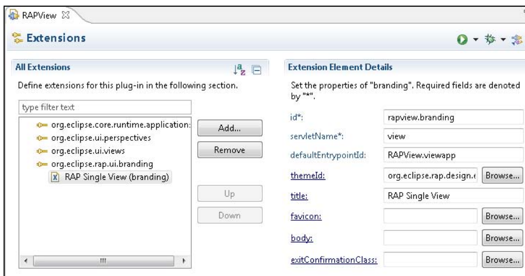
Рис. 9.6. Брендинг RAP-приложения
