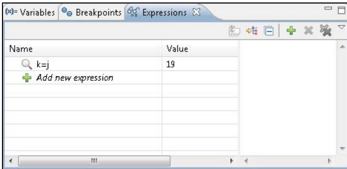
Рис. 2.11. Представление Expressions
