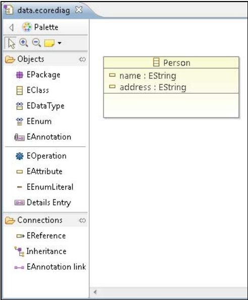
Рис. 17.1. Диаграмма Ecore-модели
