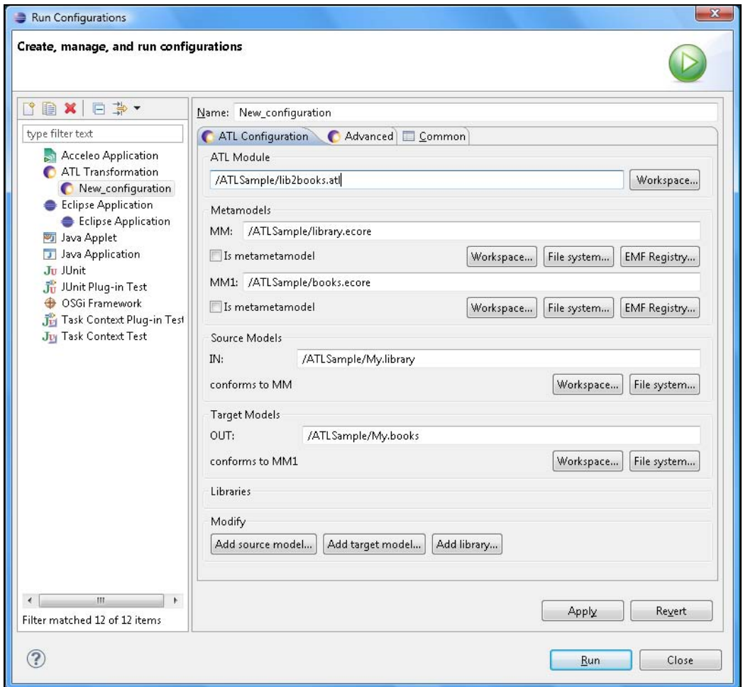
Рис. 17.14. ATL-конфигурация трансформации
