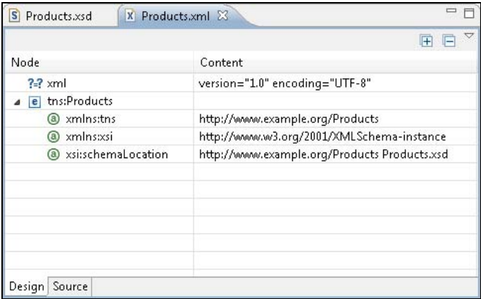
Рис. 1.42. XML-редактор XML-файлов
