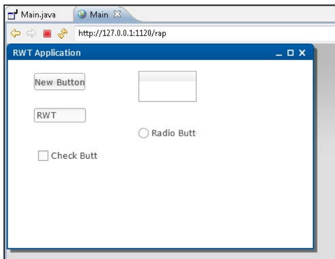
Рис. 9.8. Web-страница RWT-приложения
