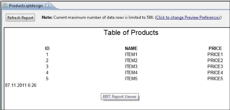
Рис. 16.11. Сформированный BIRT-отчет
