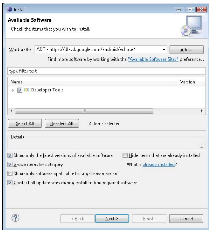
Рис. 8.1. Установка ADT-плагина
