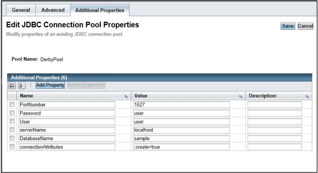
Рис. 14.13. Определение конфигурации соединения с базой данных Derby в сервере GlassFish
