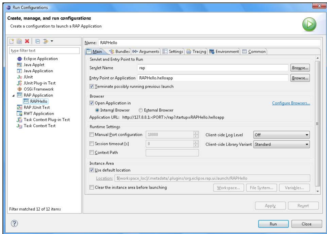
Рис. 9.4. Вкладка Main конфигурации раздела RAP Application мастера запуска приложений
