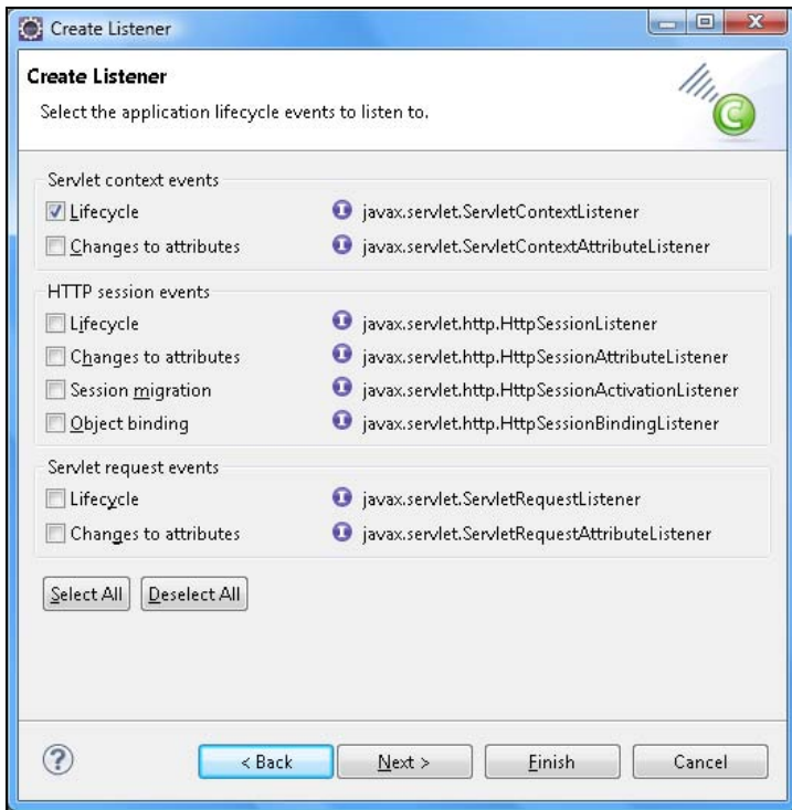
Рис. 14.11. Мастер создания слушателя Servlet-контекста
