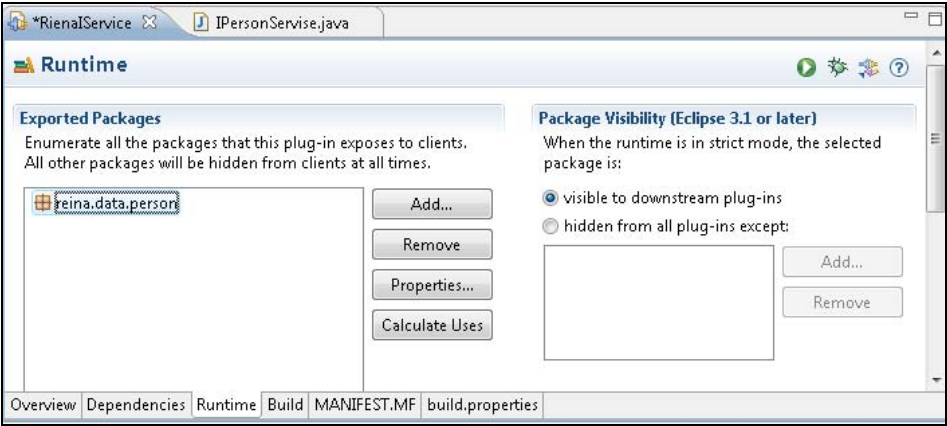
Рис. 11.6. Экспорт пакета интерфейса сервиса
