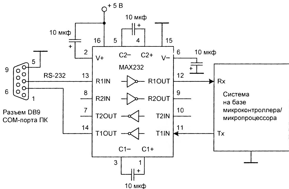
Рис. 2.5. Реализация интерфейса на базе RS-232 между двумя устройствами
