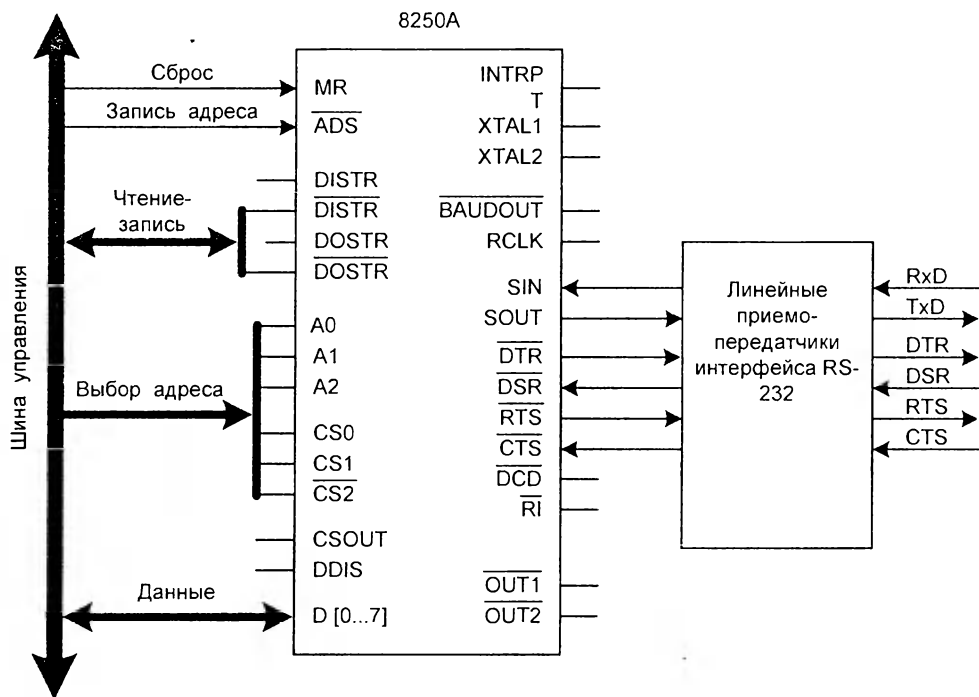
Рис. 3.1. Блок-схема подключения устройства UART 8250A
