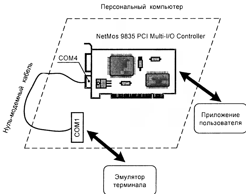
Рис. 4.2. Схема тестирования COM-портов
