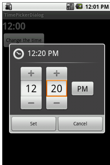
Рис. 9.9. Диалог TimePickerDialog
