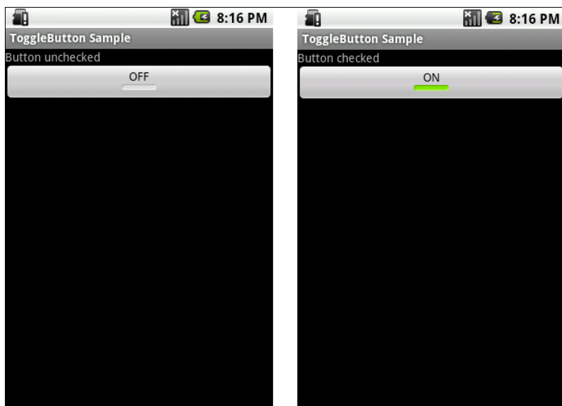
Рис. 6.12. Элемент ToggleButton
