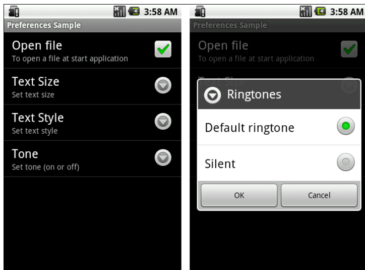
Рис. 14.8. Список RingtonePreference
