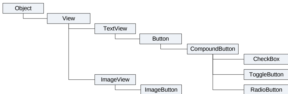
Рис. 6.7. Иерархия классов
