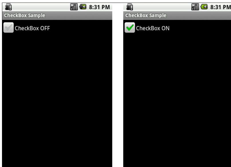
Рис. 6.11. Элемент CheckBox
