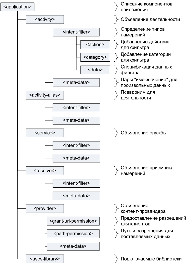
Рис. 4.4. Структура элемента <application>
