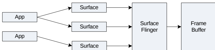
Рис. 1.2. Обработка графической информации менеджером поверхностей
