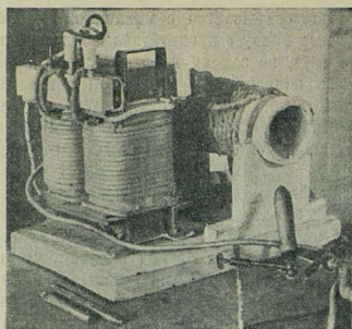
Юные техники Ивантевской средней школы Лёва Бойков и Василий Бузыкин сделали настоящий, действующий аппарат для электросварки металлических деталей.
