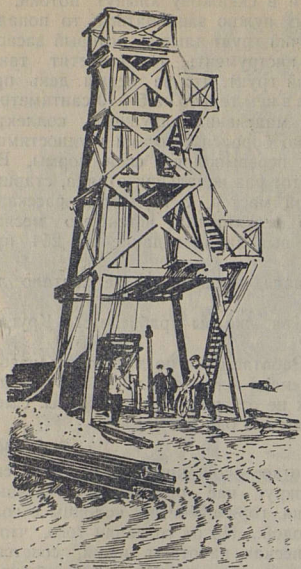
Отряд, в который мы приехали, занимался глубоким механическим бурением.
