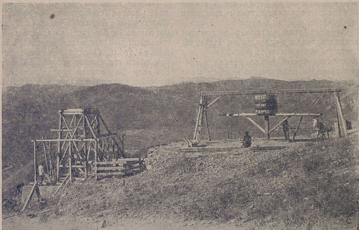
Проходка шахты.
