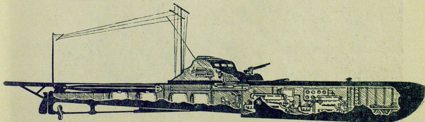
Разрез торпедного катера. В носовом отсеке лежит якорь. Затем идет машинный отсек с моторами. Над каютикой радиста устроена командирская рубка. В кормовой части бензиновые баки. Из командирской рубки идет к торпедной желобной торпедный аппарат.
