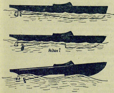
Наверху — корпус килевого катера. В середине — реданный катер в неподвижном состоянии, а внизу — на ходу.
