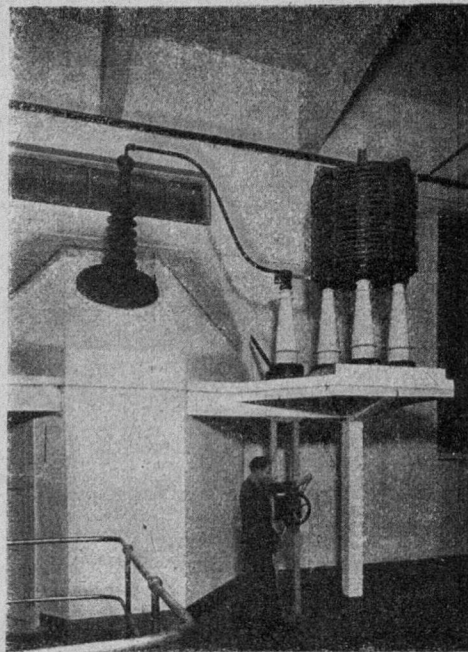
Последний предохранитель и вывод провода из башни на линию
