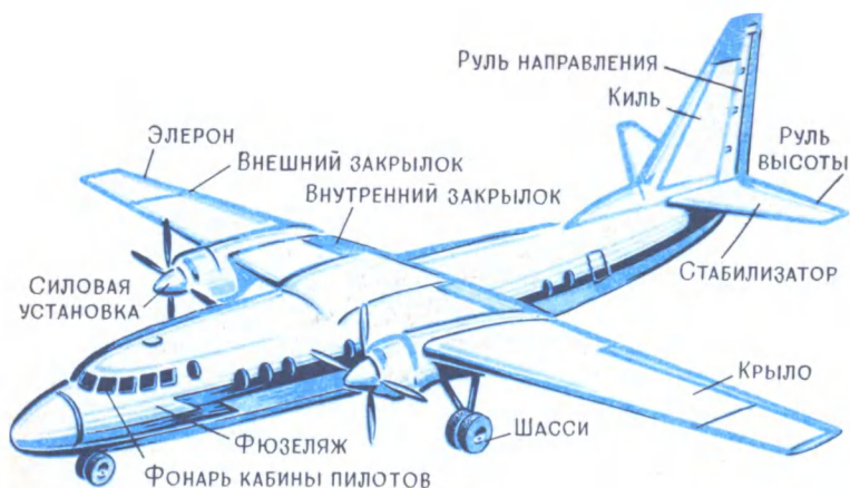
Основные части самолета
