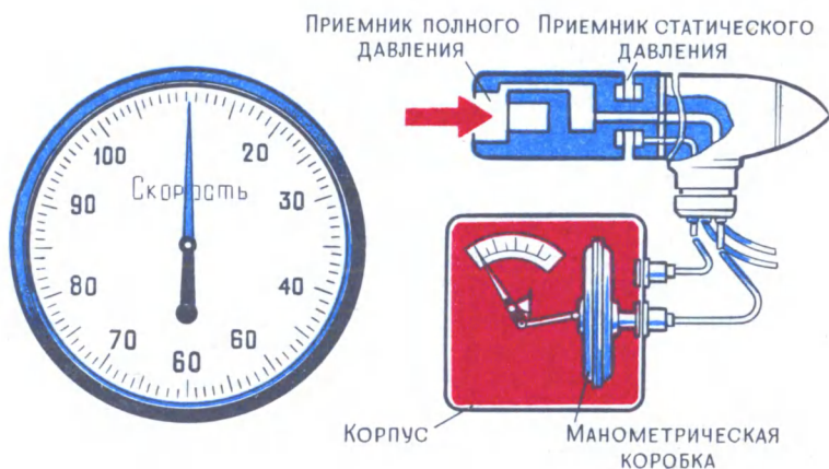
Указатель скорости
