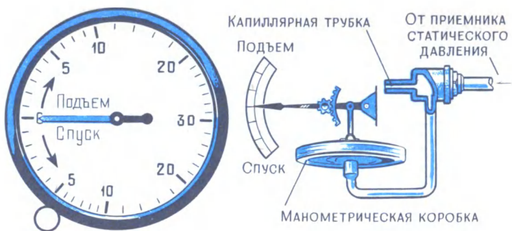
Схема вариометра
