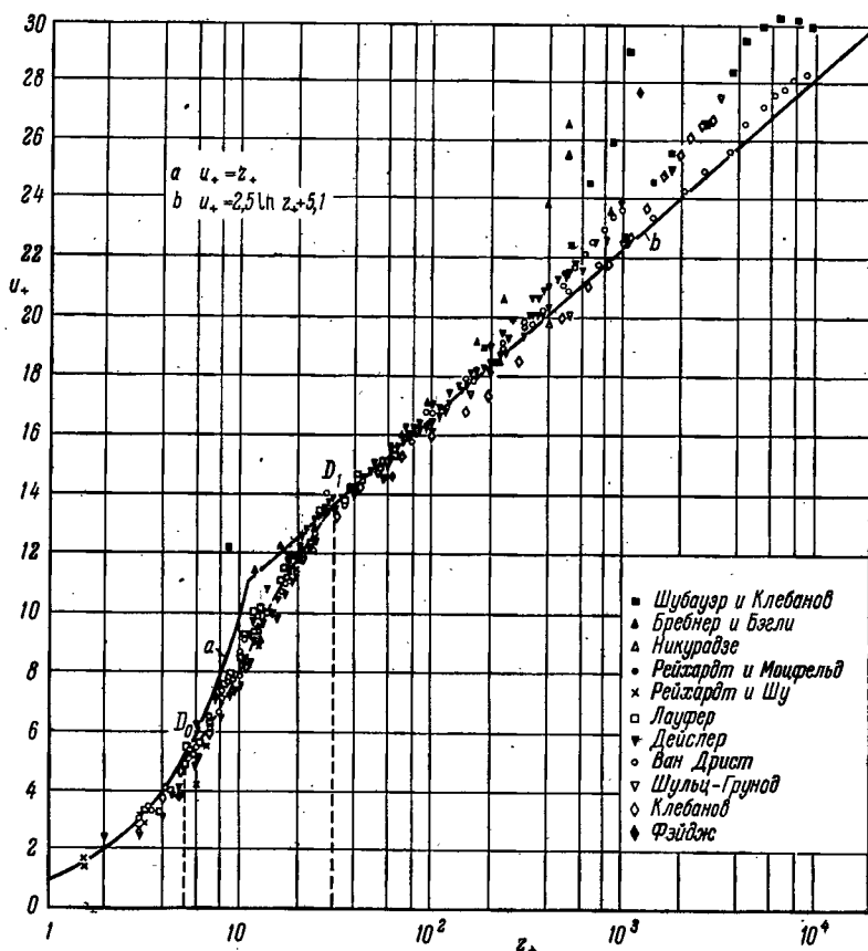
Рис. 25. Универсальный безразмерный профиль средней скорости турбулентного течения около гладкой стенки по данным измерений в трубах, каналах и пограничном слое (по Кестину и Ричардсону (1953)).
