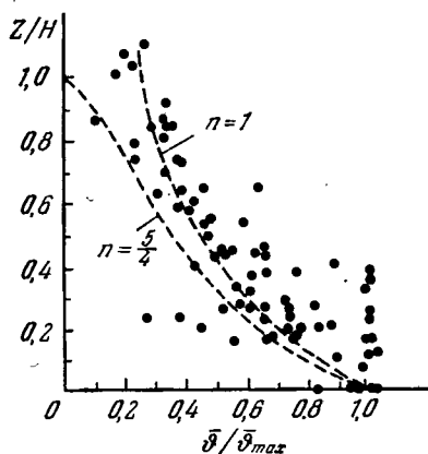
Рис. 85. Вертикальное распределение плотности дыма в дымовой струе.
