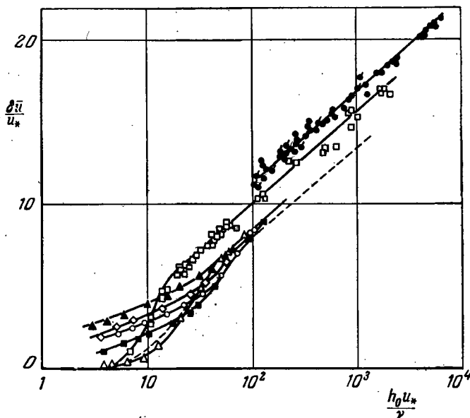
Рис. 29. Влияние шероховатости стенки на относительное уменьшение средней скорости \delta \bar{u}/u_* (по Клаузеру (1956)).
