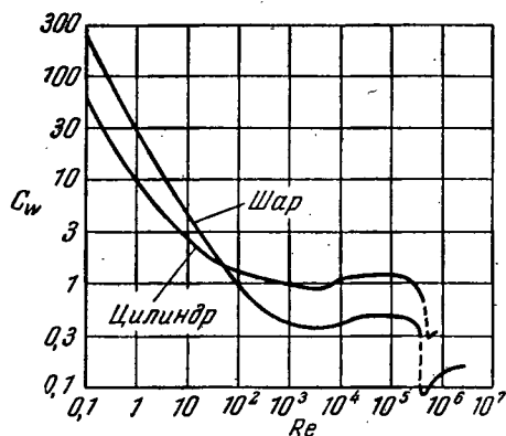
Рис. 9. Зависимость коэффициентов сопротивления шара и круглого цилиндра от числа Рейнольдса.
