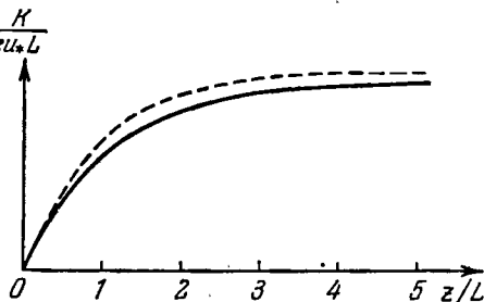
Рис. 52. Зависимость безразмерного коэффициента обмена K/\chi u_* L от безразмерной высоты \xi согласно теории Казанского и Монина (сплошная линия) и согласно эмпирической формуле Дородницына и др. (пунктир).
