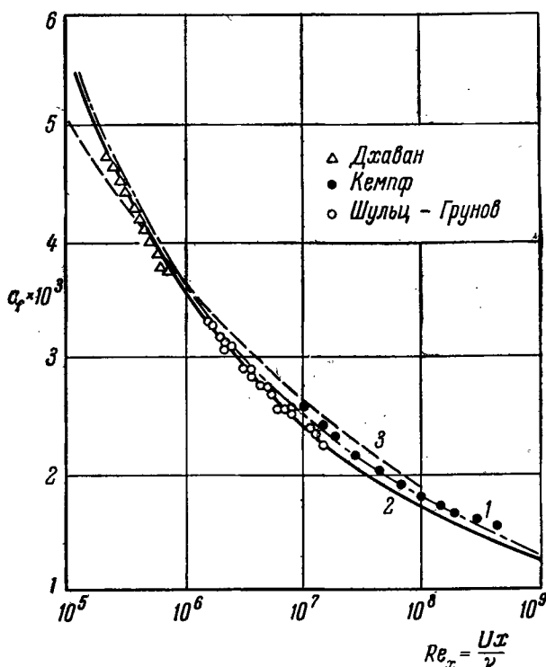
Рис. 42. Зависимость коэффициента сопротивления c_f для пограничного слоя на плоской пластинке от числа Рейнольдса Re_x по данным Кемпфа, Шульц-Грунова и Джавана.
