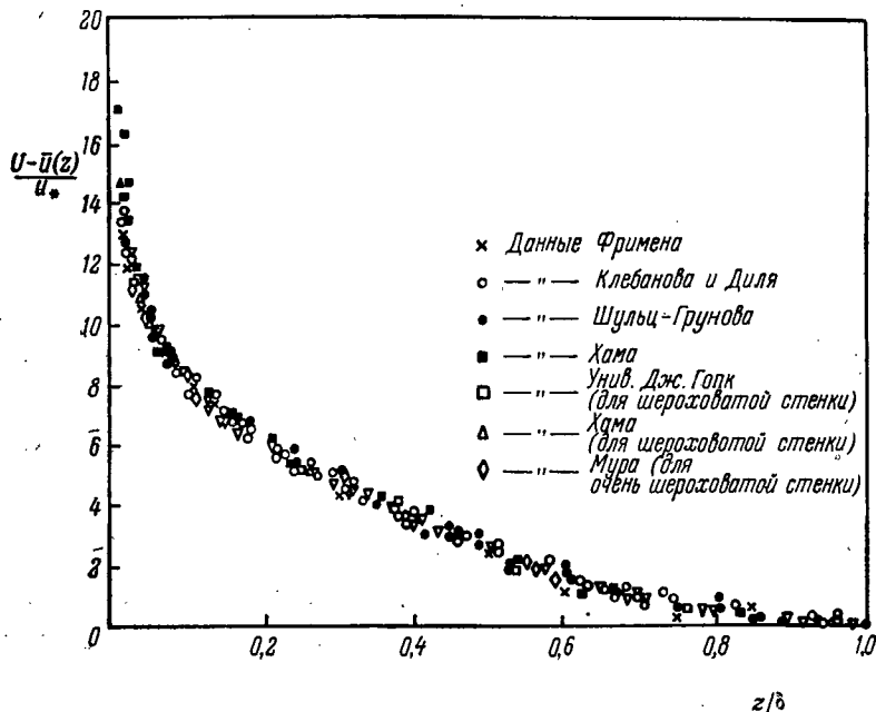
Рис. 35. Проверка закона дефекта скорости для турбулентного пограничного слоя по данным разных авторов.
