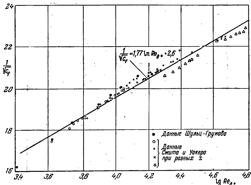
Рис. 41. Зависимость локального коэффициента сопротивления c_f для пограничного слоя на плоской пластинке от числа Рейнольдса Re_x по данным Шульц-Грунова и Смита и Уокера.
