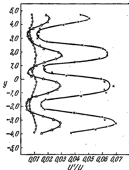
Рис. 24. Зависимость относительной величины типичной пульсации продольной скорости U' от «боковой» координаты y в пограничном слое над плоской пластинкой на различных расстояниях x от колеблющейся металлической ленты, создающей возмущения.
