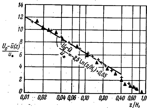
Рис. 31. Проверка закона дефекта скорости для турбулентного течения в прямоугольном канале по данным Лауфера ( \nabla ) и Дёнха (F. Döbch) (+).
