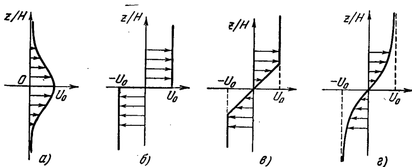
Рис. 19. Схематические формы профилей скорости для некоторых плоскопараллельных течений в безграничном пространстве.
