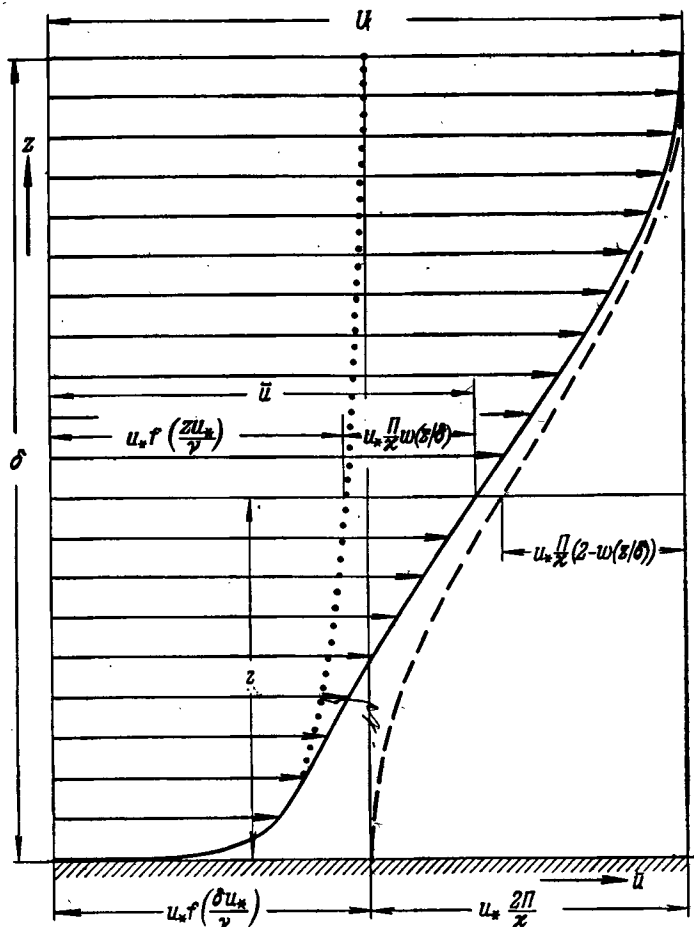
Рис. 40. Схематическое изображение профиля скорости, удовлетворяющего закону следа Коулса.
