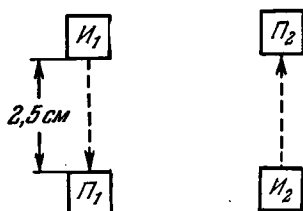
Рис. 70. Схема расположения излучателей и приемников в акустическом микроанемометре.
