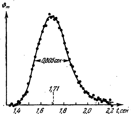
Рис. 81. Зависимость концентрации соли в фиксированном сечении прямой трубы от времени по данным Тэйлора (1954a).
