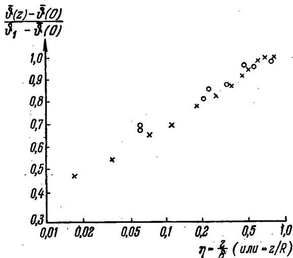
Рис. 43. Распределение средней температуры при турбулентном течении в трубе и в пограничном слое по данным Элиаса (O) и Нуннера (X).
