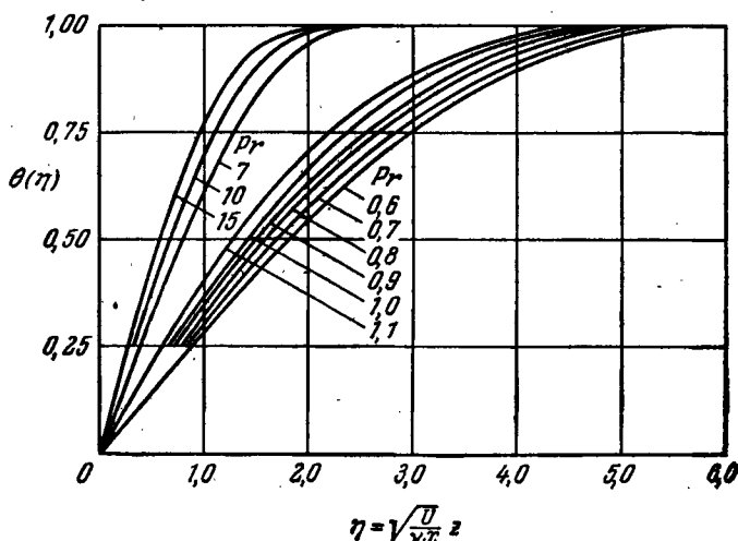
Рис. 6. Профиль температуры в пограничном слое на плоской пластинке при различных числах Прандтля.
