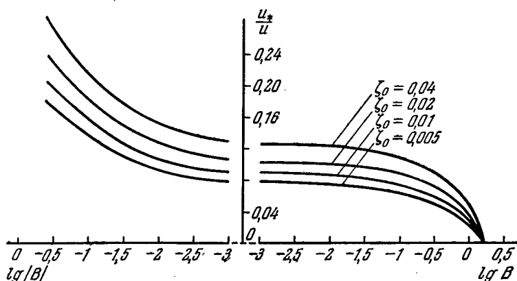
Рис. 73. Номограмма Казанского и Монины для определения безразмерного напряжения трения u_*/U = F_1 по параметру стратификации B и параметру шероховатости \zeta_0 .
