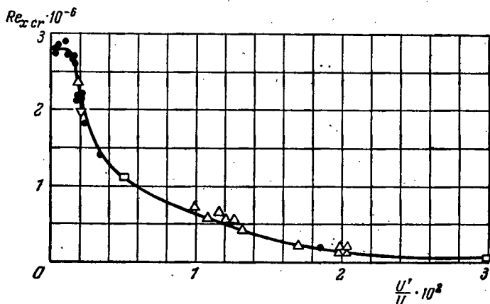
Рис. 7. Зависимость критического числа Рейнольдса для пограничного слоя на плоской пластинке от степеней возмущенности набегающего потока (по Драйдену (1959)).
