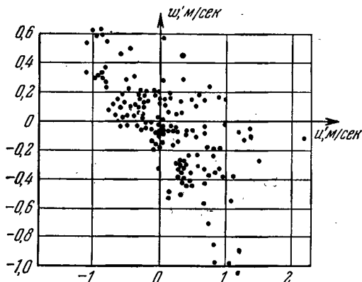
Рис. 72. Пример корреляционного графика для пульсаций горизонтальной и вертикальной компонент скорости ветра.
