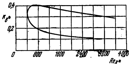
Рис. 15. Форма нейтральной кривой на плоскости (k, Re_{s*}) для пограничного слоя над плоской пластинкой.
