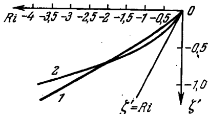
Рис. 59. Эмпирическая зависимость \zeta' = \zeta/\alpha от числа Ричардсона Ri при Ri < 0 , полученная в результате осреднения данных Пановского, Блэкедара и Маквейла (1960) и Уэбба (1960) (кривая 1) и по данным Гурвича (1962) (кривая 2).
