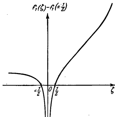
Рис. 50. Схематический вид универсальной функции
