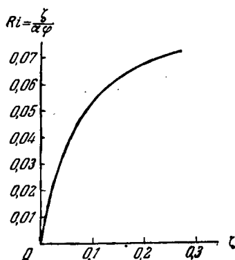
Рис. 60. Эмпирическая зависимость Ri от \zeta при устойчивой стратификации по данным Гурвича (1965).
