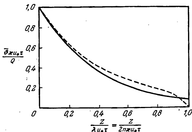
Рис. 86. Сопоставление вертикального распределения концентрации по теории диффузии с конечной скоростью (пунктирная кривая) с распределением, получаемым из параболического уравнения диффузии с линейным по высоте коэффициентом обмена (сплошная кривая).
