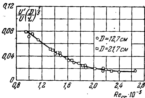
Рис. 10. Зависимость Re_{cr} при обтекании шара от величины \frac{U'}{U} \left( \frac{D}{L} \right)^{1/2} .
