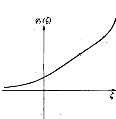
Рис. 49. Схематический вид универсальной функции \varphi_1(\zeta) .
