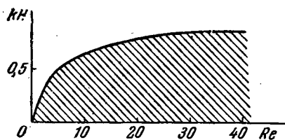
Рис. 21. Расположение нейтральной кривой и области неустойчивости (на рисунке заштрихована) на плоскости (k, Re) для зоны смещения двух плоскопараллельных потоков по данным Бетчова и Шевчика (1963).
