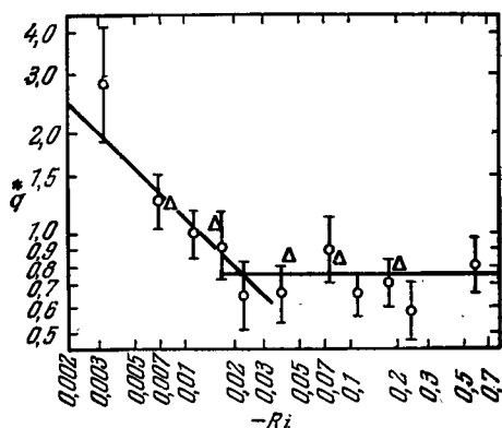
Рис. 68. Зависимость \dot{q} от Ri по данным Суинбенка и Тэйлора (O) и Перепелкиной (Δ).
