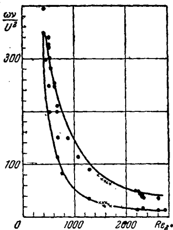
Рис. 16. Рассчитанная форма нейтральной кривой на плоскости (\omega, \text{Re}_{\delta^*}) для пограничного слоя на плоской пластинке и экспериментальные данные о частотах нейтральных колебаний.
