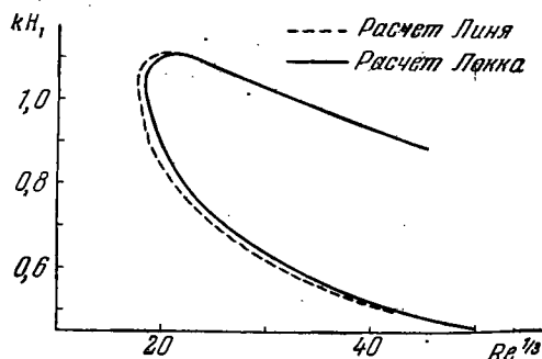
Рис. 14. Форма нейтральной кривой на плоскости (k, Re) для плоского течения Пуазейля по расчетам Линя (1945) и Локка (1955).
