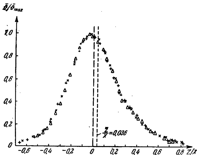
Рис. 82. Распределение температуры в нескольких сечениях двумерной турбулентной струи, в которую помещена нагретая проволочка (по Хинце и Ван дер Хегге Цийнеу).
