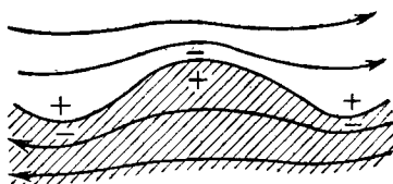
Рис. 12. Схематическая форма линий тока и распределения давления вблизи возмущенной поверхности тангенциального разрыва скорости.
