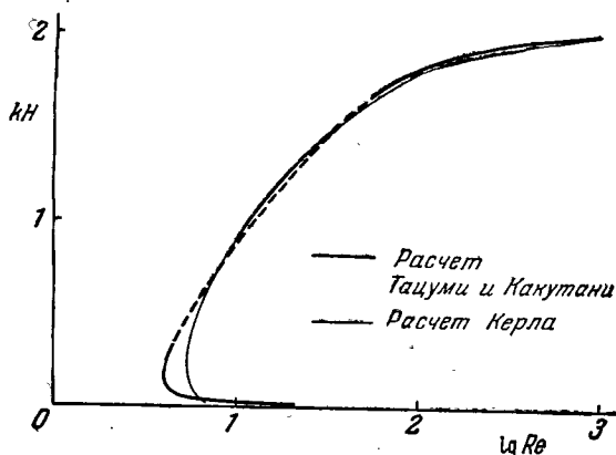
Рис. 20. Форма нейтральной кривой на плоскости (k, Re) для плоской струи по расчетам Керла (1956) и Тацуми и Какутани (1958).
