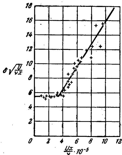
Рис. 4. Зависимость толщины пограничного слоя \delta на плоской пластинке от расстояния x от передней кромки пластинки (по данным Ханзена (1928)).
