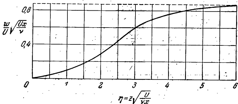
Рис. 3. Профиль вертикальной скорости в пограничном слое на плоской пластинке.
