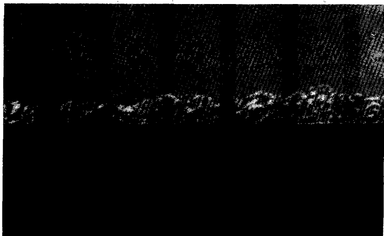
Рис. 37. Теневая фотография турбулентного пограничного слоя на цилиндре (из статей Ротта (1962а, б)). Направление течения — слева направо.
