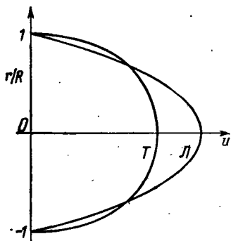
Рис. 32. Сравнение профилей средней скорости при ламинарном (Л) и турбулентном (Т) течениях в трубе.
