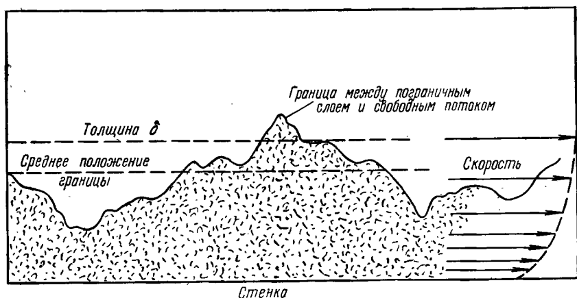
Рис. 38. Общая схема турбулентного пограничного слоя на плоской пластинке.
