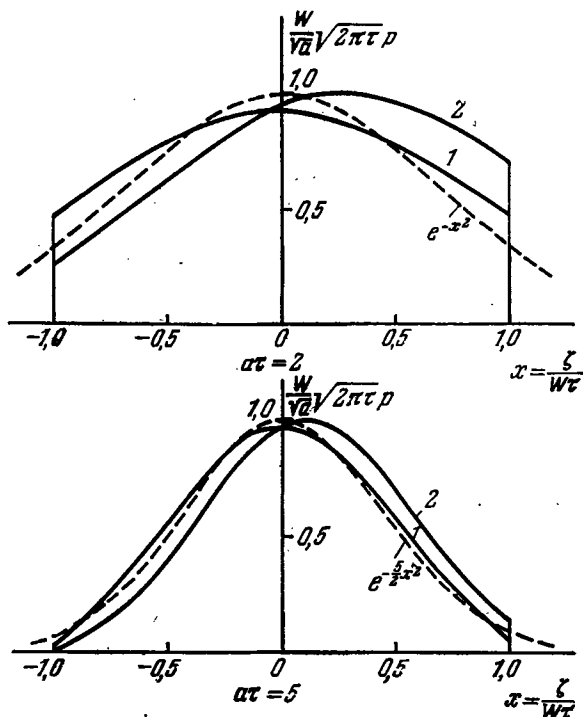
Рис. 84. Сопоставление непрерывной части распределения p(Z|z, t) при a\tau = 2 и a\tau = 5 по теории диффузии с конечной скоростью с распределением Гаусса, вытекающим из параболического уравнения диффузии.
