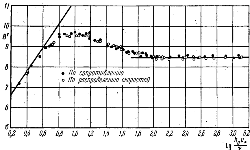
Рис. 28. Зависимость коэффициента B' от \frac{h_0 u_*}{\nu} по данным Никурадзе (1933).
