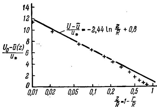
Рис. 30. Проверка закона дефекта скорости для турбулентного течения в трубе по данным Лауфера (1954).
