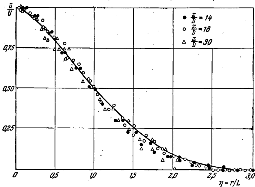
Рис. 44. Зависимость нормированной средней скорости \bar{u}/U от \eta = r/L в трех разных сечениях осесимметричной струи по данным Рейхардта (1942).
