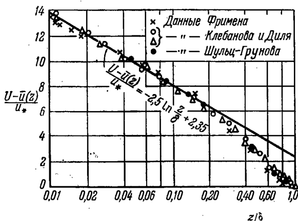
Рис. 36. Логарифмическая форма закона дефекта скорости для пограничного слоя.
