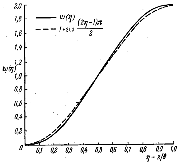
Рис. 39. Универсальная функция следа w(\eta) по Коулсу (1956).
