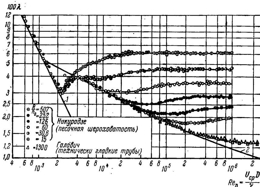
Рис. 34. Зависимость коэффициента сопротивления \lambda от числа Рейнольдса Re_D для шероховатых труб различной шероховатости.
