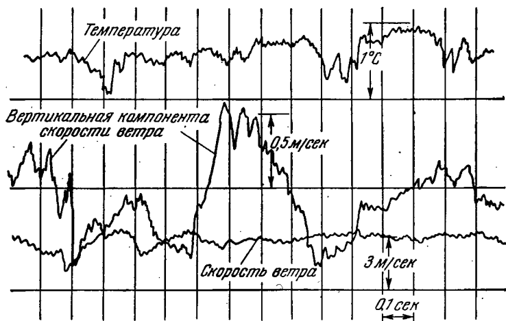
Рис. 1. Типичный пример записи пульсаций температуры, скорости ветра и вертикальной компоненты скорости ветра.
