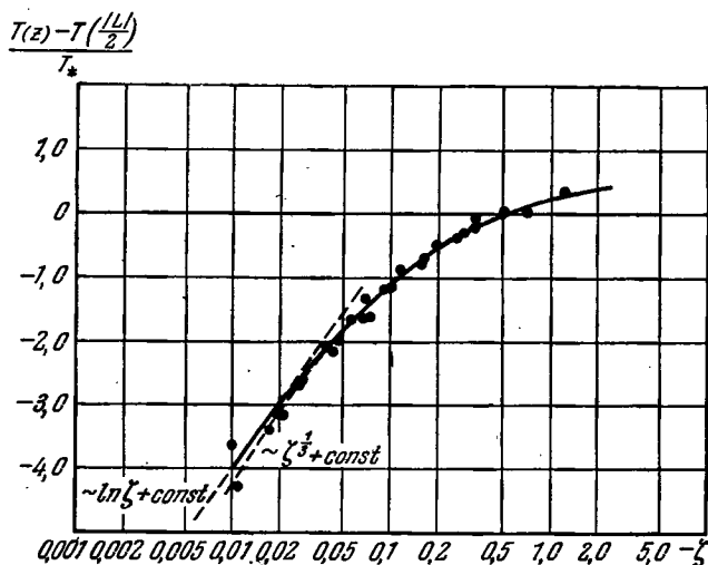
Рис. 64. Эмпирический график функции f_1(\zeta) = f_1\left(-\frac{1}{2}\right) при \zeta < 0 по данным Гурвича (1965).
