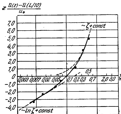
Рис. 56. Эмпирический график функции f(\zeta) - f\left(\frac{1}{10}\right) при \zeta > 0 по данным Гурвича (1965).
