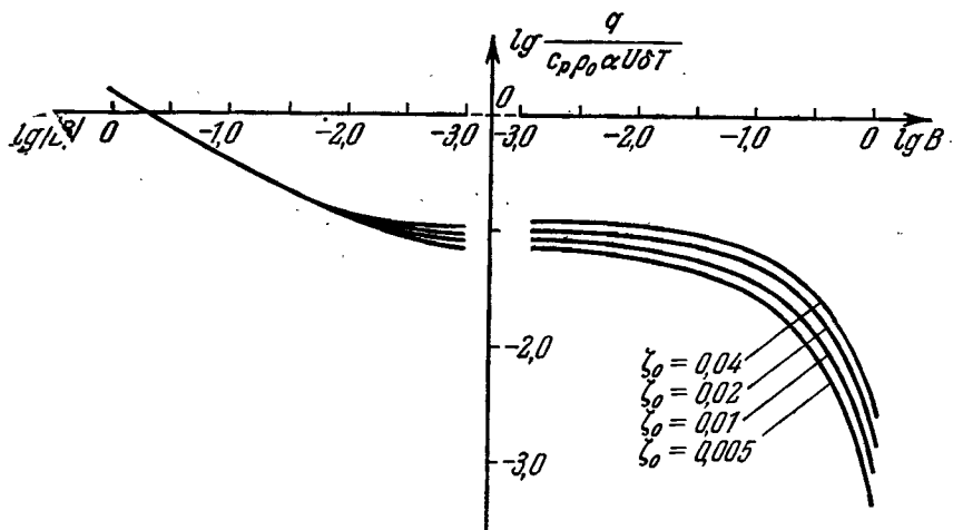
Рис. 74. Номограмма для определения безразмерного потока тепла q/c_p \rho_0 \alpha U \delta T = F_2 по B и \zeta_0 .
