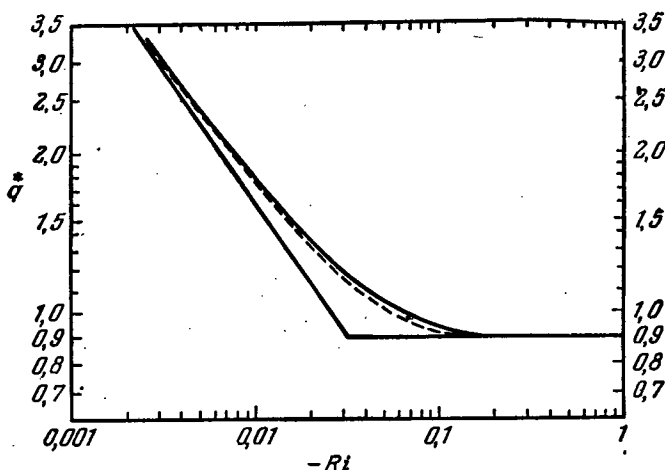
Рис. 51. Зависимость безразмерного потока тепла \dot{q} от числа Ричардсона Ri .
