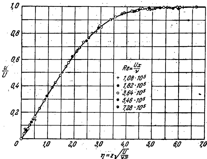
Рис. 2. Профиль продольной скорости в пограничном слое на плоской пластинке.
