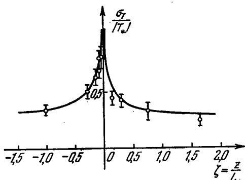
Рис. 77. Эмпирический график функции \sigma_T/|T_*| = f_6(\zeta) .
