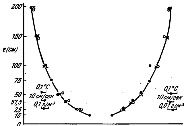
Рис. 63. Эмпирические профили скорости ветра (○), температуры (×) и влажности (●) в приземном слое при двух термических стратификациях.
