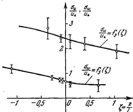
Рис. 76. Эмпирический график функций \sigma_u/u_* = f_3(\zeta) и \sigma_w/u_* = f_5(\zeta) .
