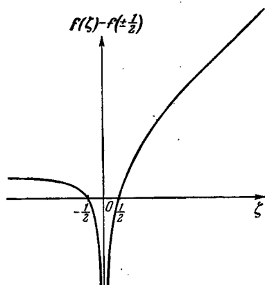
Рис. 48. Схематический вид универсальной функции
