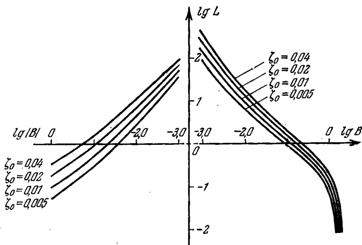
Рис. 75. Номограмма для определения L/H = F_3 по B и \zeta_0 .
