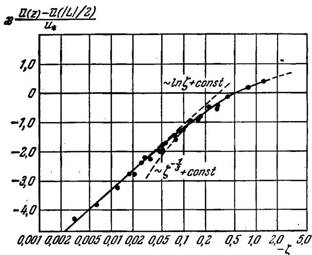
Рис. 55. Эмпирический график функции f(\zeta) = f\left(-\frac{1}{2}\right) при \zeta < 0 по данным Гурвича (1965).
