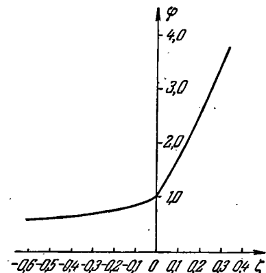
Рис. 58. Эмпирический график универсальной функции \varphi(\zeta) по данным Гурвича.
