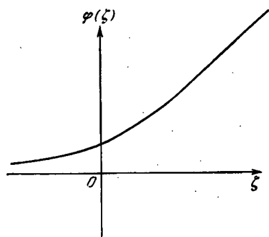
Рис. 47. Схематический вид универсальной функции \varphi(\zeta) .
