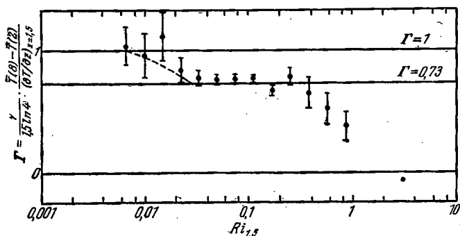
Рис. 67. Зависимость величины \Gamma от Ri при неустойчивой стратификации по эмпирическим данным.
