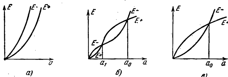
Рис. 11. Различные варианты зависимости получаемой и теряемой осциллятором энергии от амплитуды колебаний.
