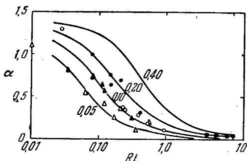
Рис. 69. Сравнение эмпирических данных Дж. Тэйлора и Эллисона и Тэрнера о зависимости \alpha от Ri с формулой Эллисона (8.14).
