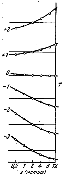
Рис. 62. Эмпирические профили средней температуры в приземном слое при различной стратификации.
