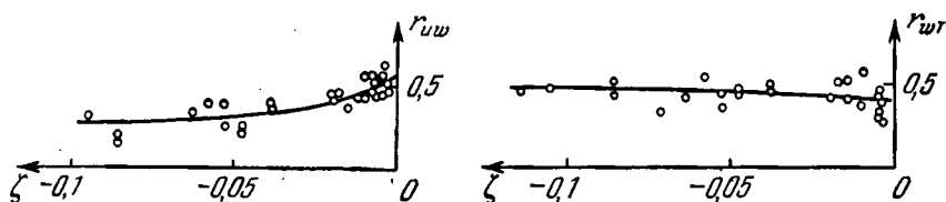
Рис. 79. Зависимость коэффициентов корреляции r_{uw} и r_{wT} от \zeta при \zeta < 0 по эмпирическим данным.
