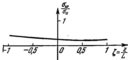
Рис. 78. Зависимость коэффициента анизотропии \sigma_w/\sigma_u от \zeta по эмпирическим данным.
