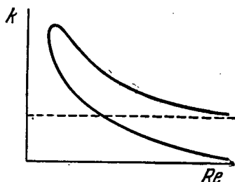
Рис. 18. Схематическая форма нейтральной кривой в плоскости (k, Re) для течения с профилем скорости, имеющим точку перегиба (например, для пограничного слоя при наличии замедляющего градиента давления).
