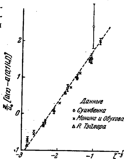
Рис. 61. Проверка «закона 1/3 » для профиля ветра при сильно неустойчивой стратификации (по Тэйлору (19606)).
