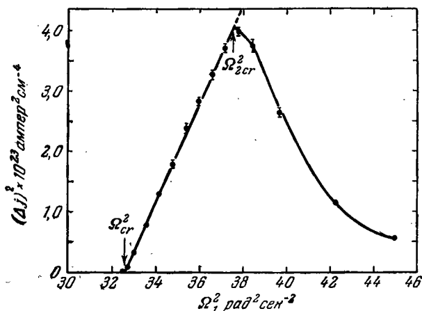
Рис. 23. Зависимость квадрата амплитуды добавочного тока (\Delta j)^2 в электролите между вращающимися цилиндрами от угловой скорости внутреннего цилиндра (по Доннелли (1963)).
