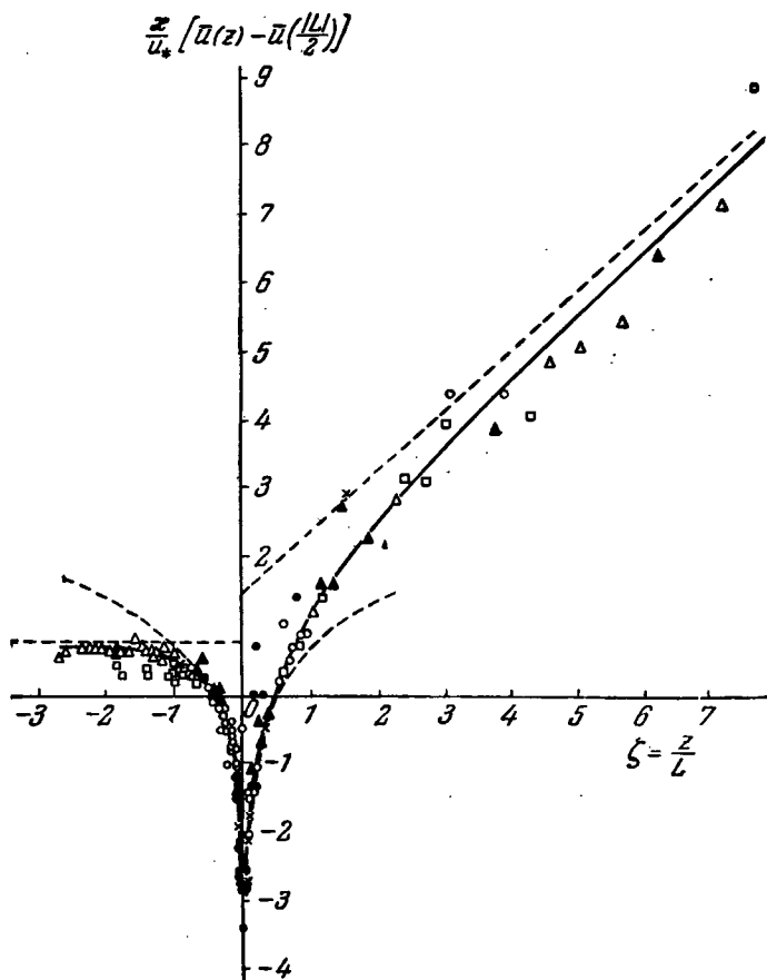
Рис. 54. Эмпирический график функции f(\zeta) - f\left(\pm \frac{1}{2}\right) по Мониному и Обухову (1953, 1954).
