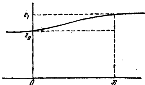
Рис. 5. Схематический вид линии тока в пограничном слое на плоской пластинке.
