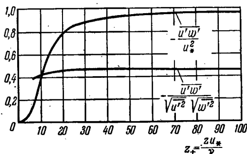
Рис. 27. Универсальные функции f_4(z_+) и f_5(z_+) по данным измерений Лауфера.
