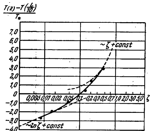
Рис. 65. Эмпирический график функции f_1(\zeta) - f_1(0, 1) при \zeta > 0 по данным Гурвича (1965).
