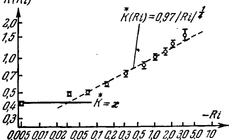
Рис. 57. Эмпирический график функции \dot{K}(Ri) по Гурвичу (1962).
