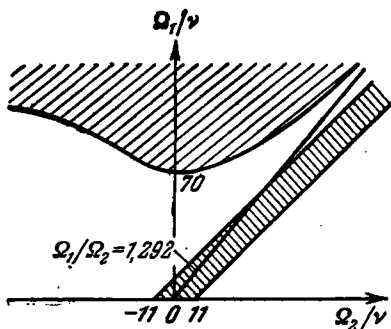
Рис. 22. Расположение области неустойчивости относительно бесконечно малых возмущений и области устойчивости относительно любых конечных возмущений для изученного Тэйлором течения Куэтта между цилиндрами.
