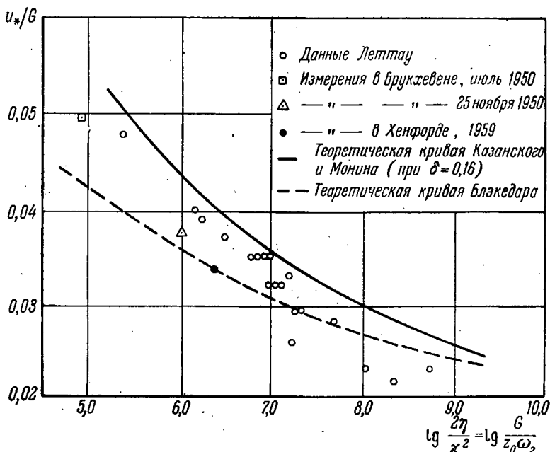
Рис. 46. Зависимость u_*/G от \eta = \frac{x^2 G}{2 z_0 \omega_z} по эмпирическим данным и по теориям Казанского и Моинна (1961) и Блэкедара (1962).
