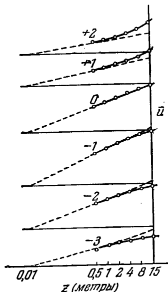
Рис. 53. Эмпирические профили средней скорости ветра в приземном слое при различных термических стратификациях.
