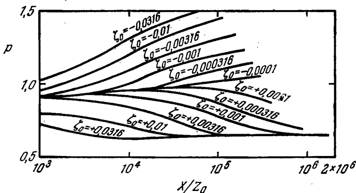
Рис. 83. Зависимость показателя p в законе убывания наземной концентрации примеси от расстояния от источника и от параметра устойчивости.
