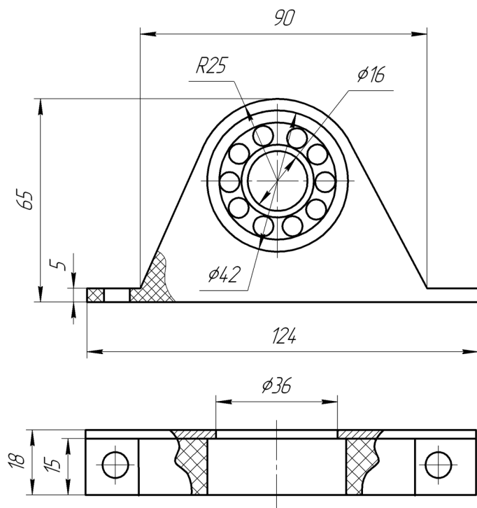
Рис.4. Опорная стойка.
