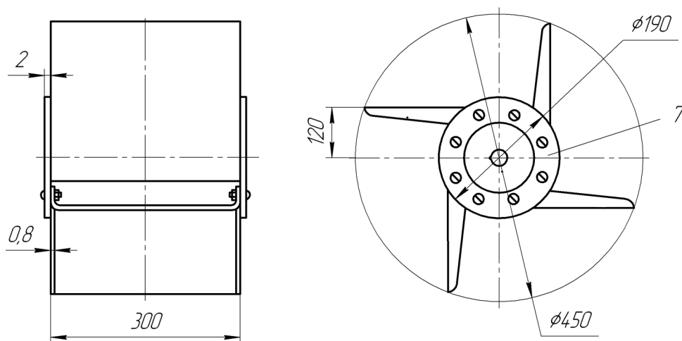
Рис. 3. Гребное колесо.
