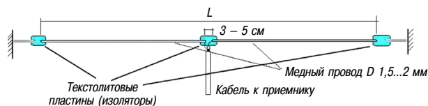
Полуволновой симметричный вибратор
