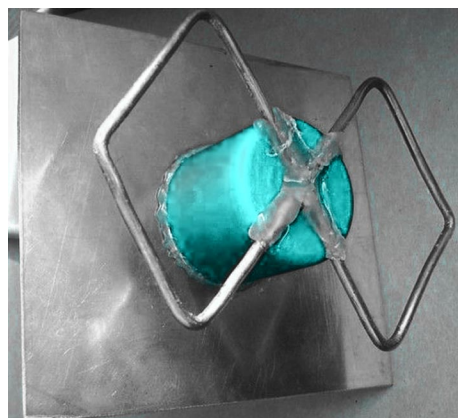
Wi-Fi-антенна
