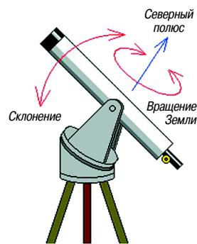
Экваториальная монтажка
