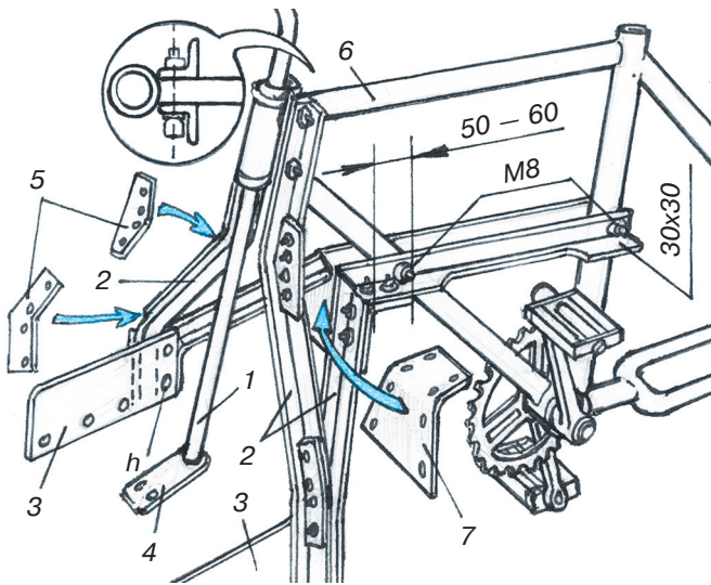
Рис. 2. Доработка рамы и рулевой колонки:
