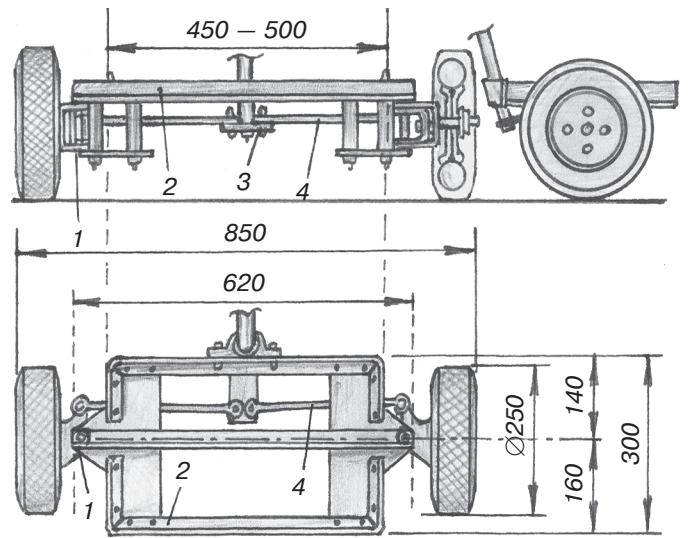
Рис. 3. Общий вид переднего моста и грузовой платформы:
