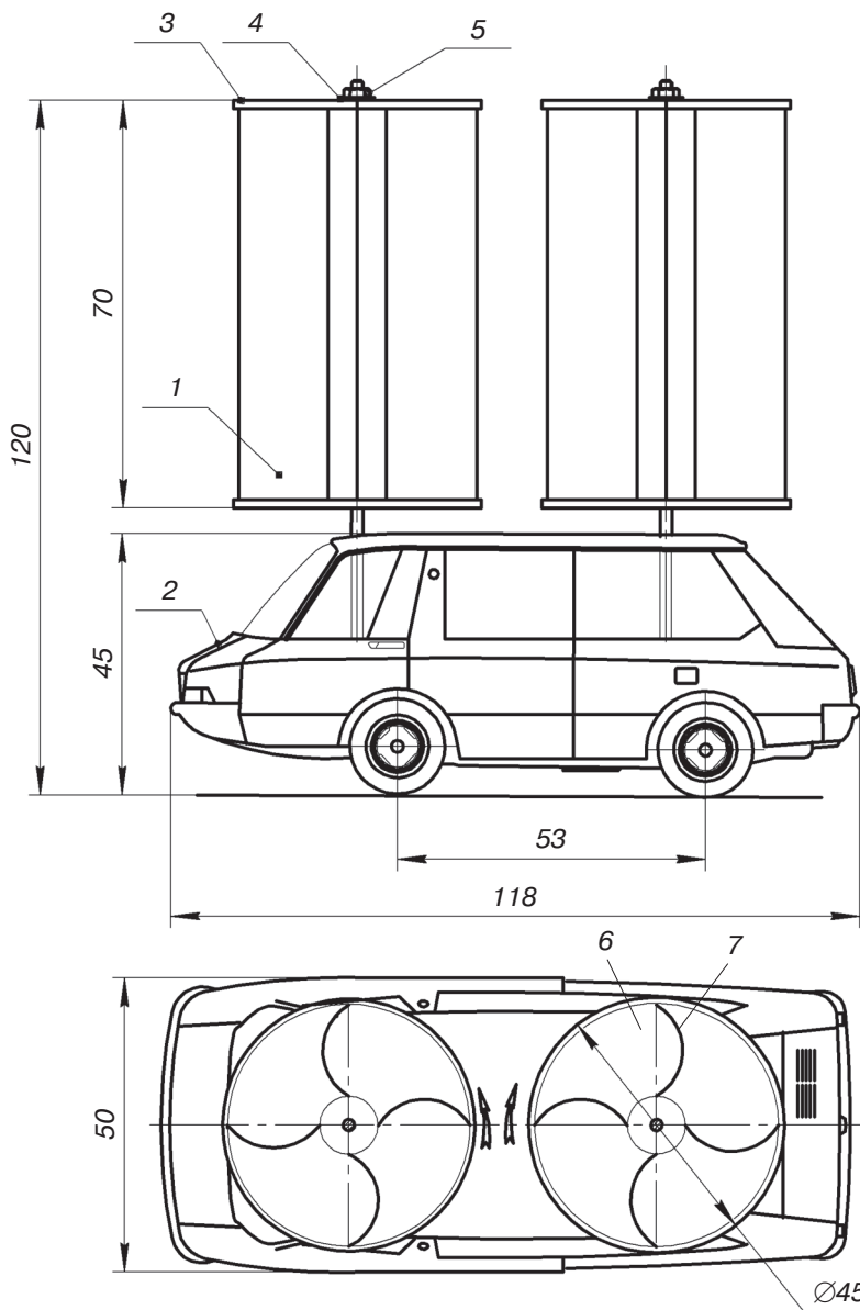
Рис. 2. Основные размеры модели.
