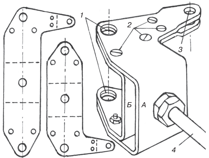
Рис. 4. Поворотная цапфа (левая):
