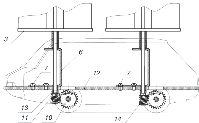
Рис. 4. Схема установки осей роторов.
