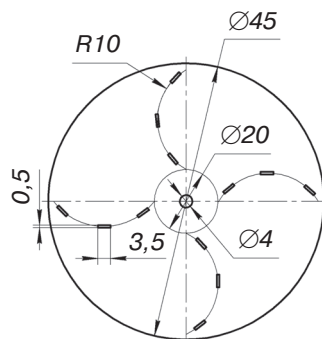
Рис. 6. Лопасть ротора.
