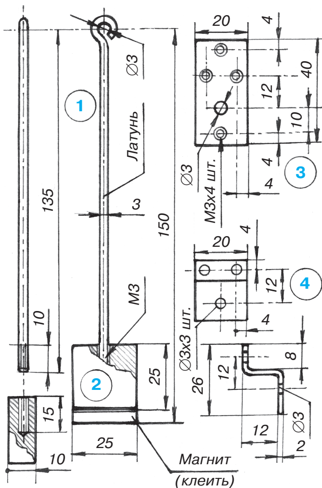
Рис. 4. Детали и размеры маятника: 1 — маятник; 2 — груз; 3 — крепежная пластина (сталь толщиной 3 — 4 мм); 4 — кронштейн.
