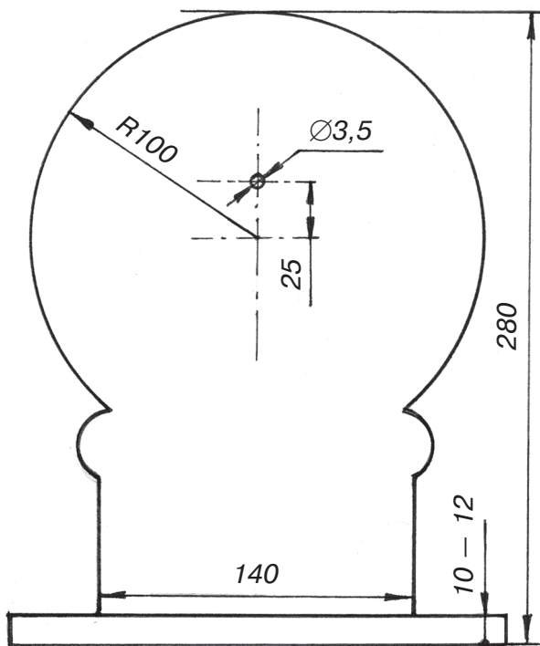
Рис. 3. Примерные размеры панели маятника.
