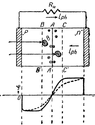
Рис. 16. Схема действия фотоэлемента с p — n -переходом.
