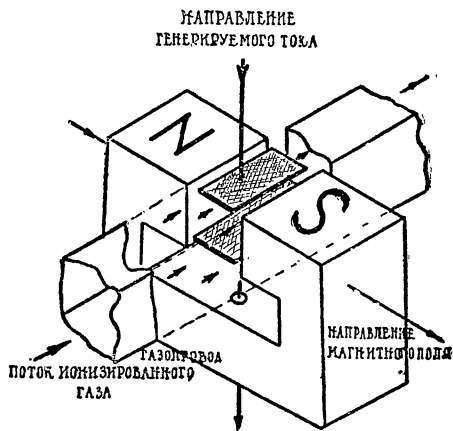
Рис. 6. Принцип магнитогиродинамического генератора.
