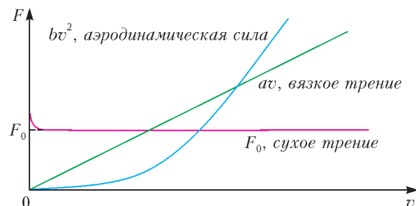
Рис.1. Зависимость сил сопротивления от скорости плуга
