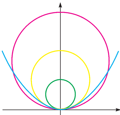
Рис.6. Большая окружность слишком велика, маленькая – слишком мала
