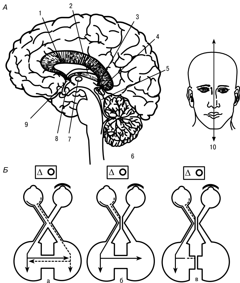
Рис. 14. Межполушарные связи:
