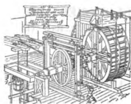
Рудоподъемная машина, построенная К. Фроловым в 1785 г.
