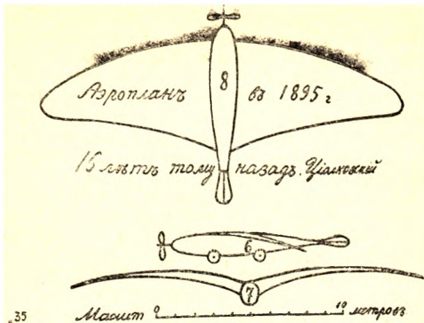
Собственноручная схема самолета Циолковского (1895) с обложки брошюры «Защита аэронаута» (1911).
