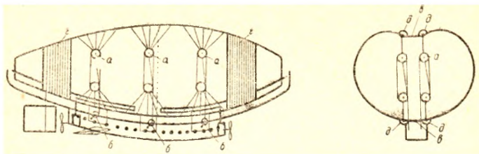
Схема цельнометаллического дирижабля Циолковского в продольном и поперечном разрезах.
