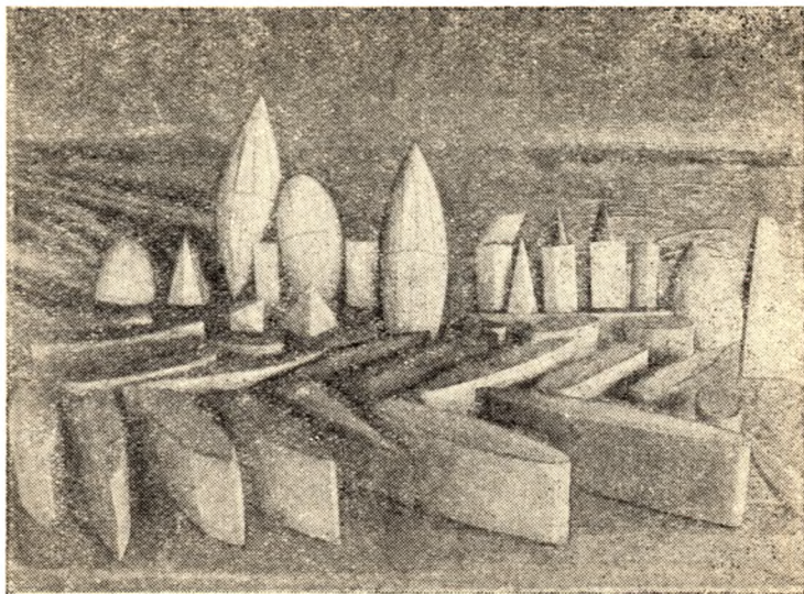
Модели (работы Циолковского), служившие при опытах по сопротивлению воздуха.
