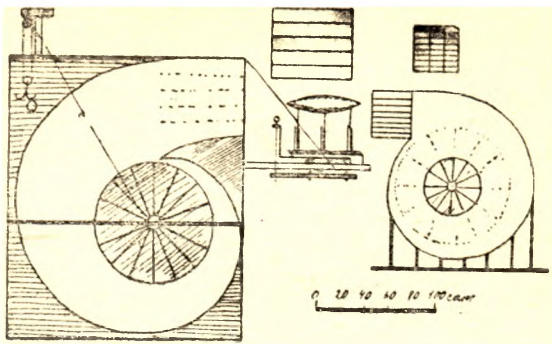
Факсимиле собственноручной схемы первой (1897) и второй (1900—1901) аэродинамической трубы Циолковского.
