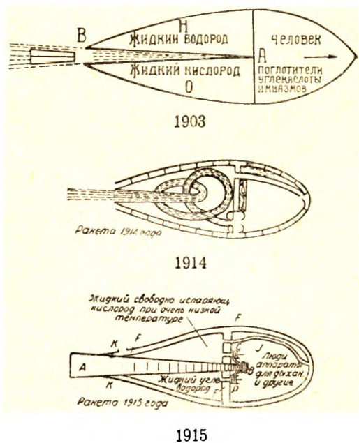
Схемы космических ракет Циолковского.
