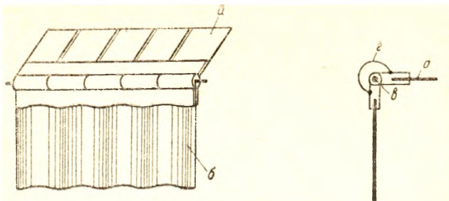
Шарнирное соединение гофрированных боковин с основанием оболочки.
