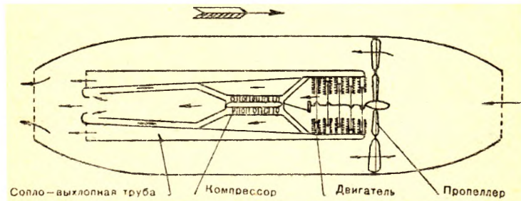
Схема полуреактивного стратоплана Циолковского.
