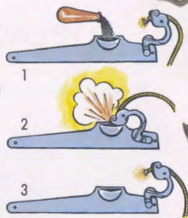
Этапы действия замка фитильного мушкета: 1. Засыпка пороха; 2. Удар и воспламенение; 3. Исходное положение
