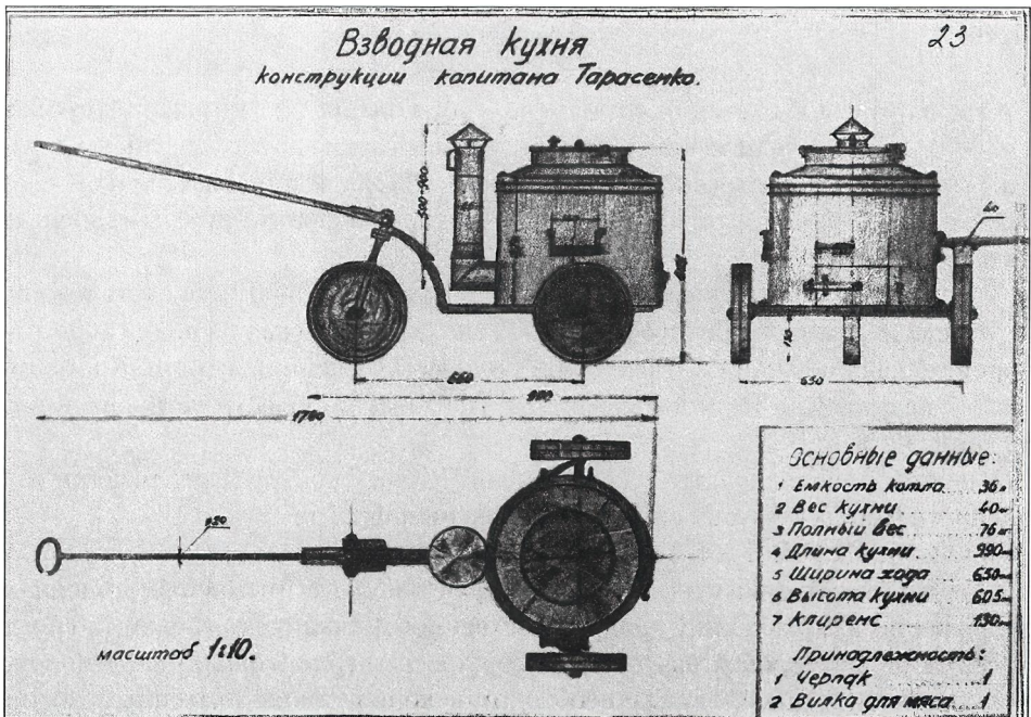
Схема армейской взводной кухни конструкции капитана Тарасенко
