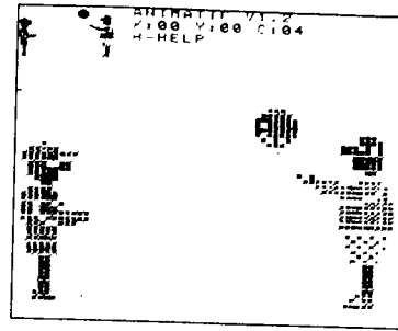
Рис. 6б. Графический редактор Animatic. Общий вид экрана в режиме создания и редактирования спрайтов
